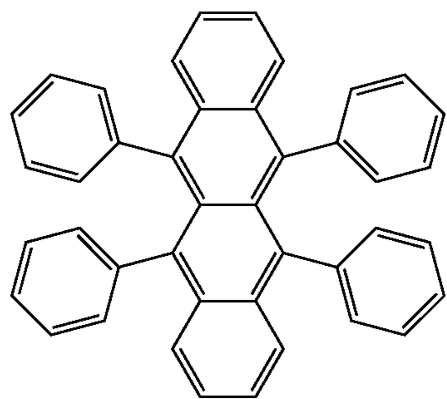
Rubrene
