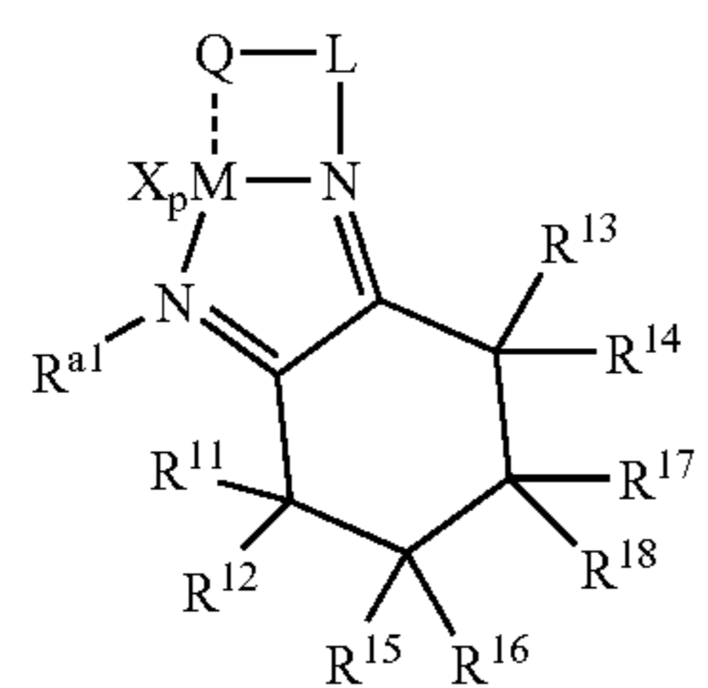
Structure 18e
