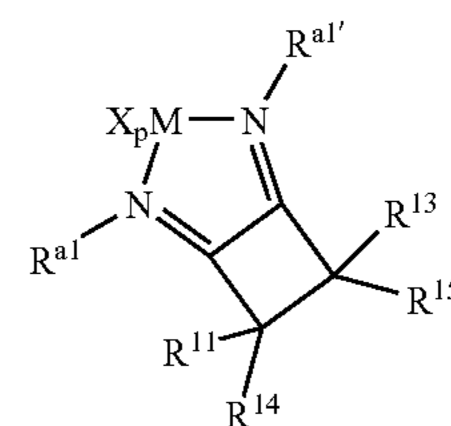
Structure 3e
