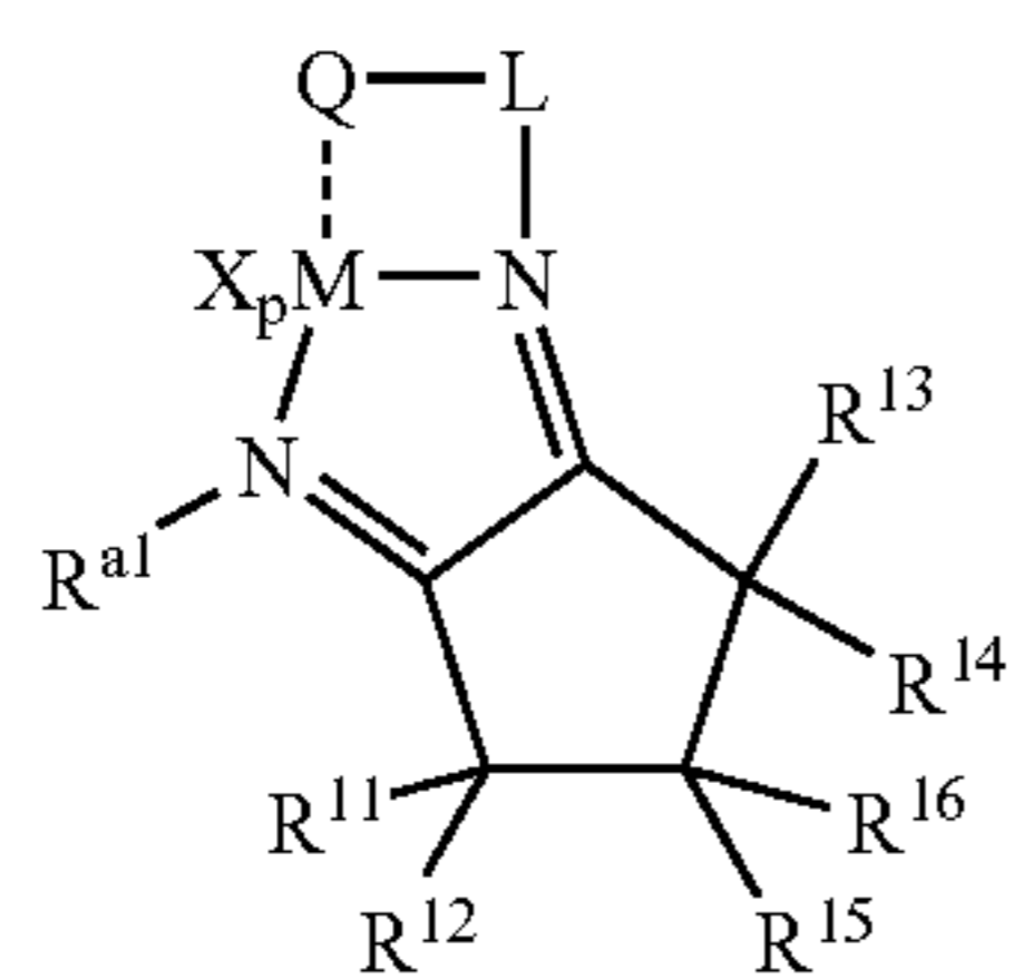
Structure 17e
