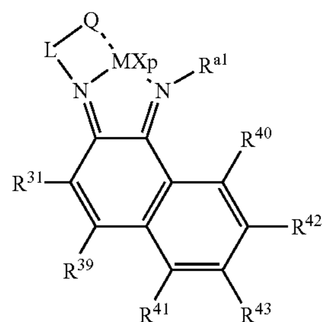
Structure 23e
