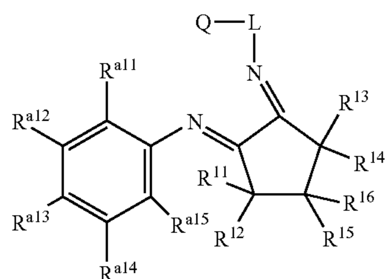
Structure 30f
