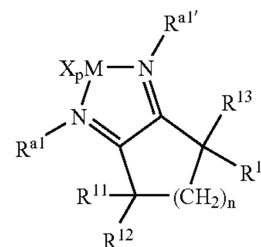
Structure 2e
