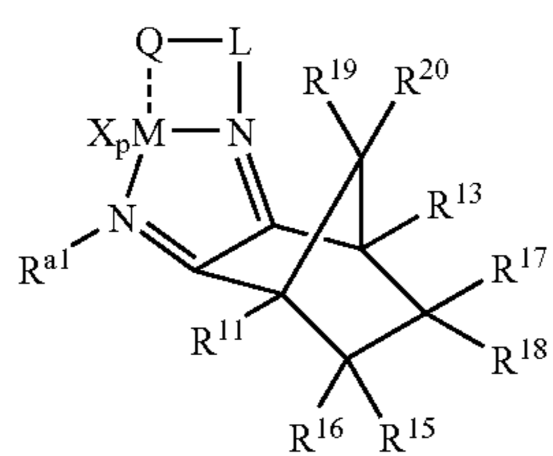
Structure 19e
