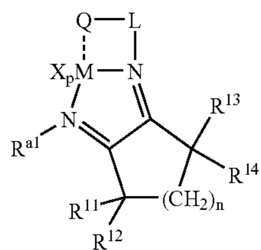
Structure 15e
