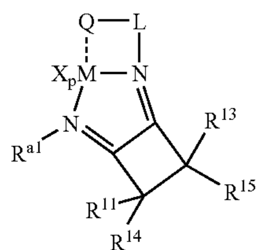
Structure 16e
