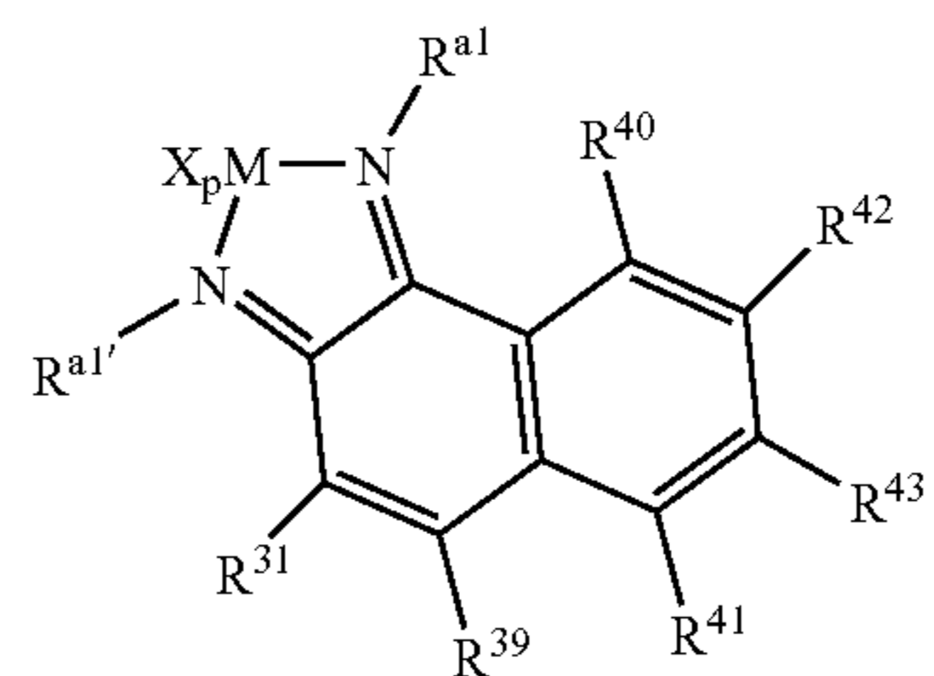
Structure 10e
