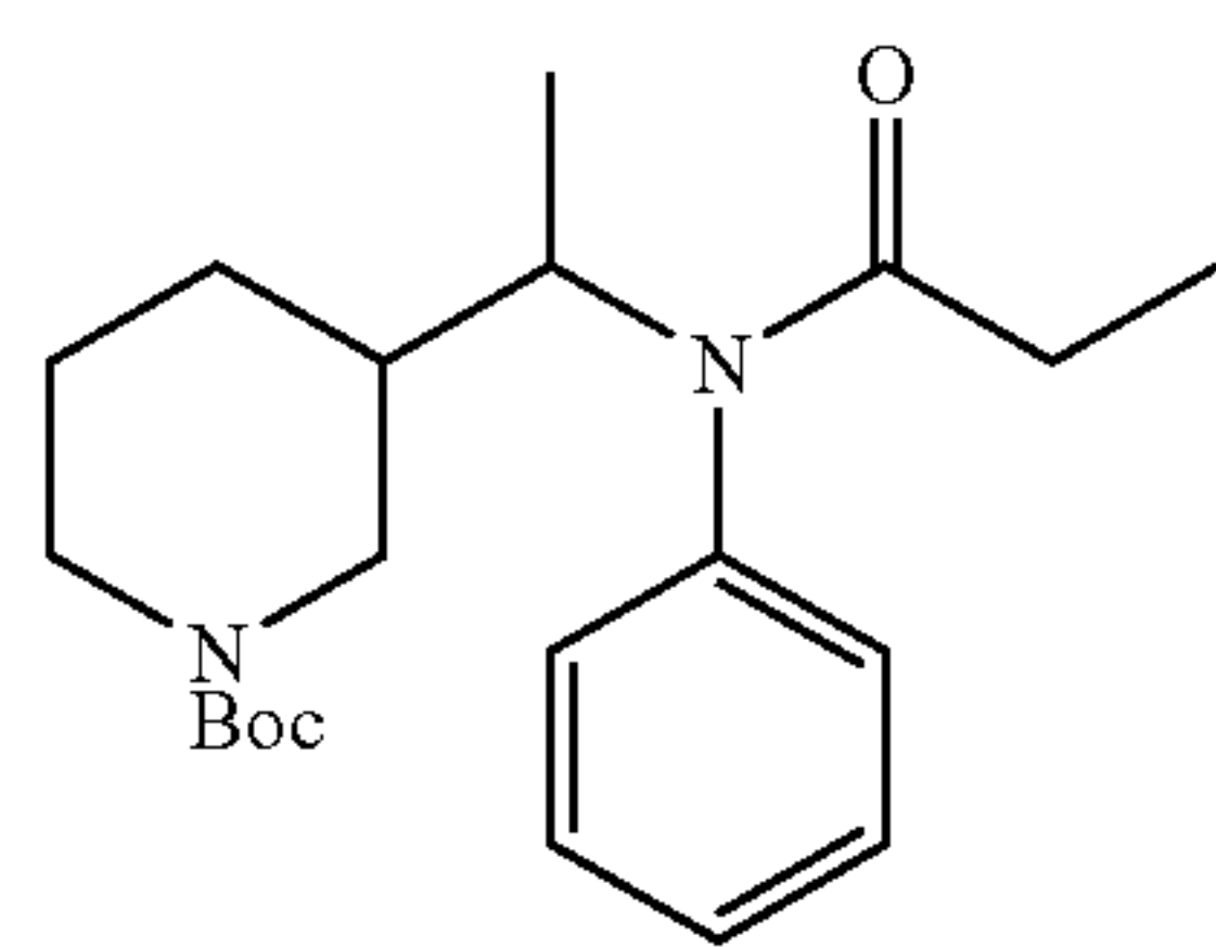
191 single enantiomer
