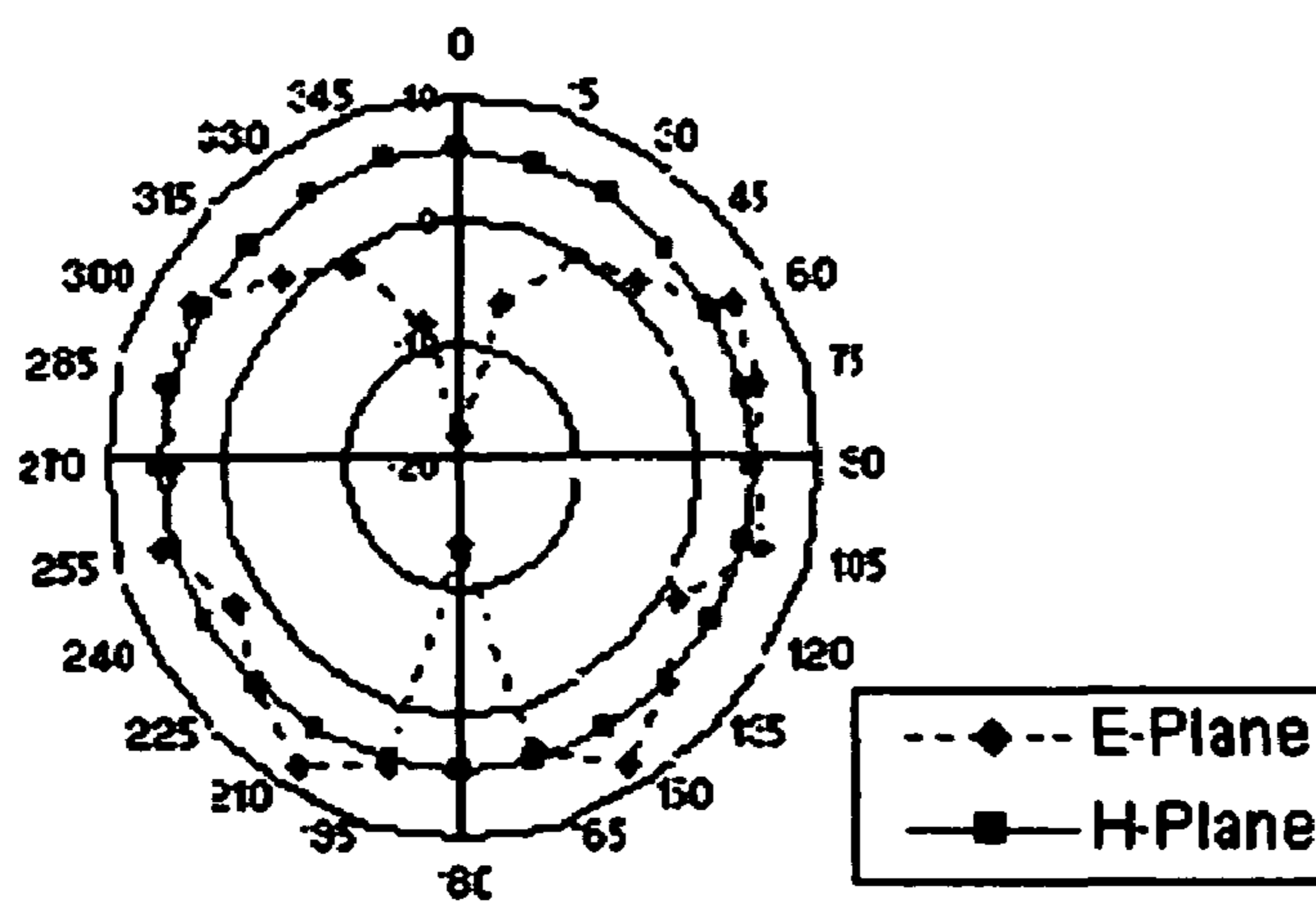
FIG. 3E
