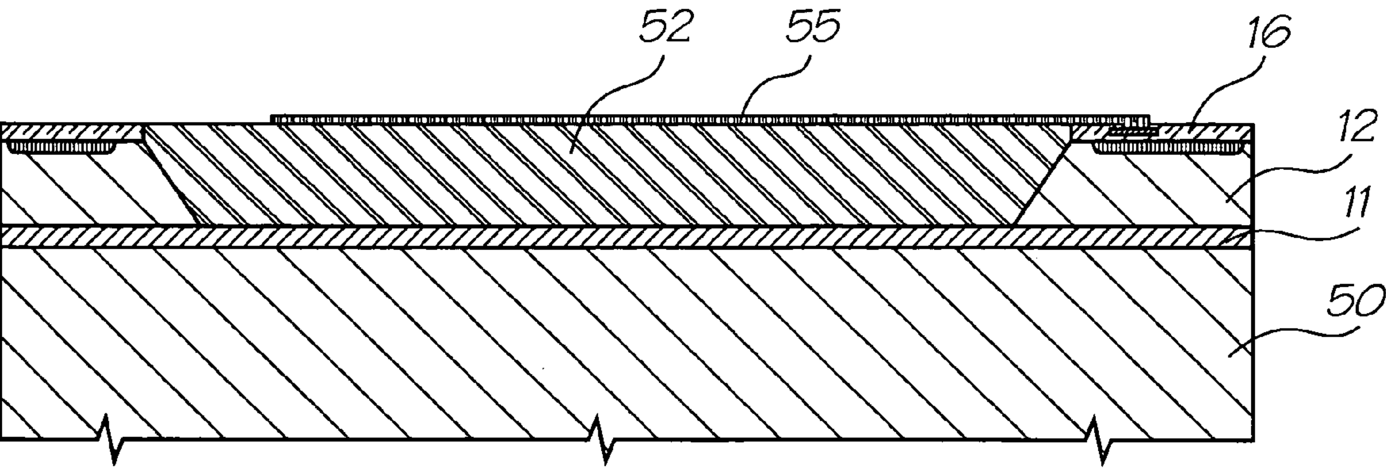
FIG. 10
