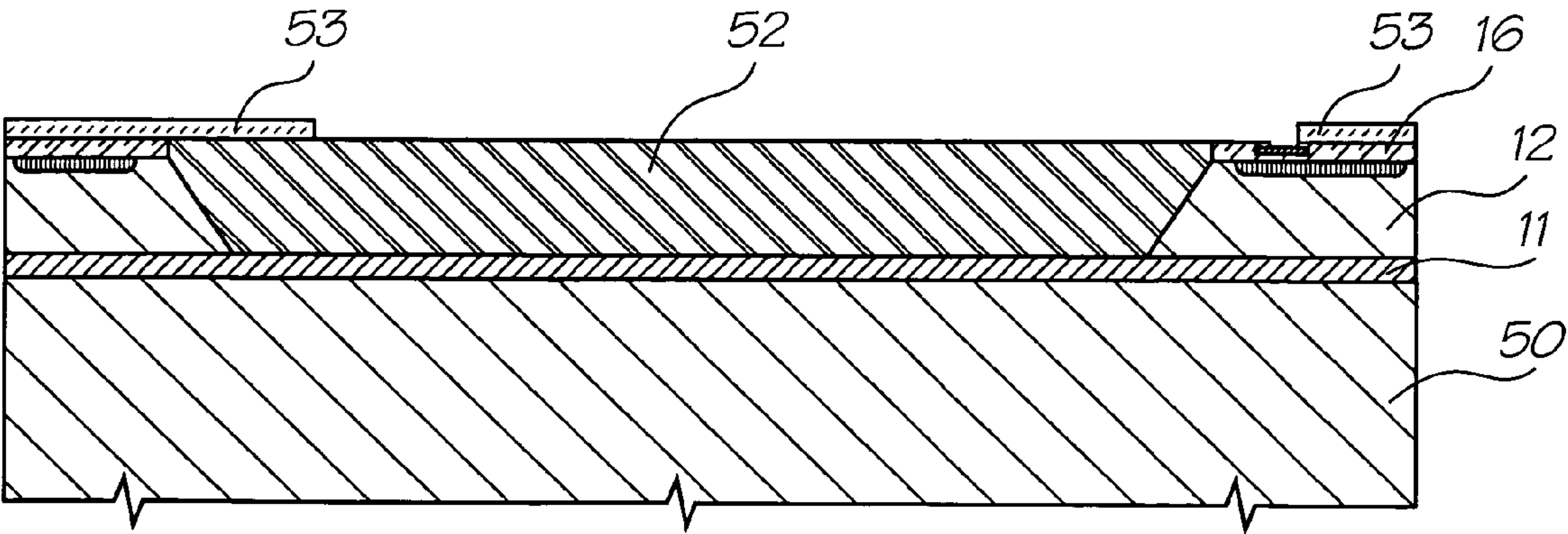
FIG. 9
