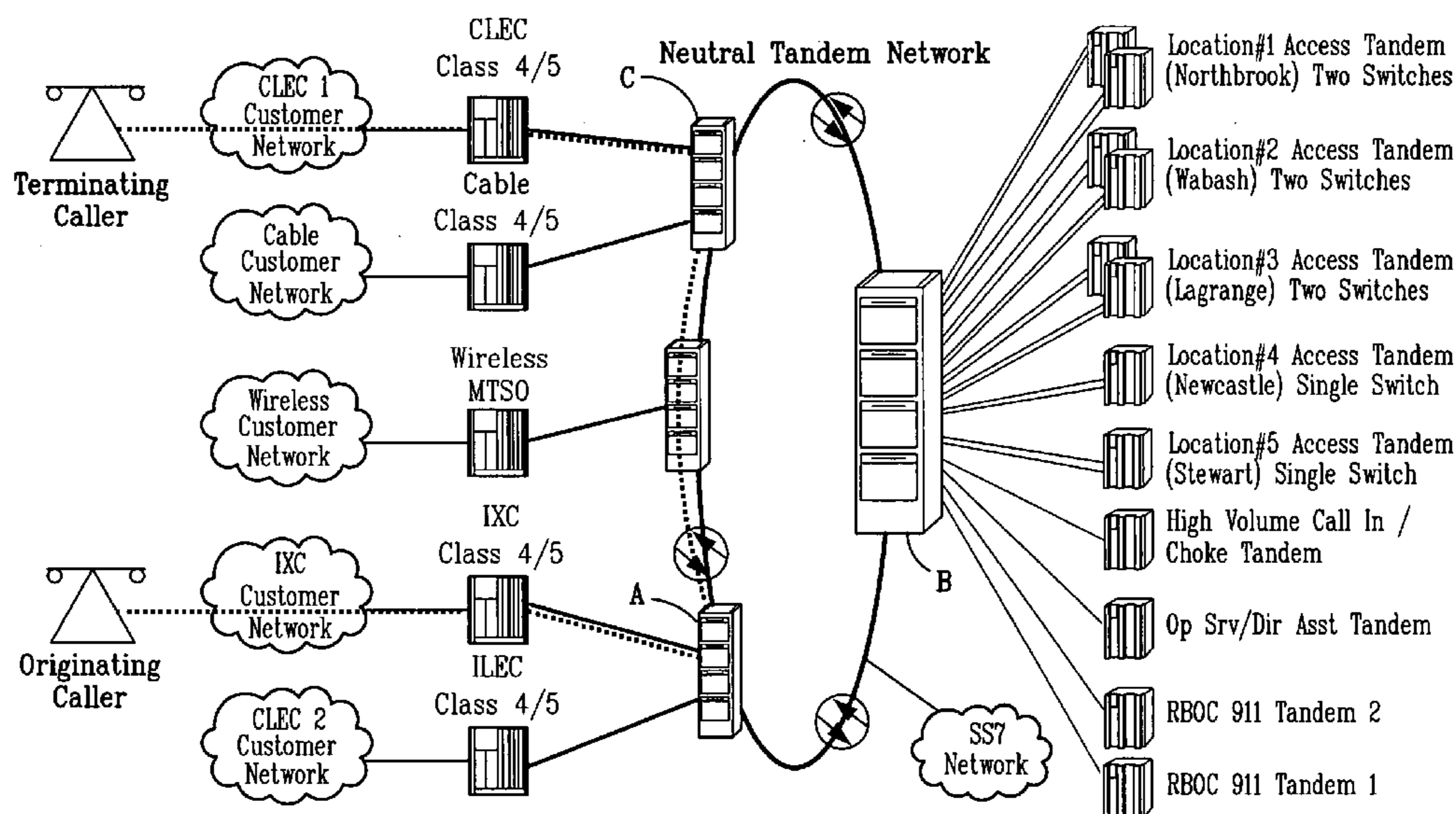
Ameritech LATA 357 Tandem Trunking Requirements
