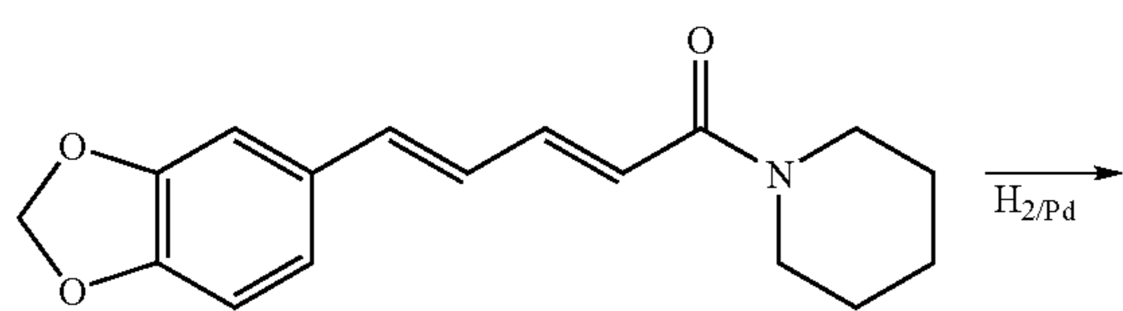
Piperine (1)
