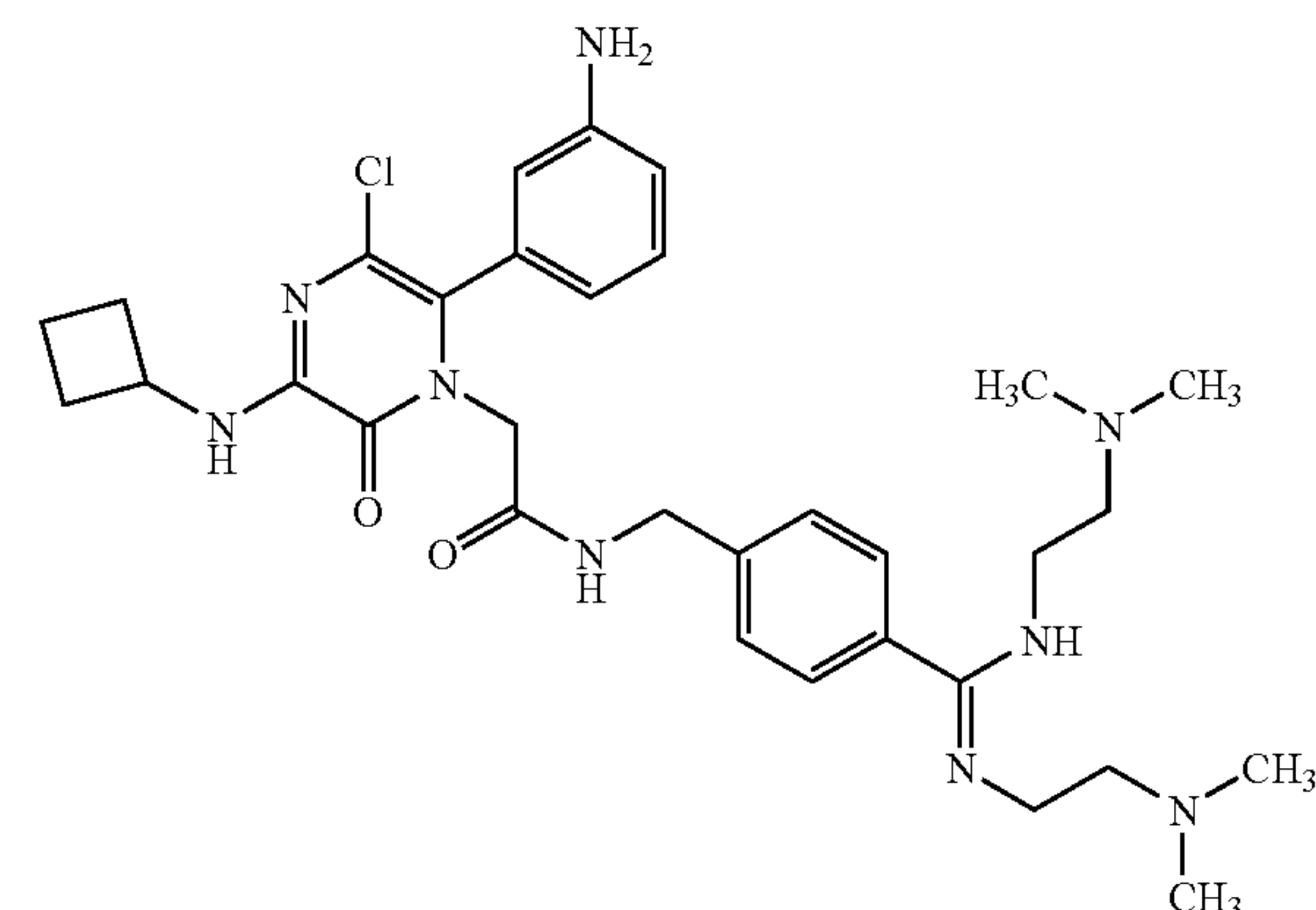
Example 165
