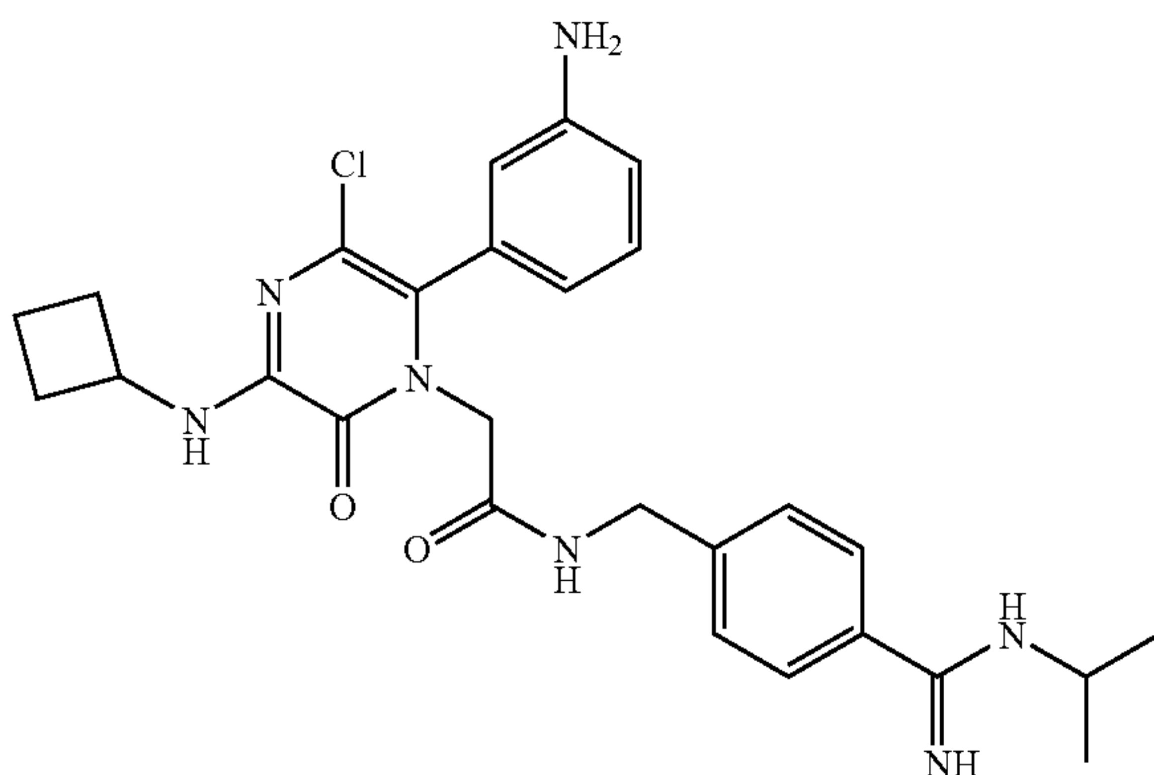
Example 161
