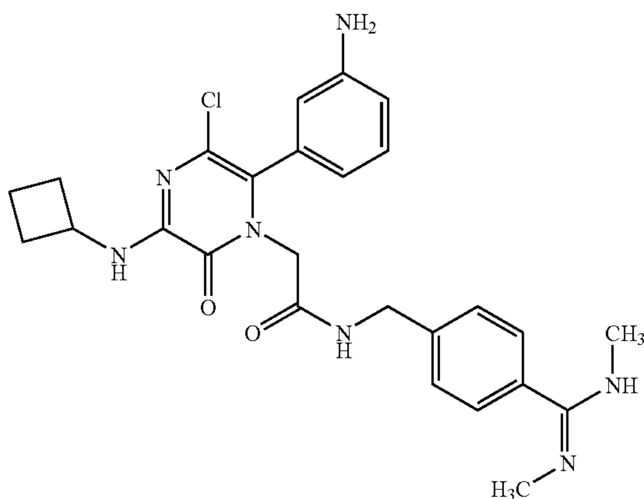
Example 162
