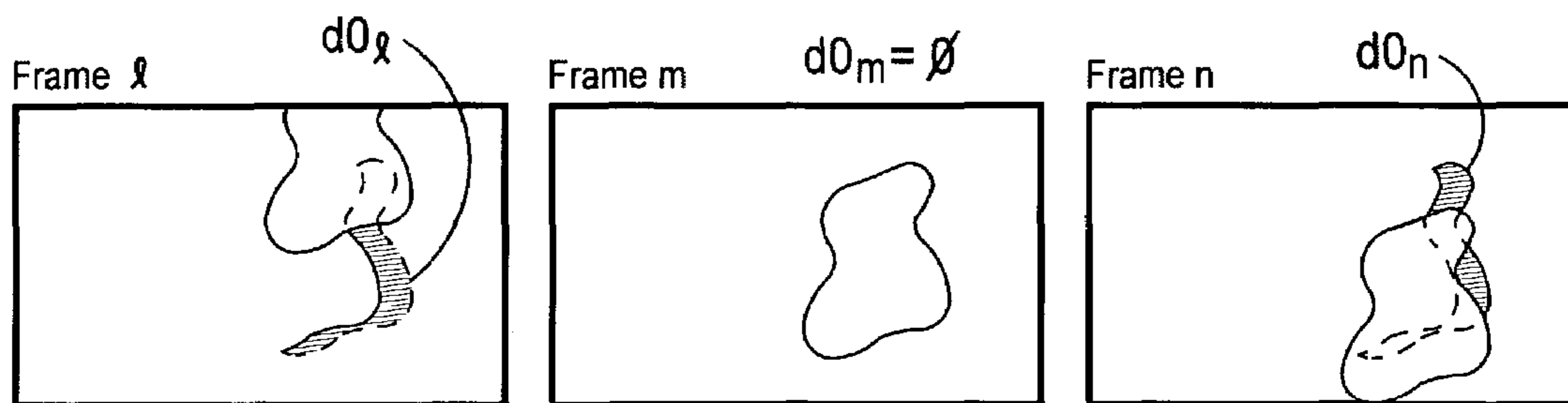
dOm = \emptyset Optimal Area = \cup_i (dO_i) FIG. 9
