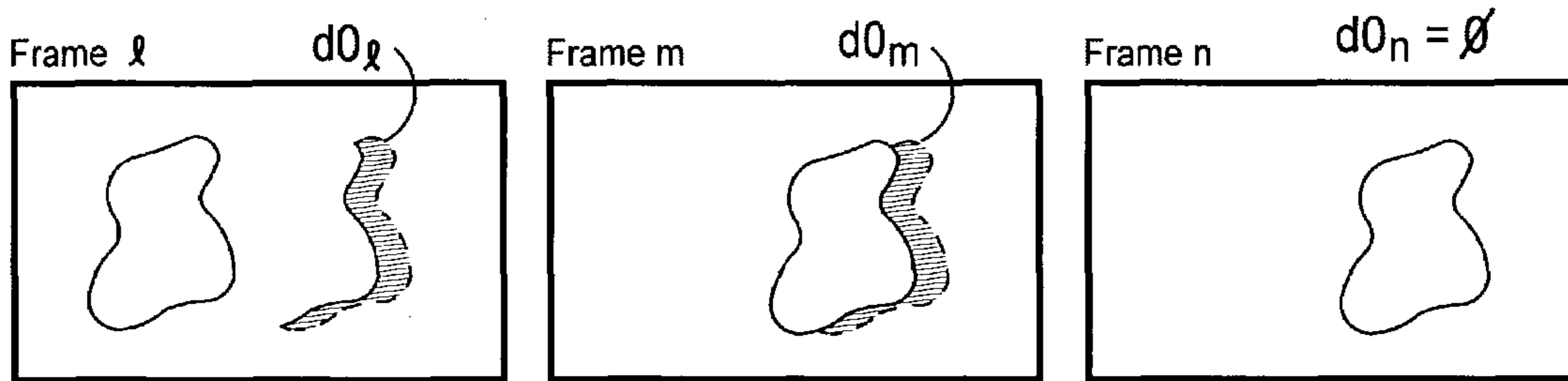
Optimal Area = \max \{ \|dO_i\|_{\mathbb{R}^2} \}_i FIG. 8
