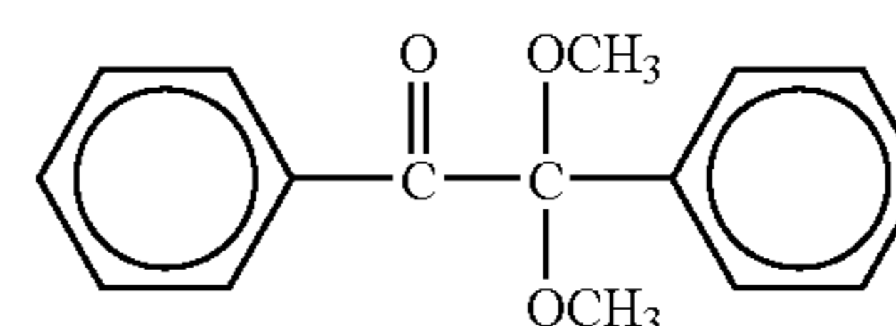
Irgacure 651:
