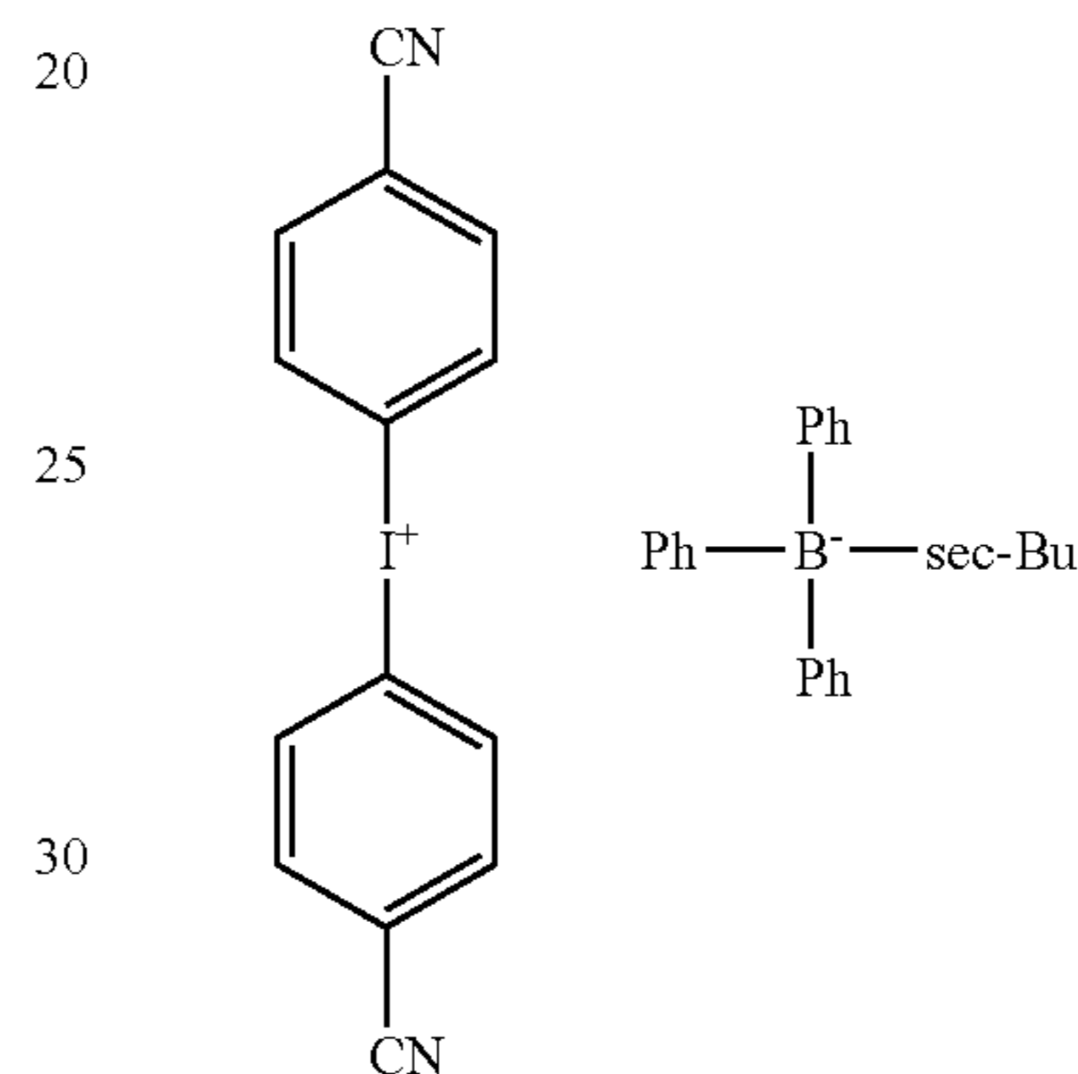
I-3:
