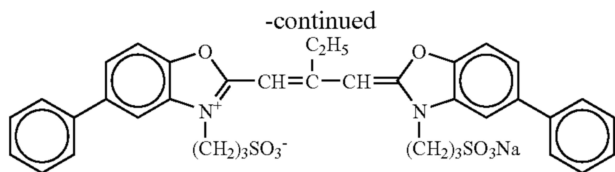
D-1
