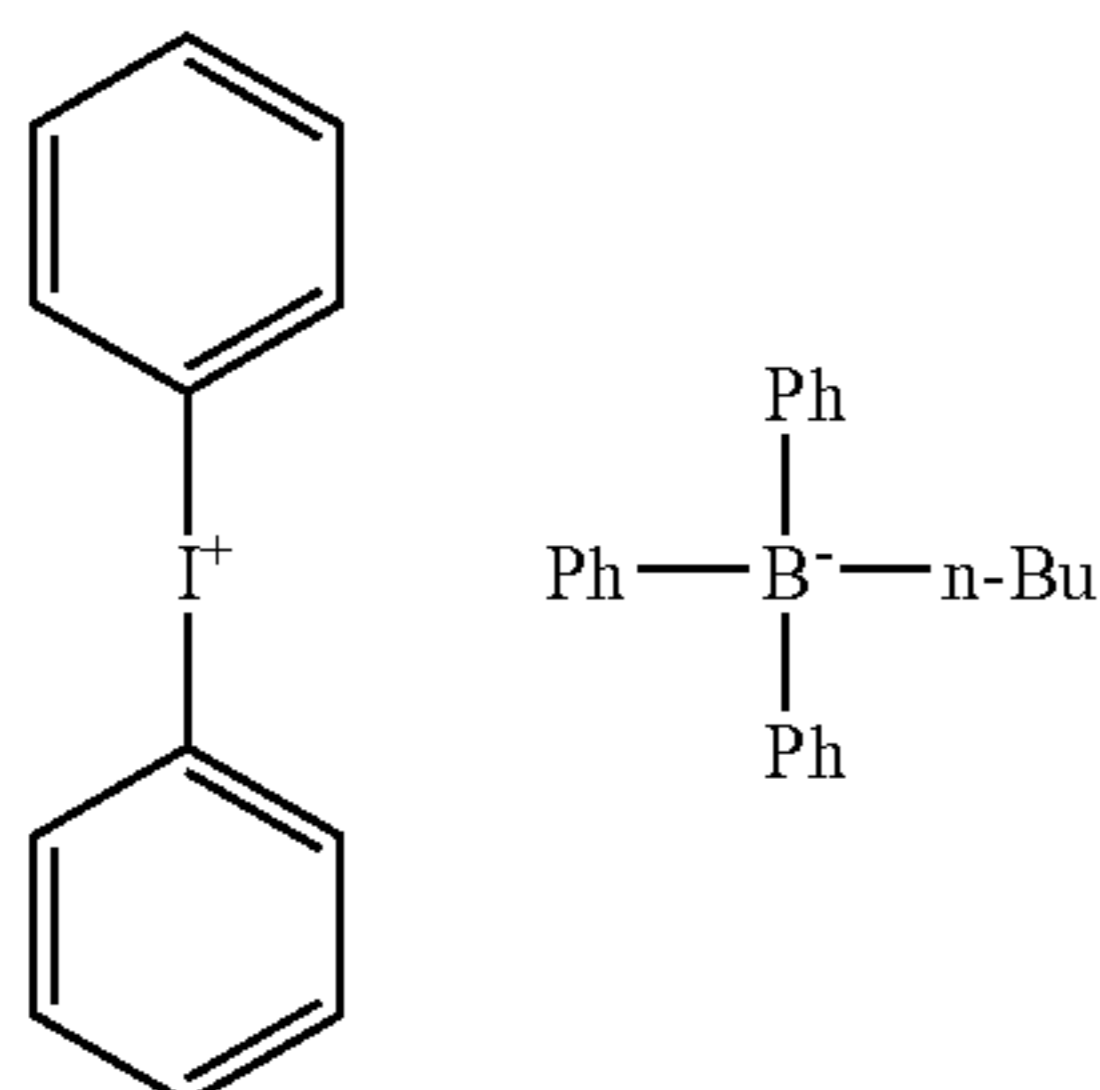
I-1:
