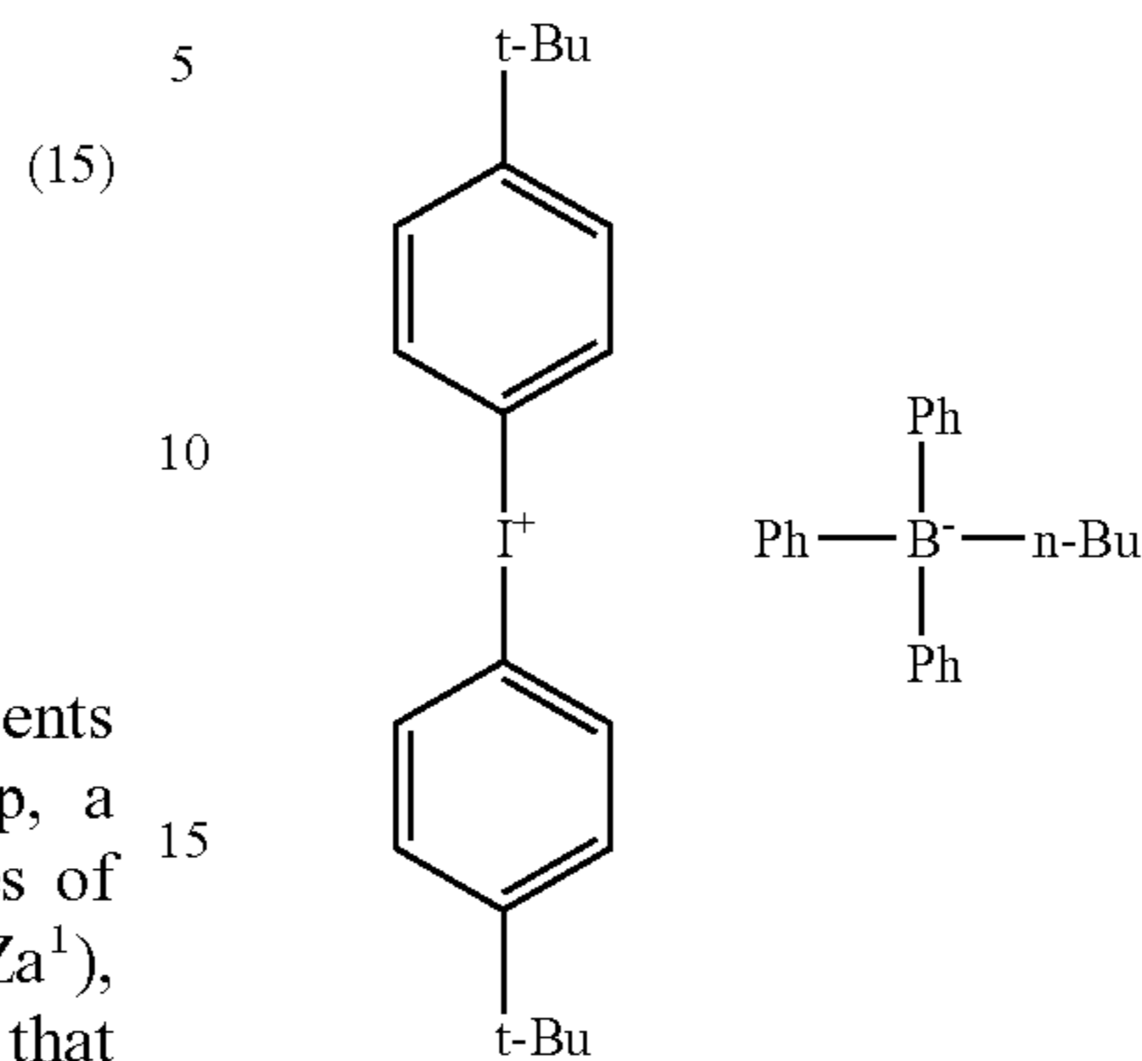
I-3:
