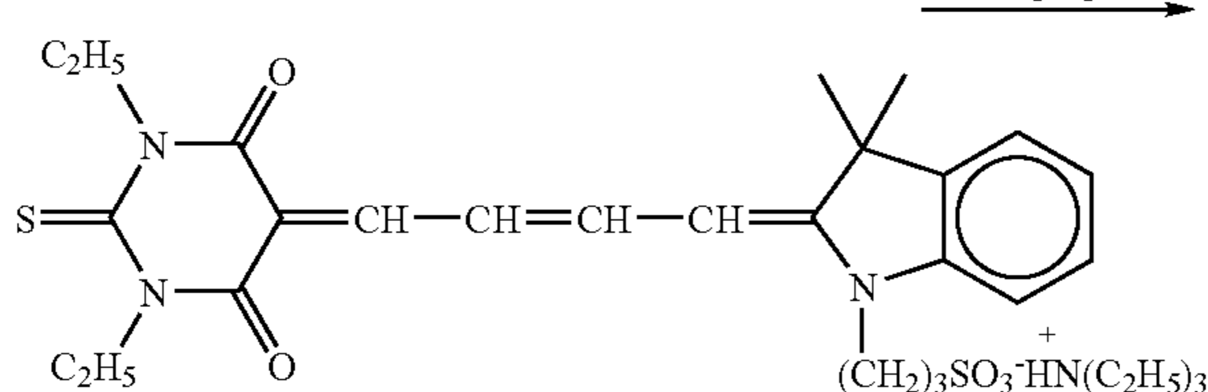
D-42
