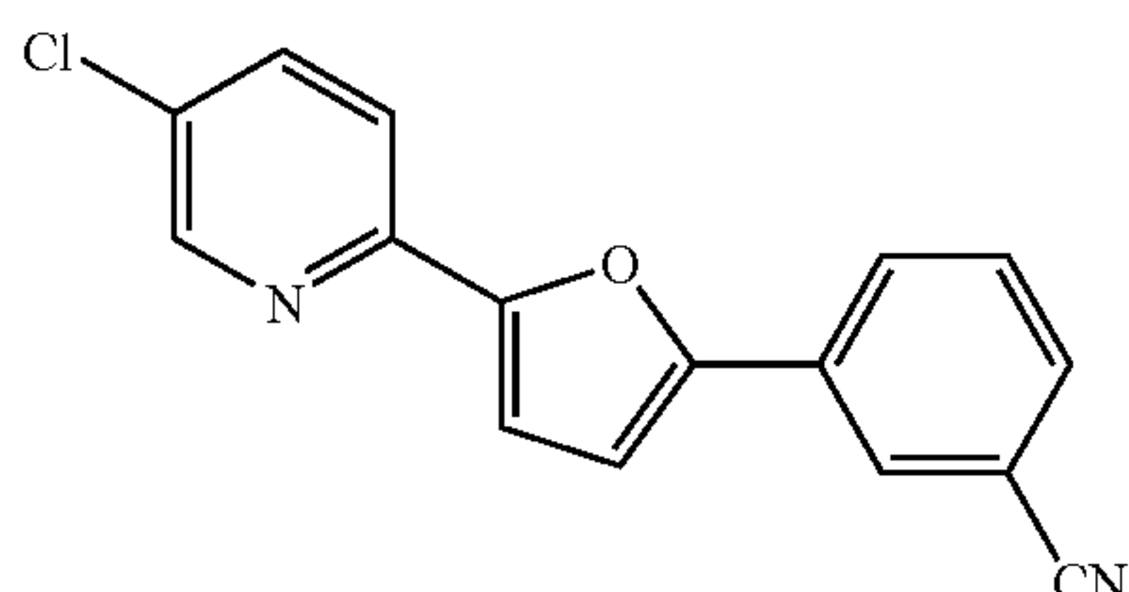
3-(5-(5-chloro-2-pyridyl)-2-furyl)-benzonitrile
