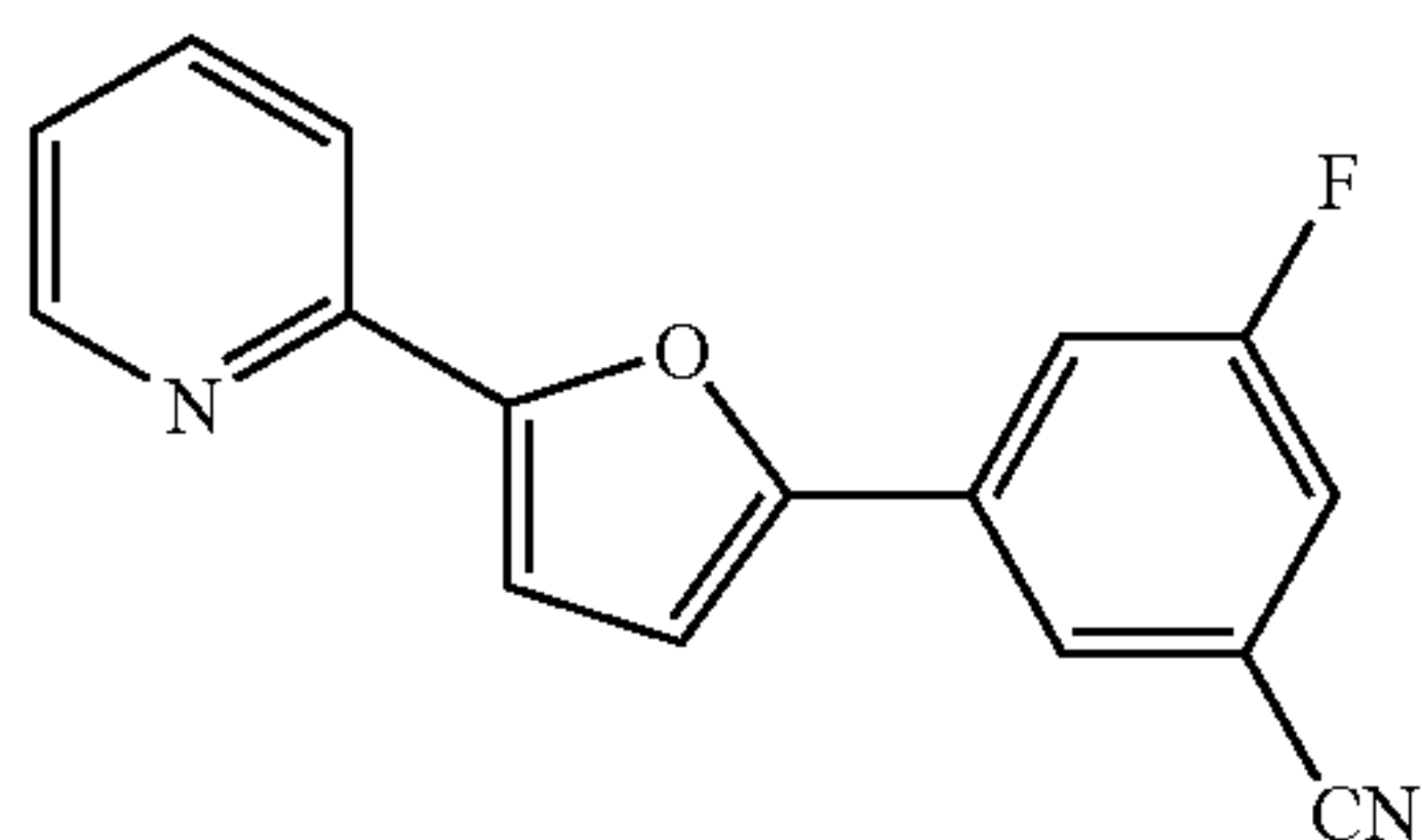
3-Fluoro-5-(5-(2-pyridyl)-2-furyl)-benzonitrile
