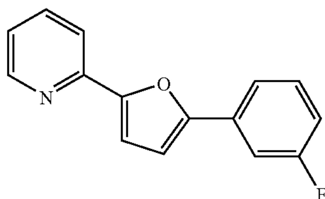
3-(5-(2-pyridyl)-2-furyl)-benzonitrile
