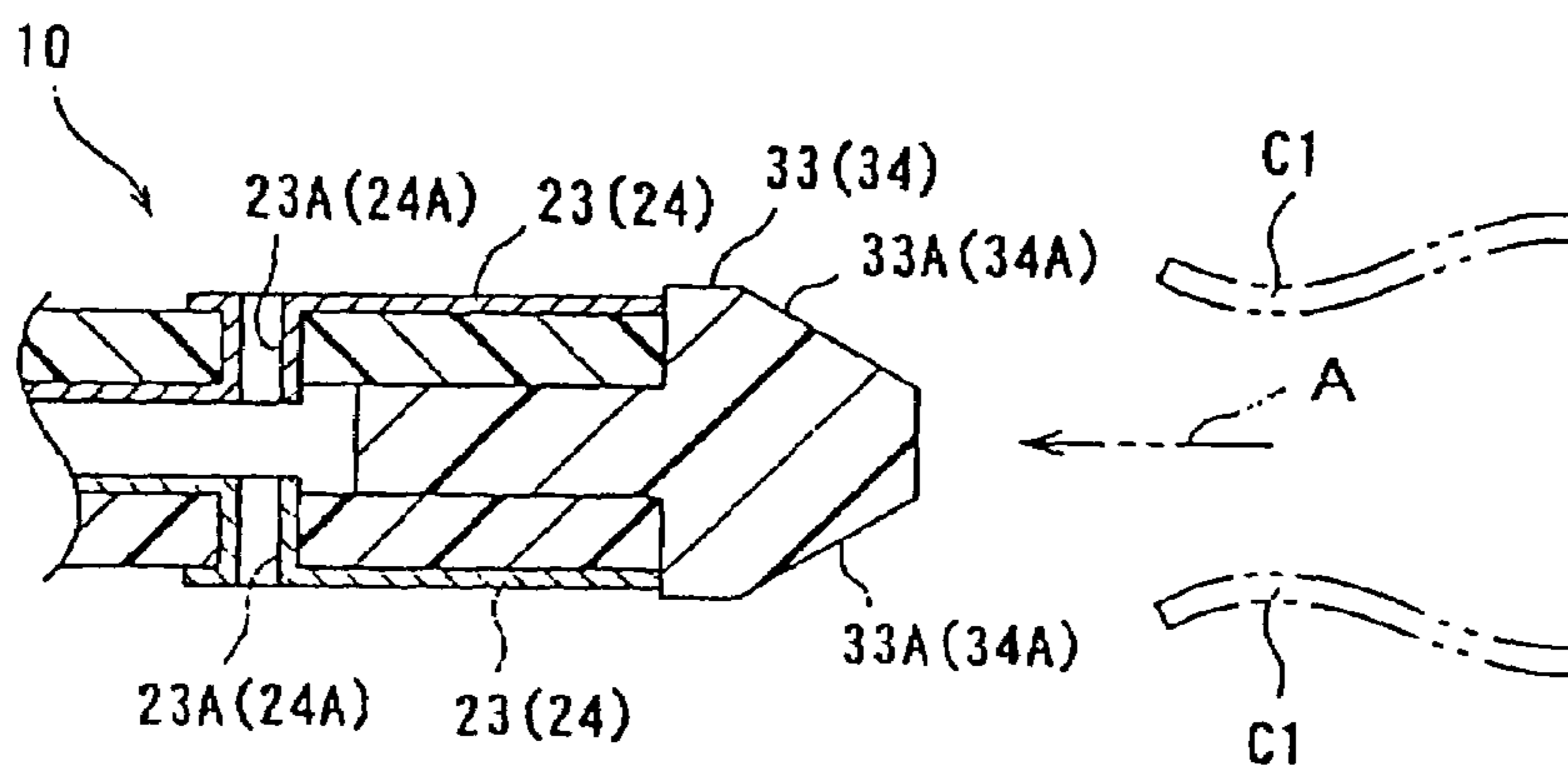
FIG. 3(B)
