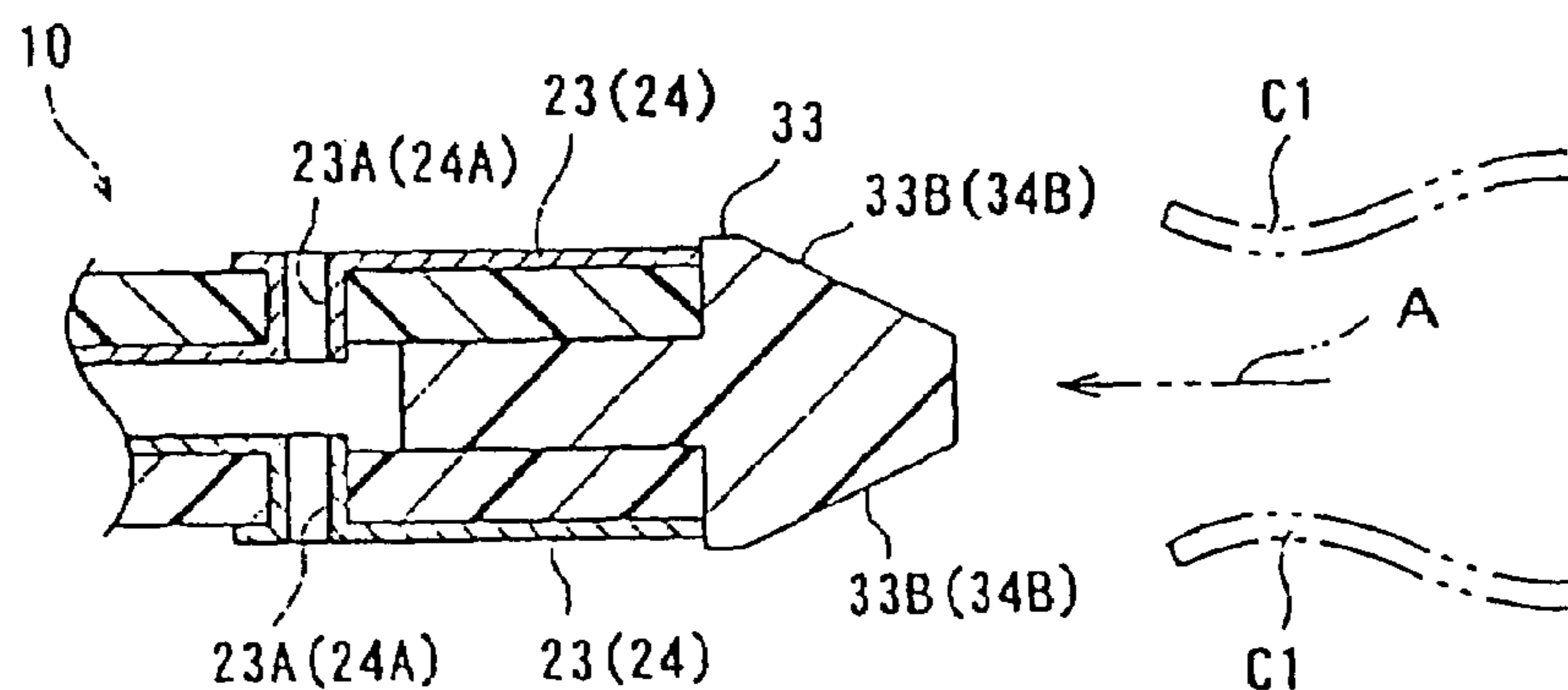
FIG. 3(C)
