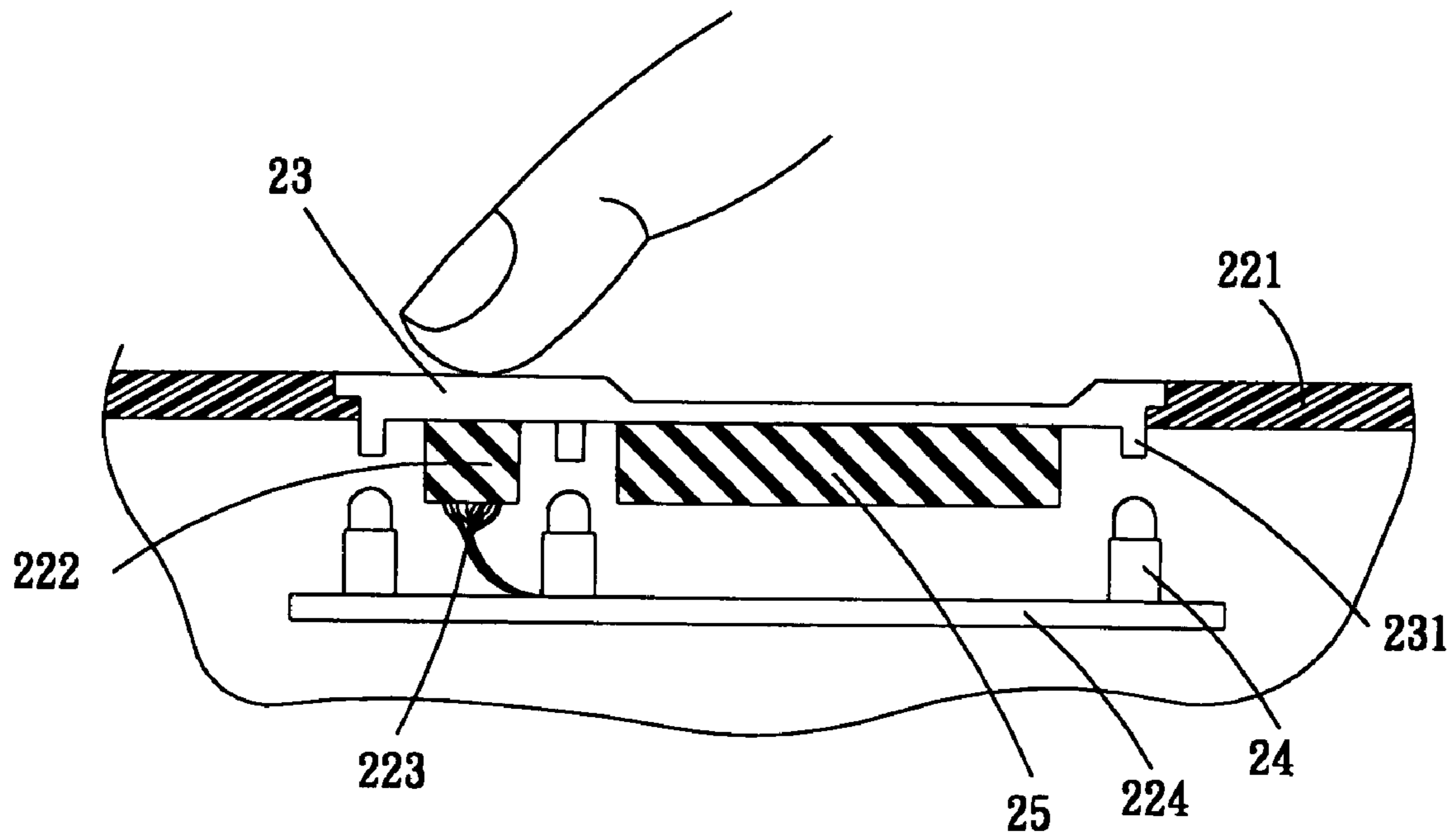
FIG. 5A
