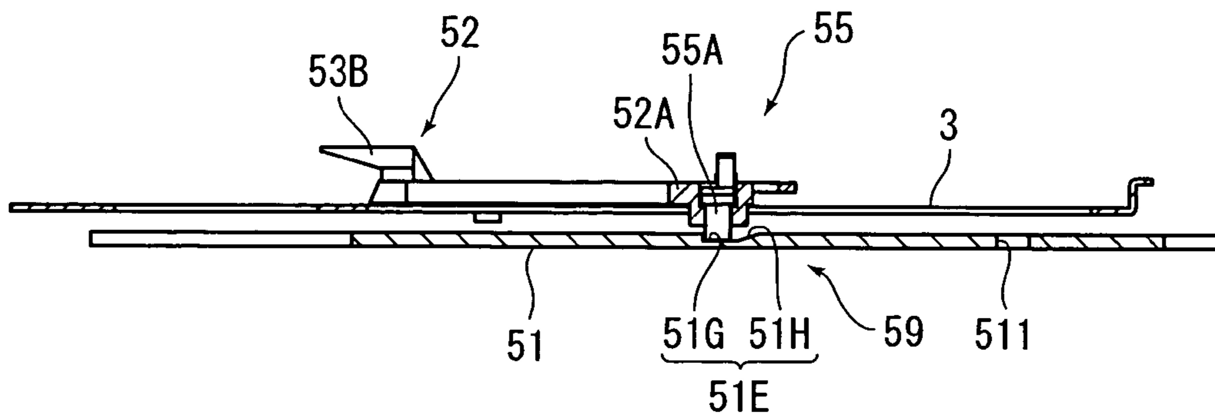
FIG. 5A
