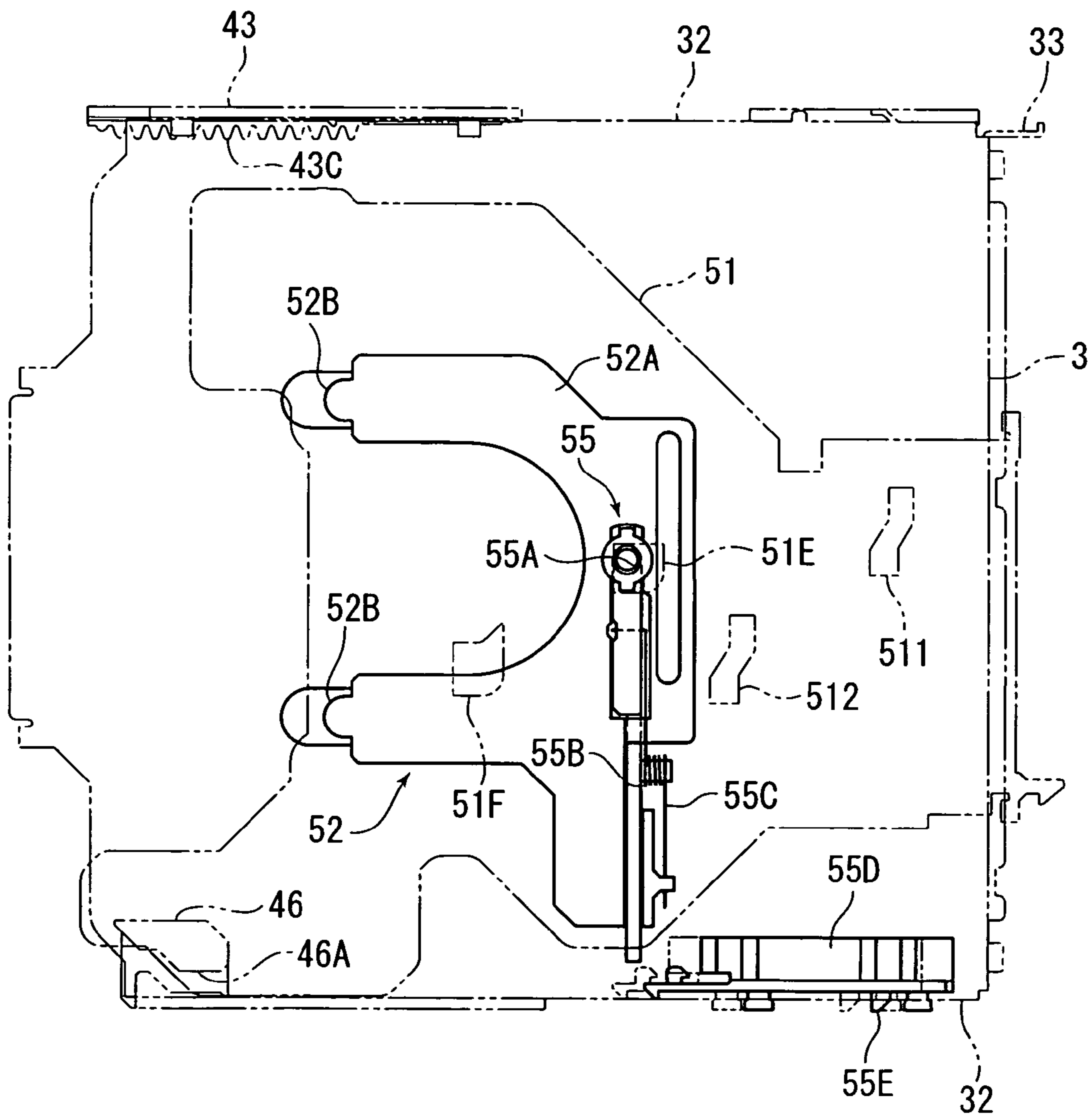
FIG. 5B
