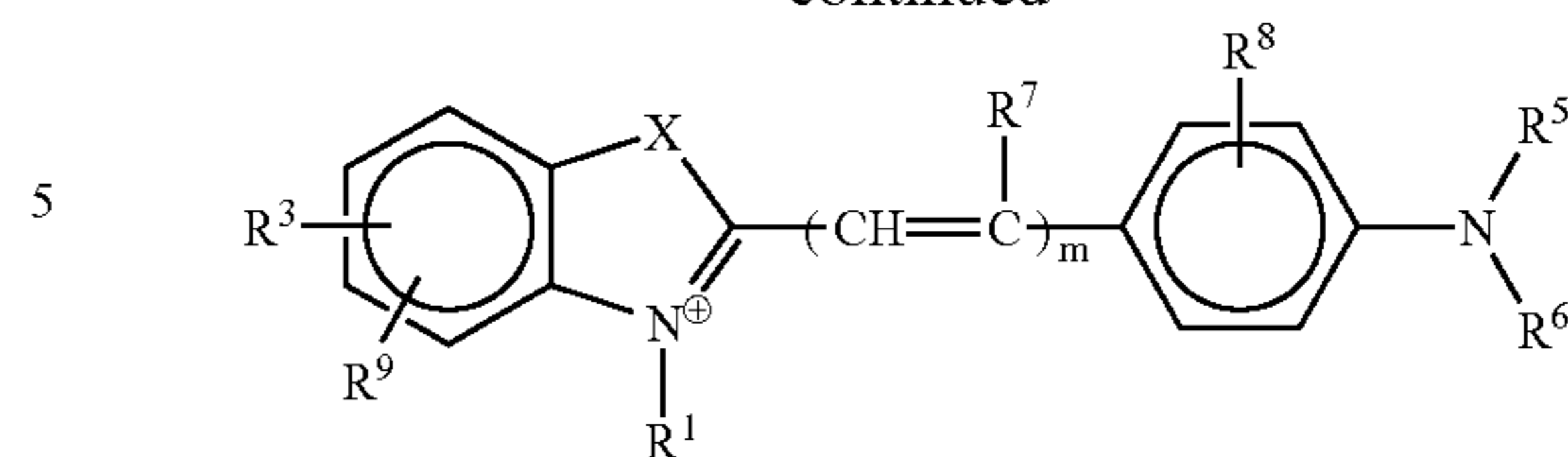
styryl
