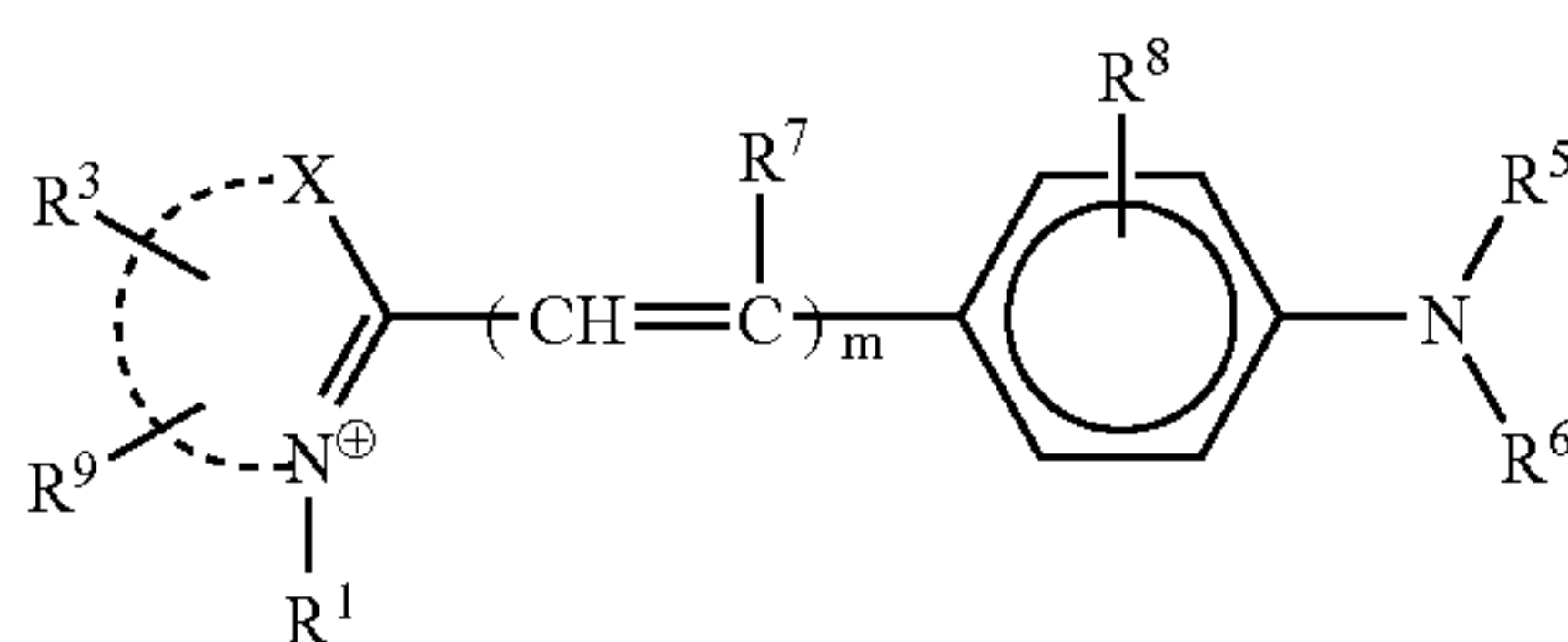
styryl
