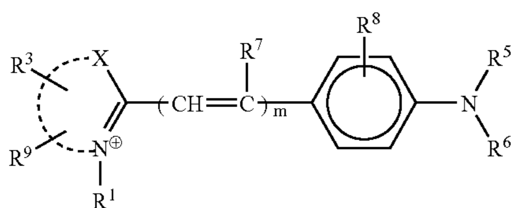
styryl
