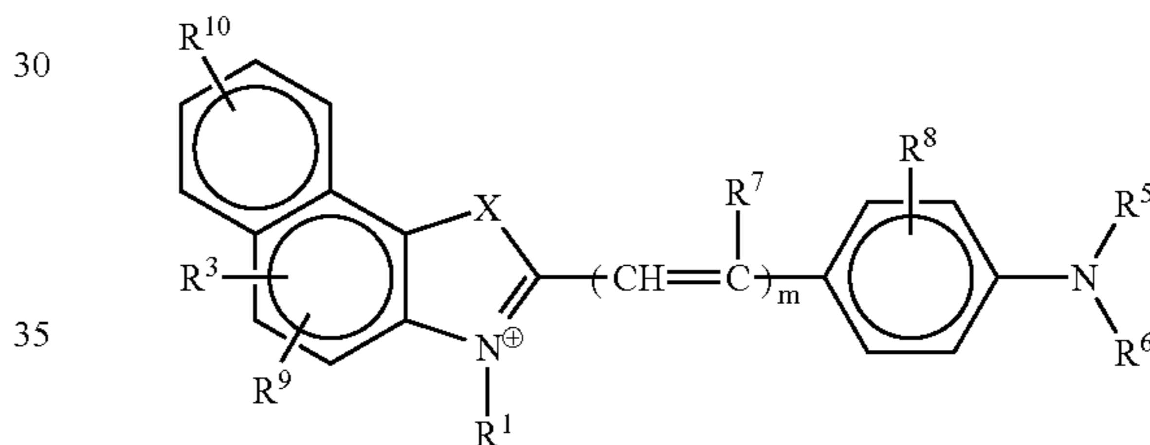
styryl
