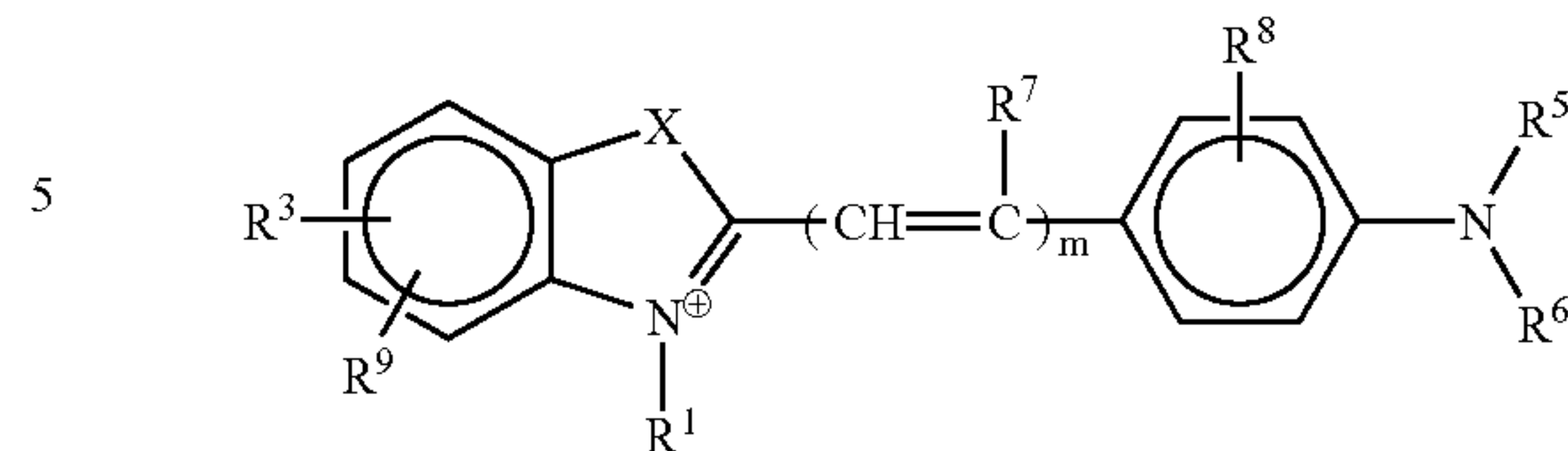
styryl
