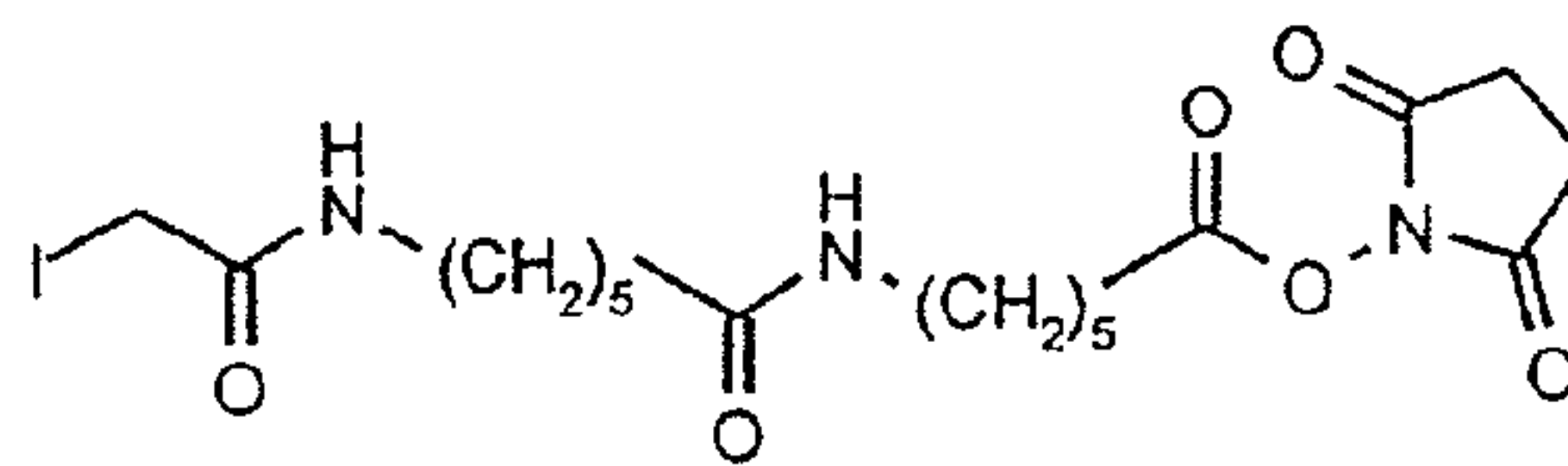
Succinimidyl 6-[6-(((iodoacetyl)amino)-hexanoyl)amino]hexanoate
