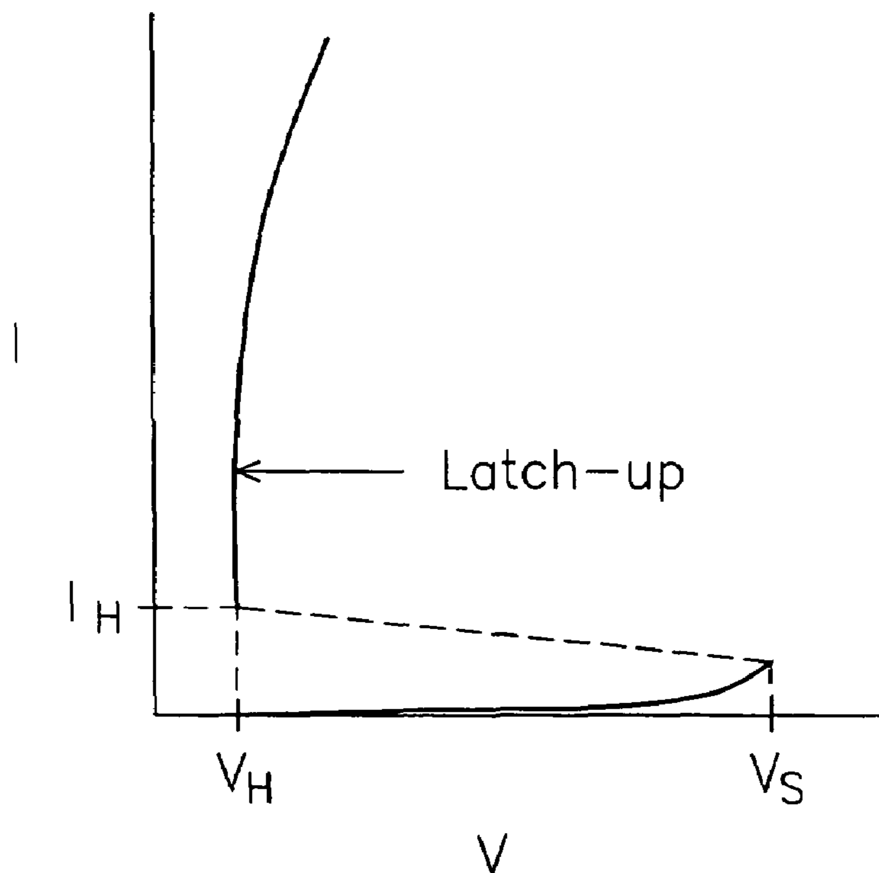
FIG. 3B(PRIOR ART)
