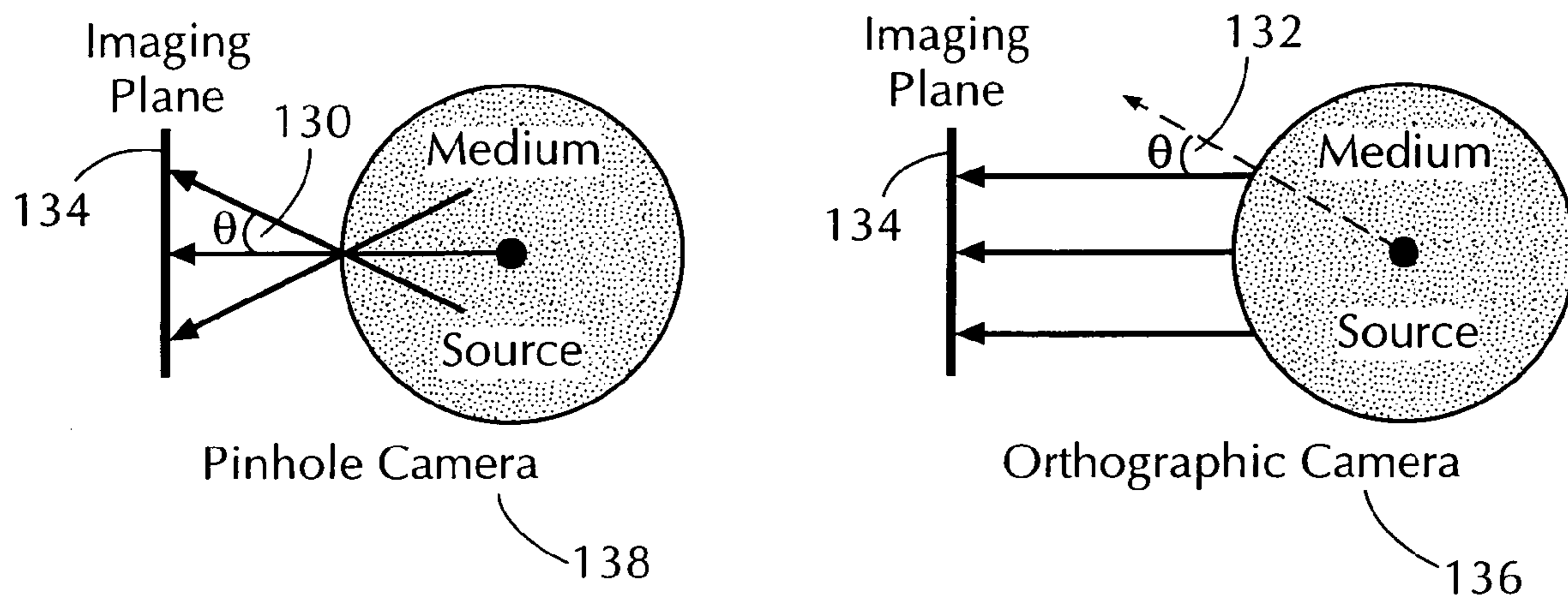
FIG. 13
