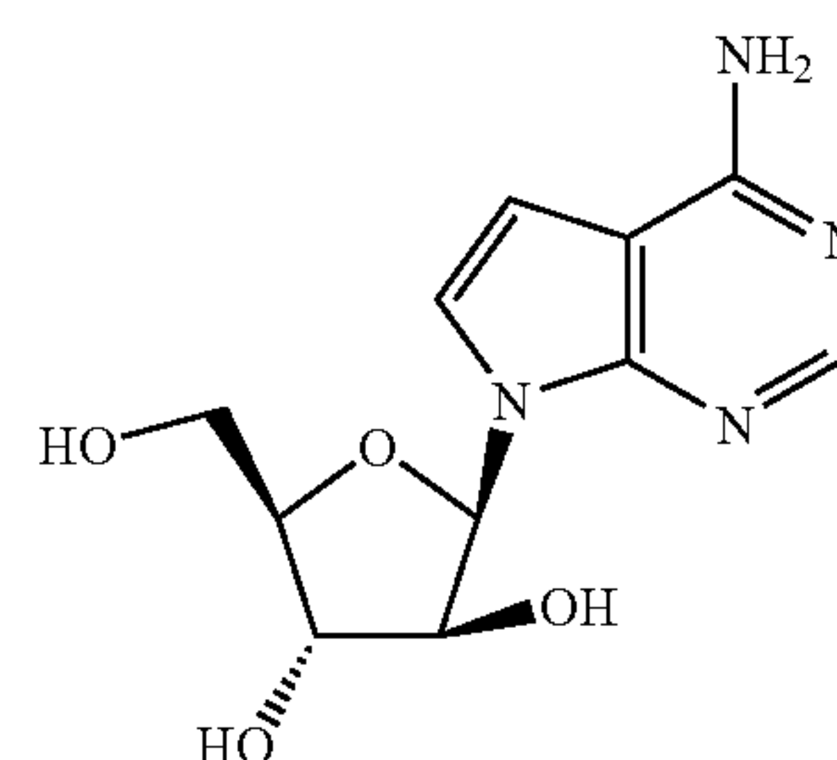
4-Amino-7-(β-D-arabinofuranosyl)-7H-pyrrolo[2,3- d]pyrimidine
