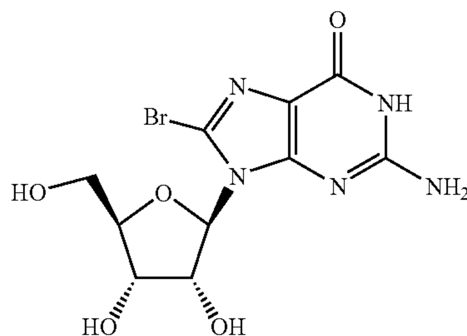
8-Bromoguanosine
