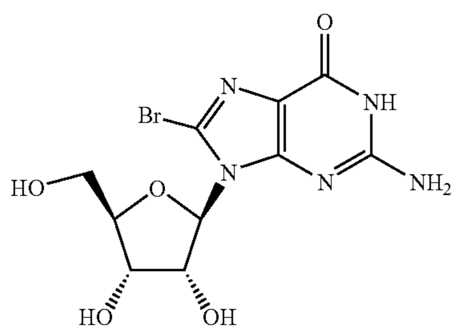
8-Bromoguanosine
