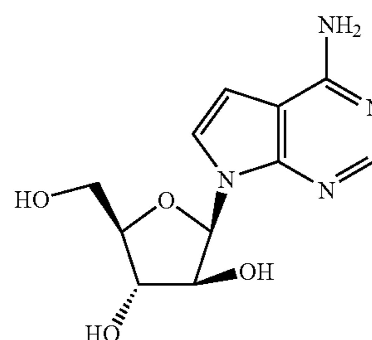
4-Amino-7-(β-D-arabinofuranosyl)-7H-pyrrolo[2,3-d]pyrimidine
