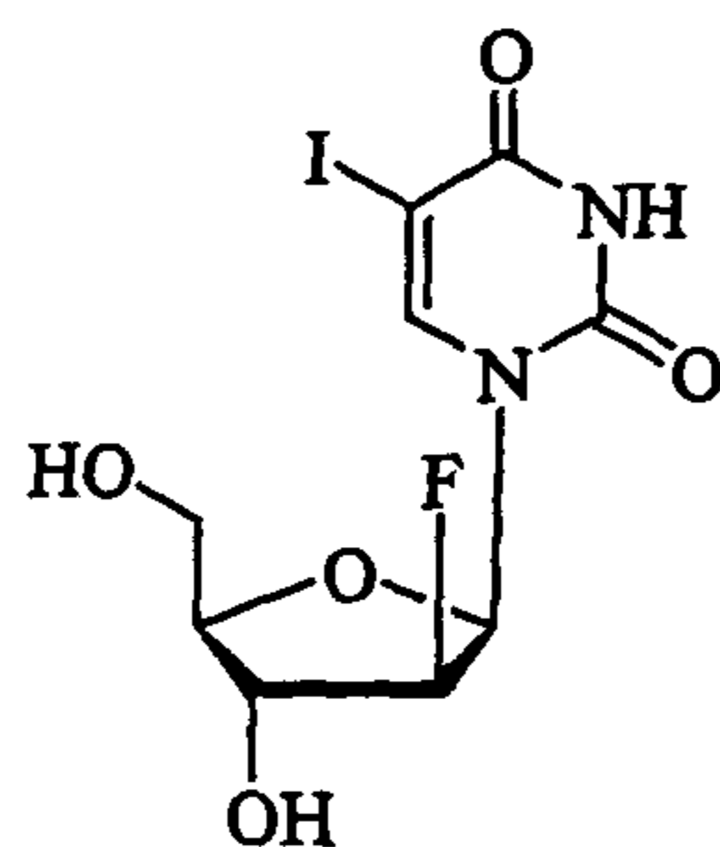
FIAU
