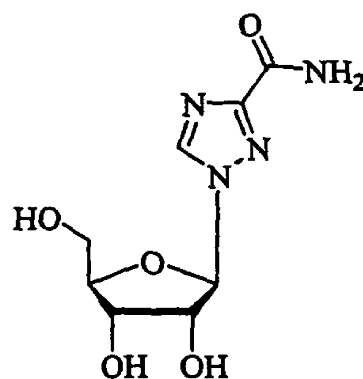
Ribavirin
