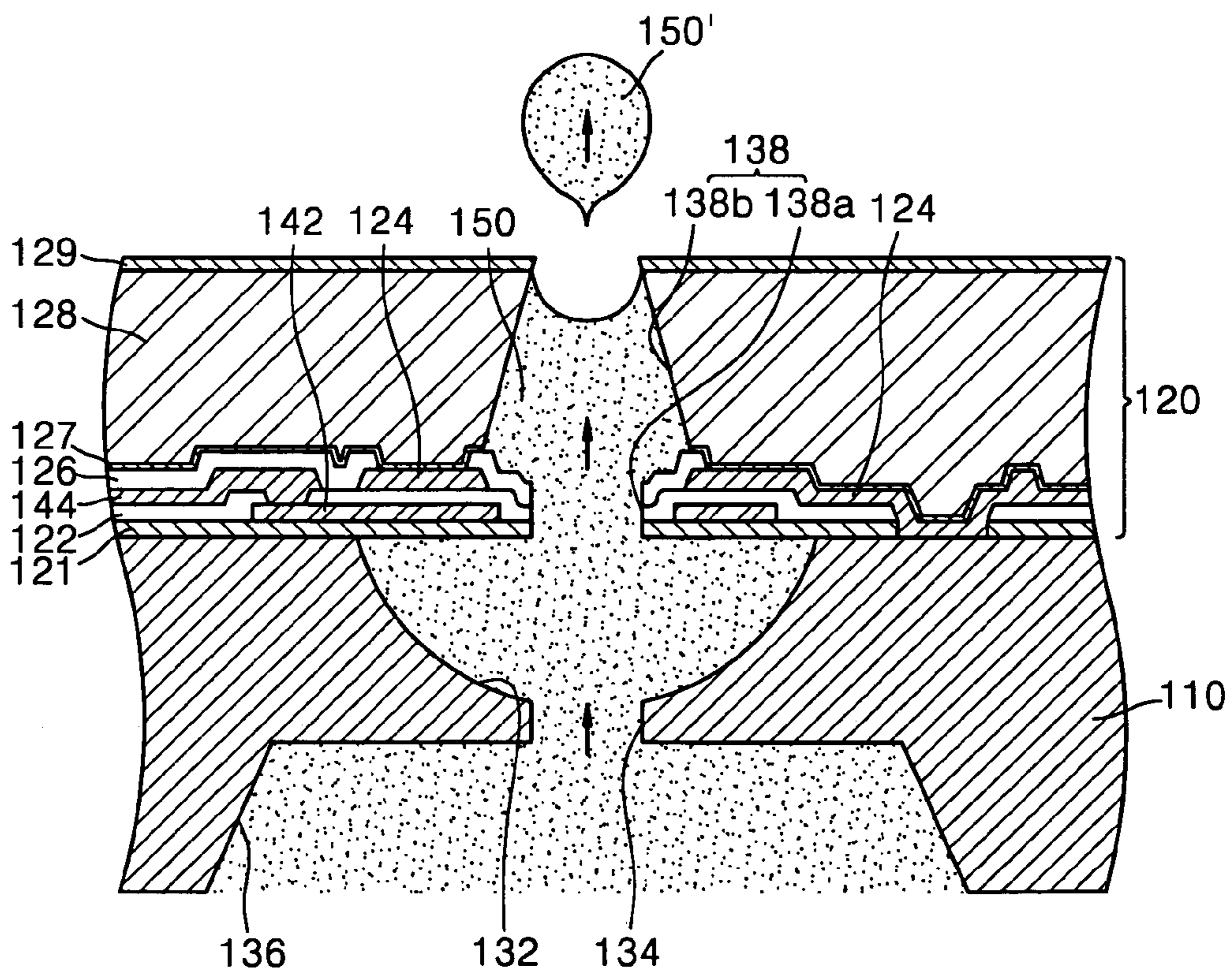
FIG. 4C
