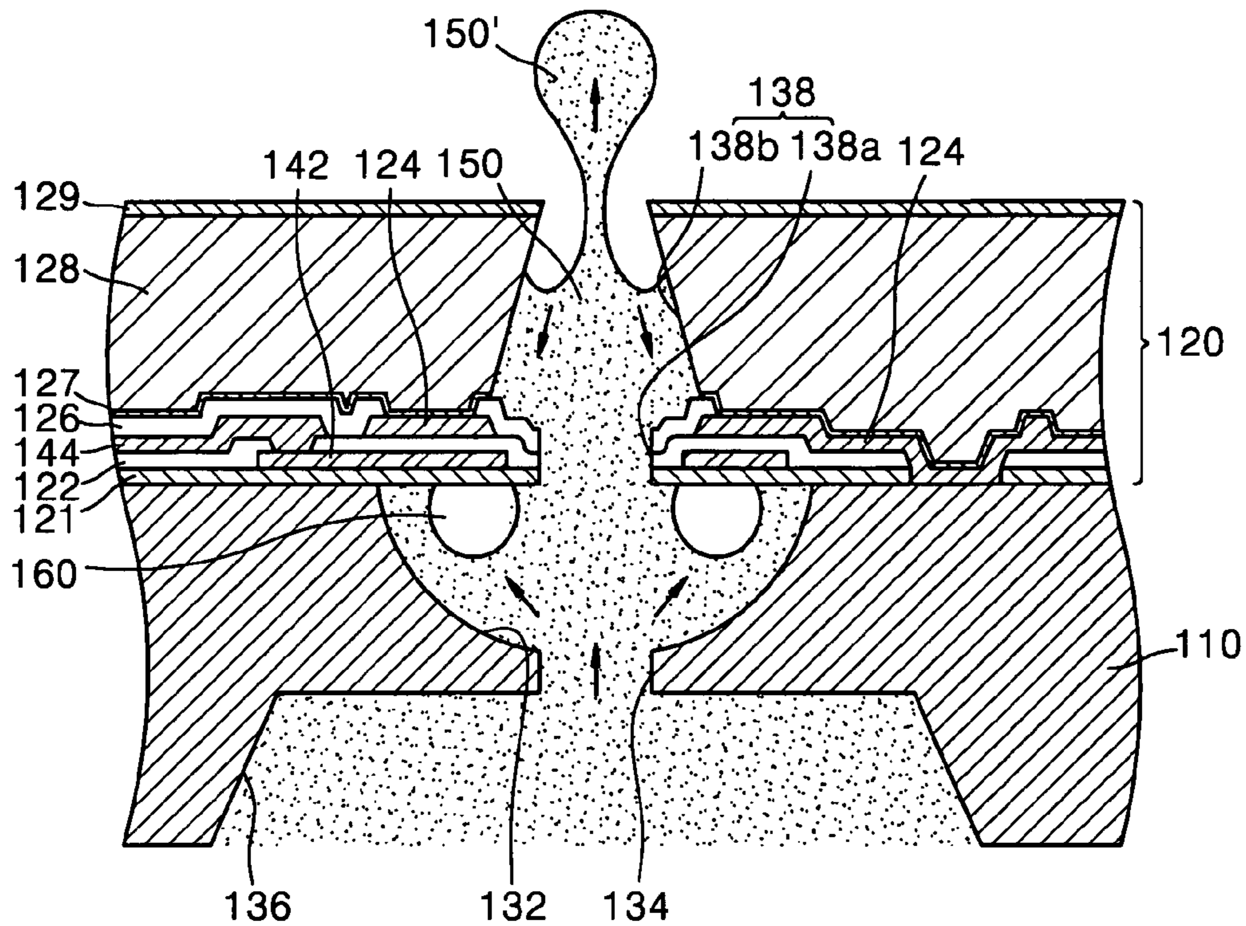
FIG. 4C
