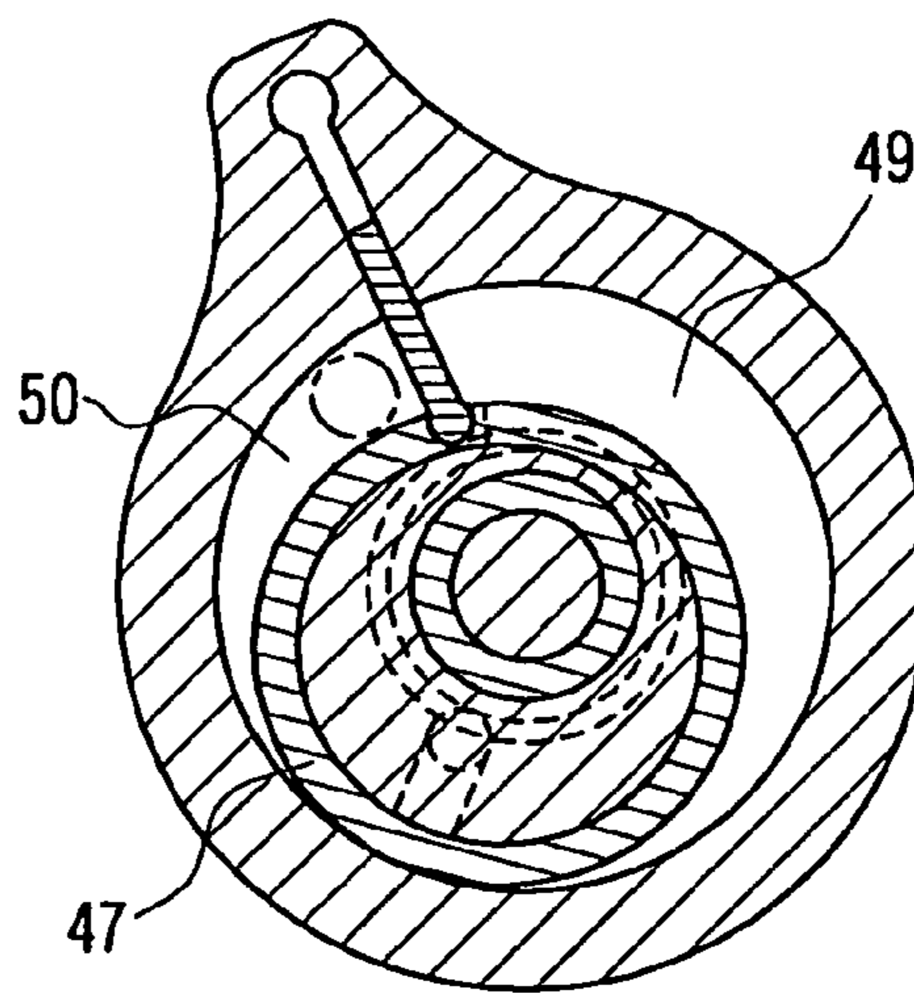
(ROTATIONAL ANGLE : 180° )
