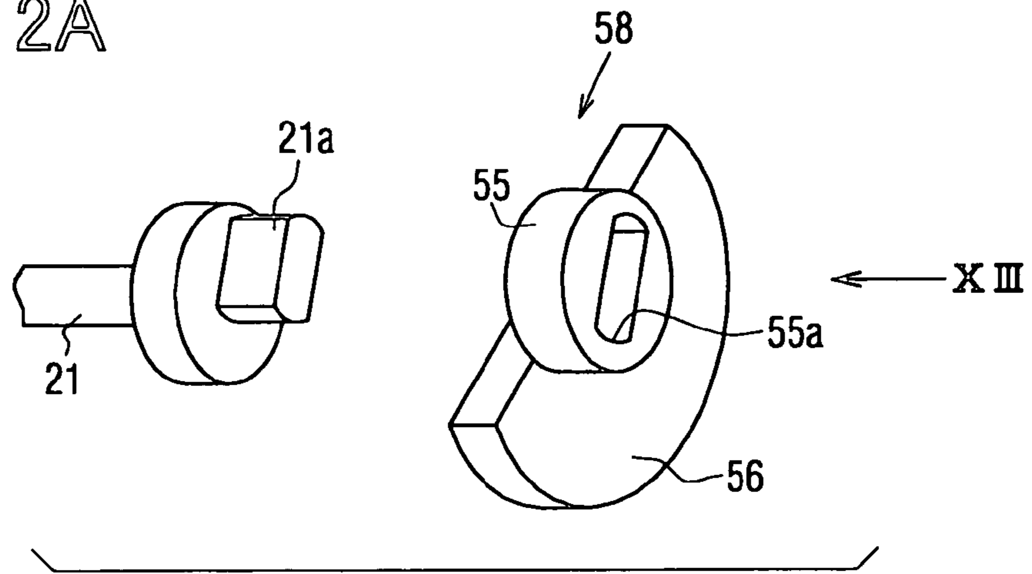
FIG. 12B
