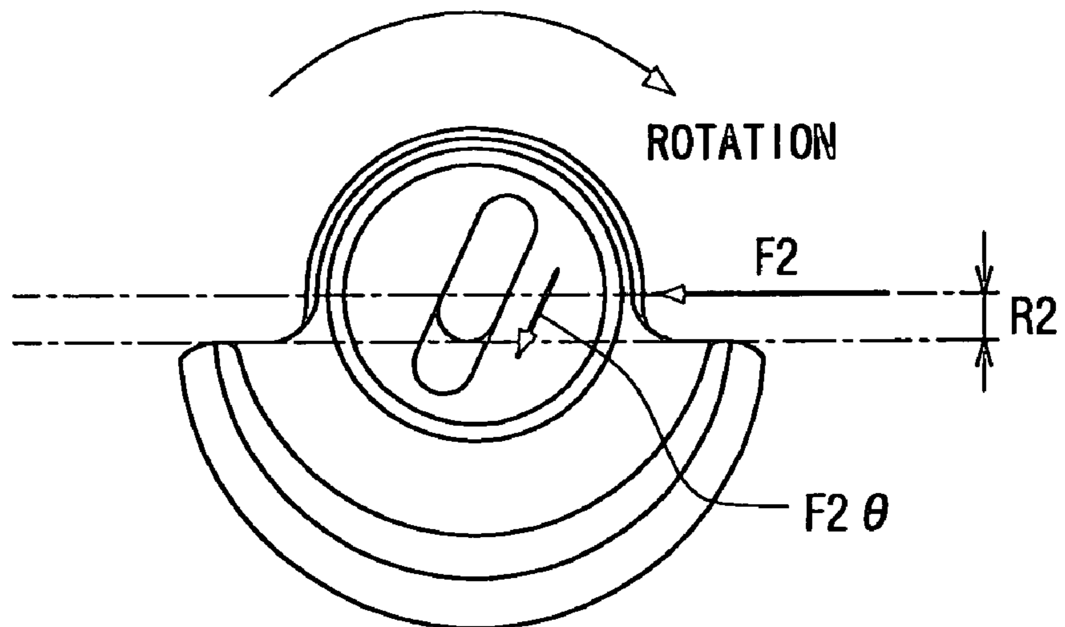
FIG. 14B
