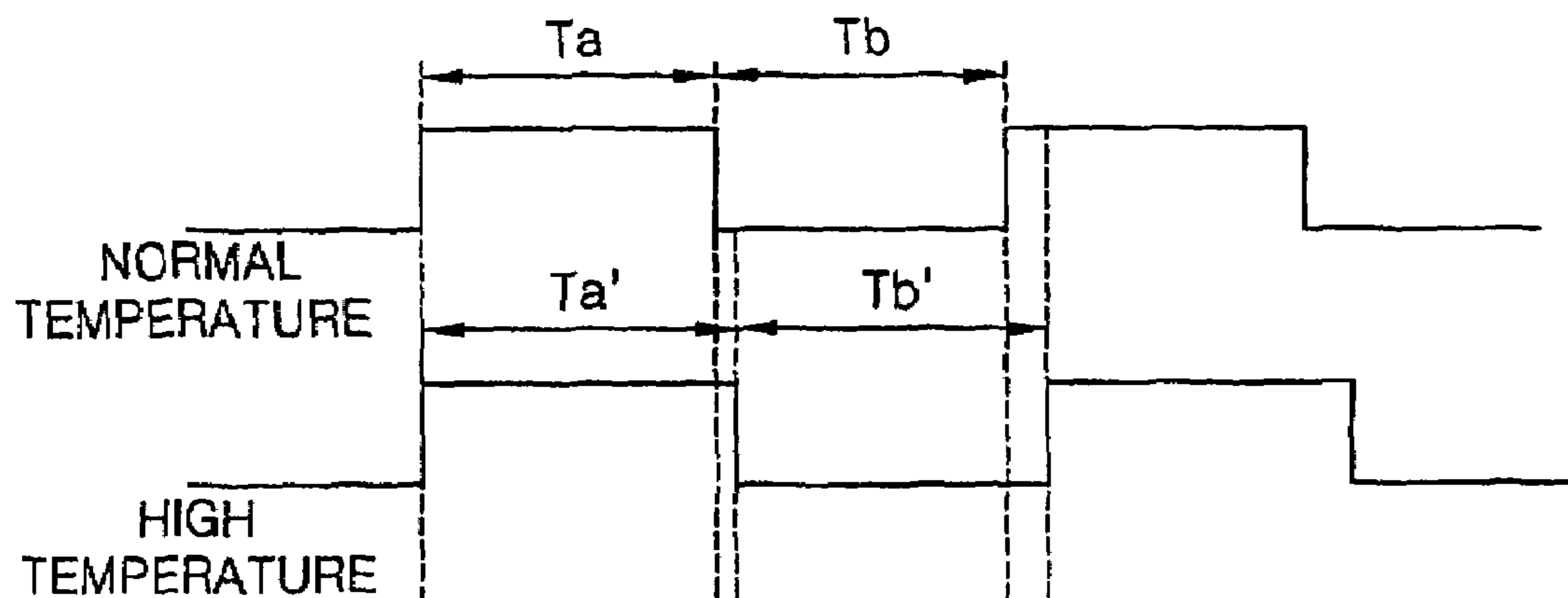
FIG. 9A
