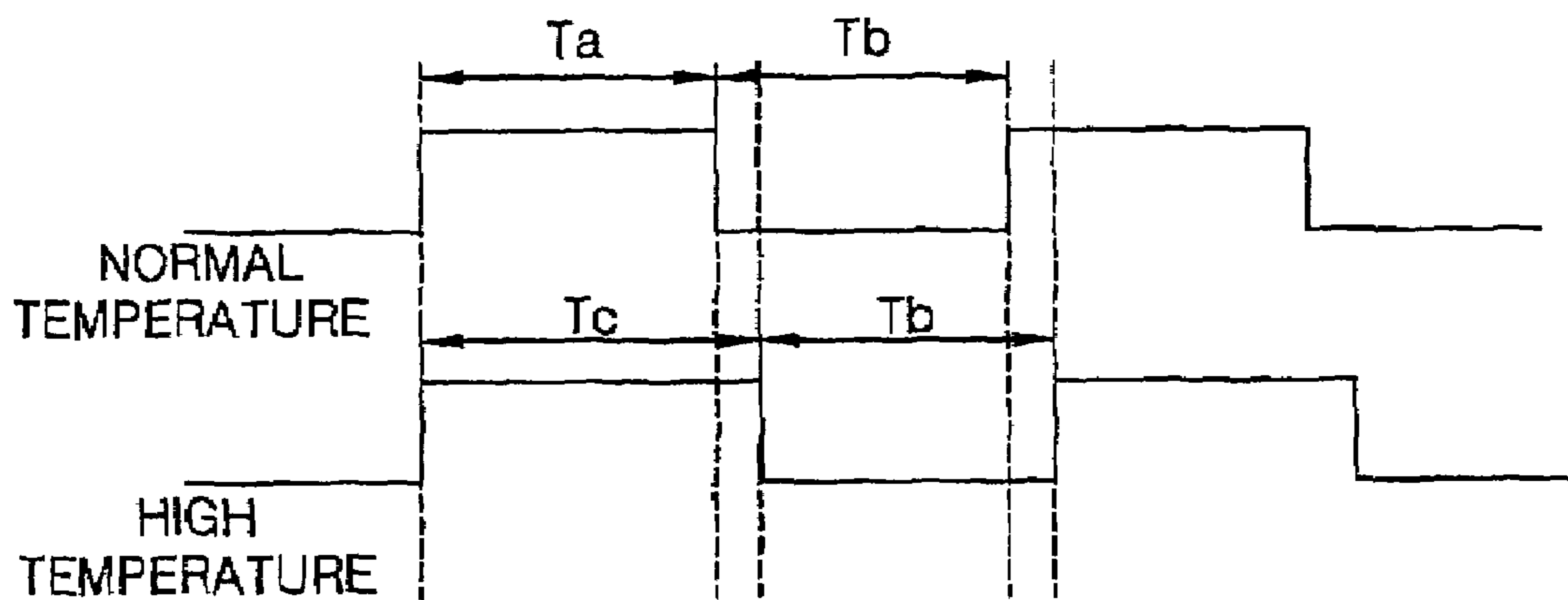
FIG. 9B
