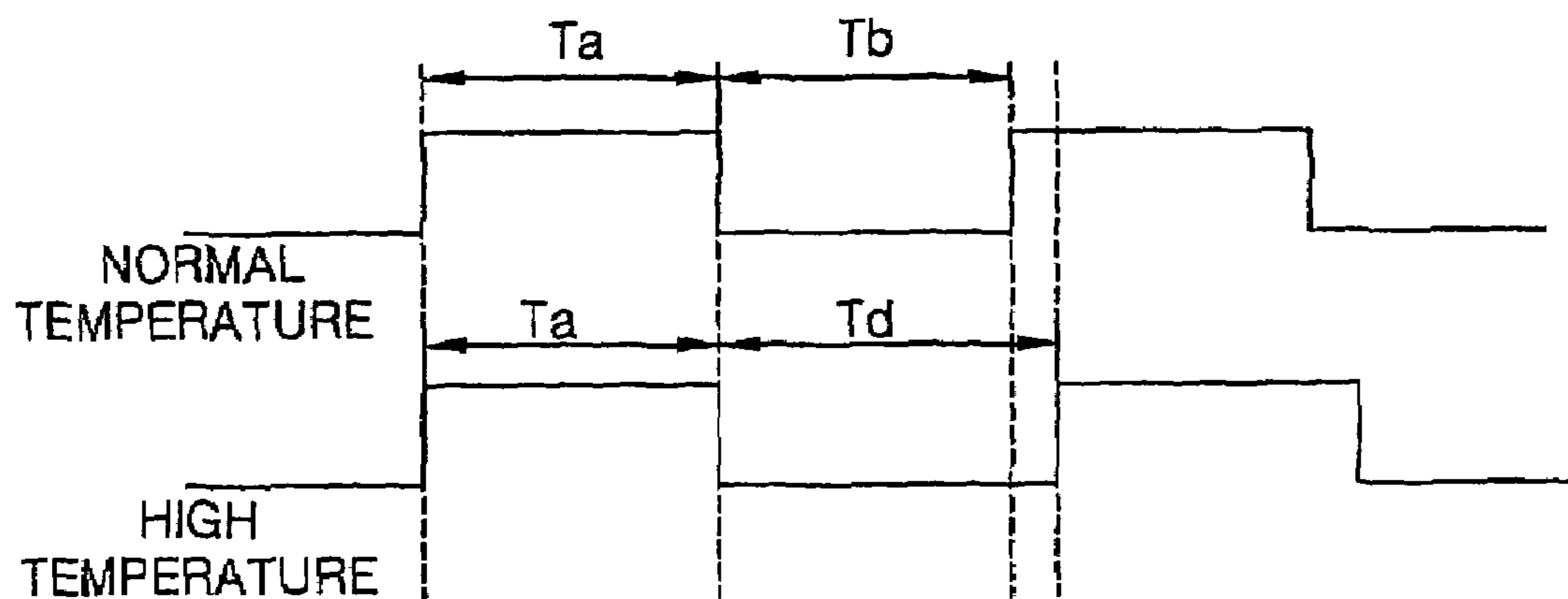
FIG. 9C
