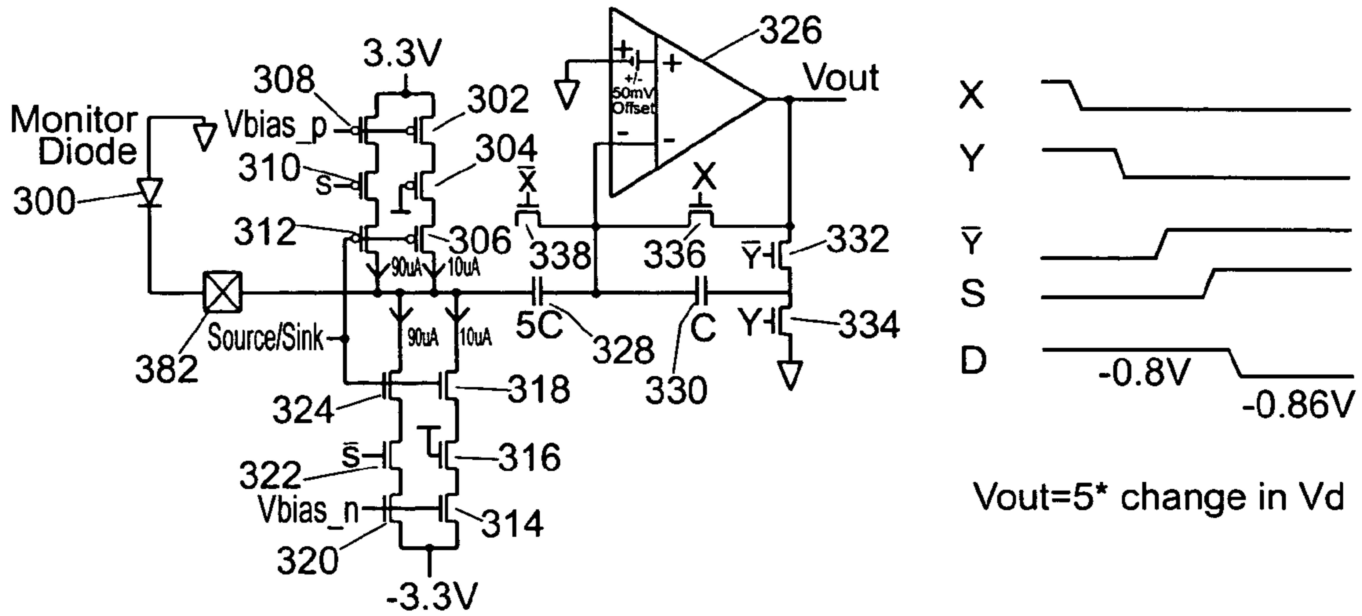
FIG. 10
