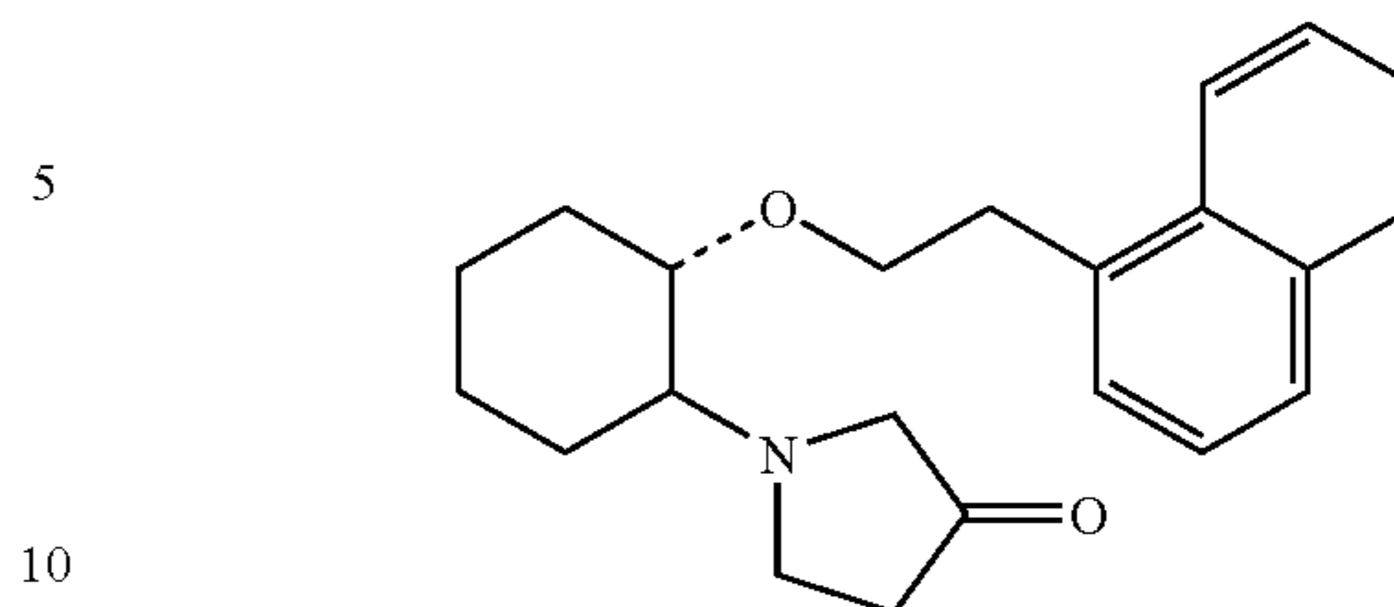
(1R,2R)/(1S,2S)-2-(3-ketopyrrolidinyl)-1-(1-naphthenethoxy)cyclohexane
