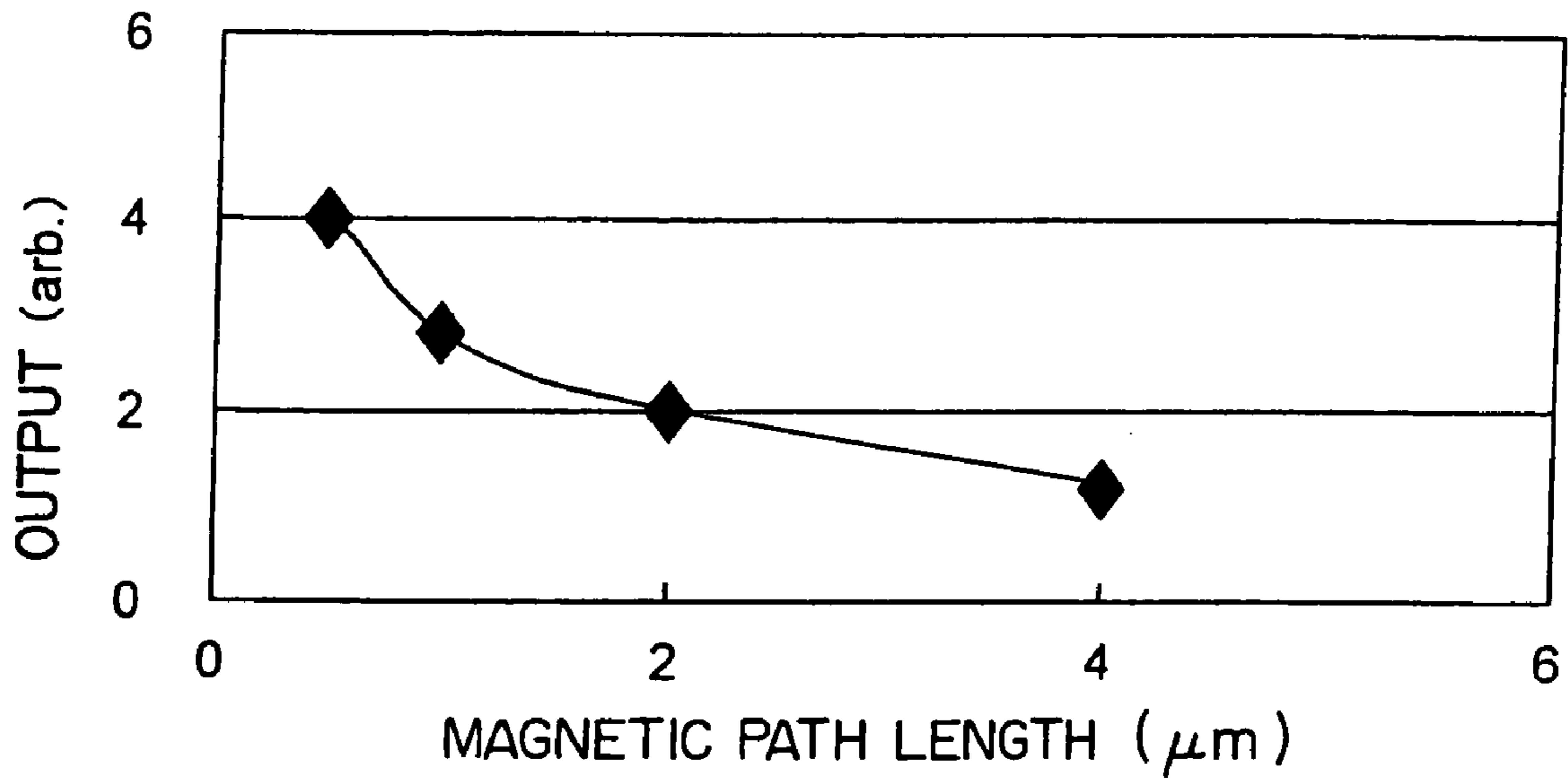
FIG. 18A
