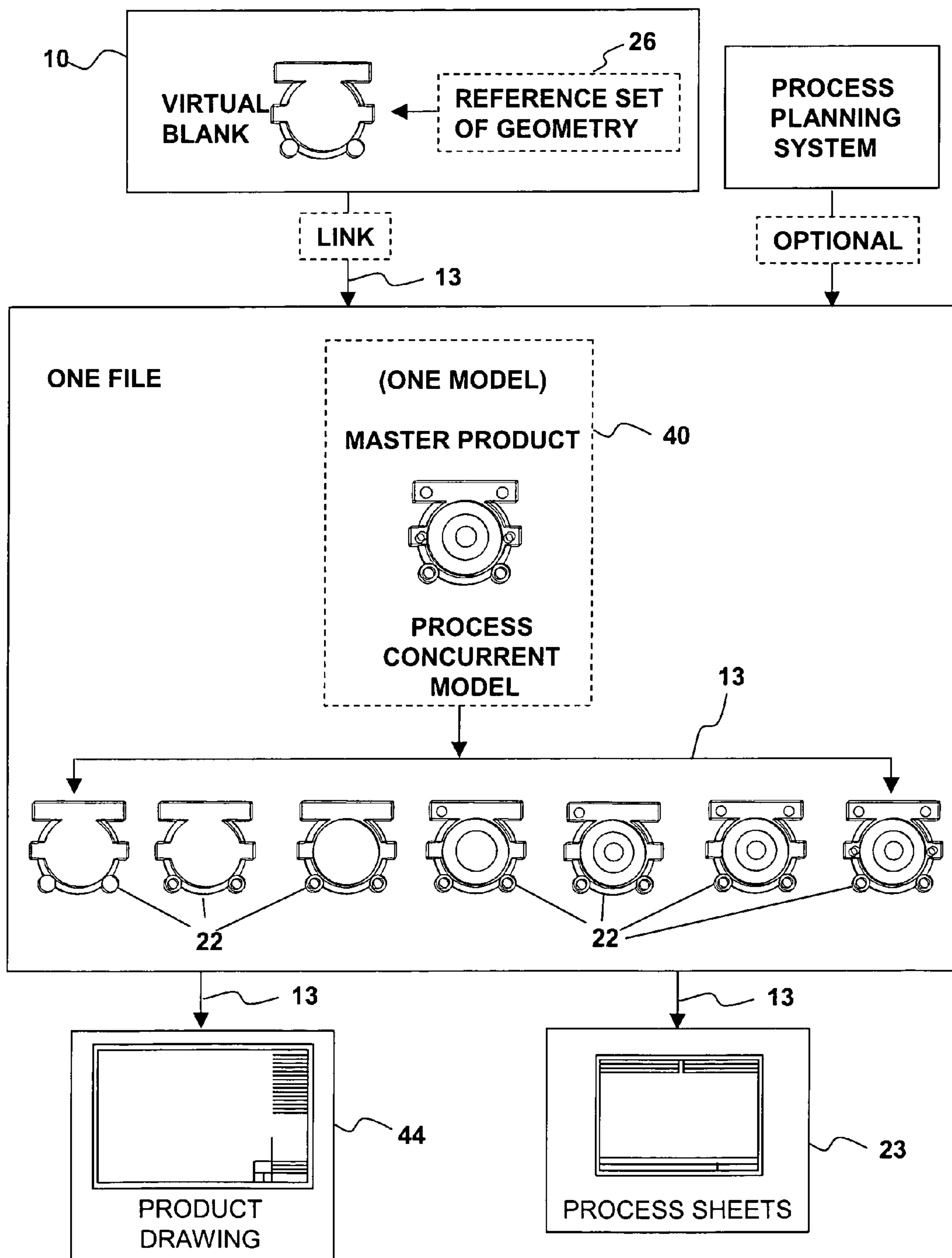
FIG. 14
