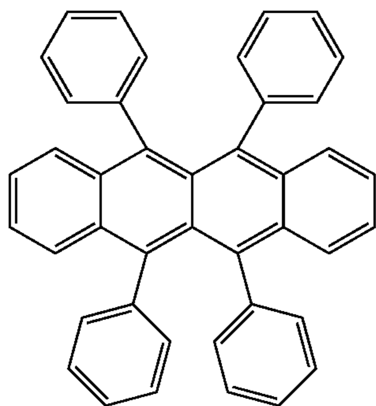
rubrene
