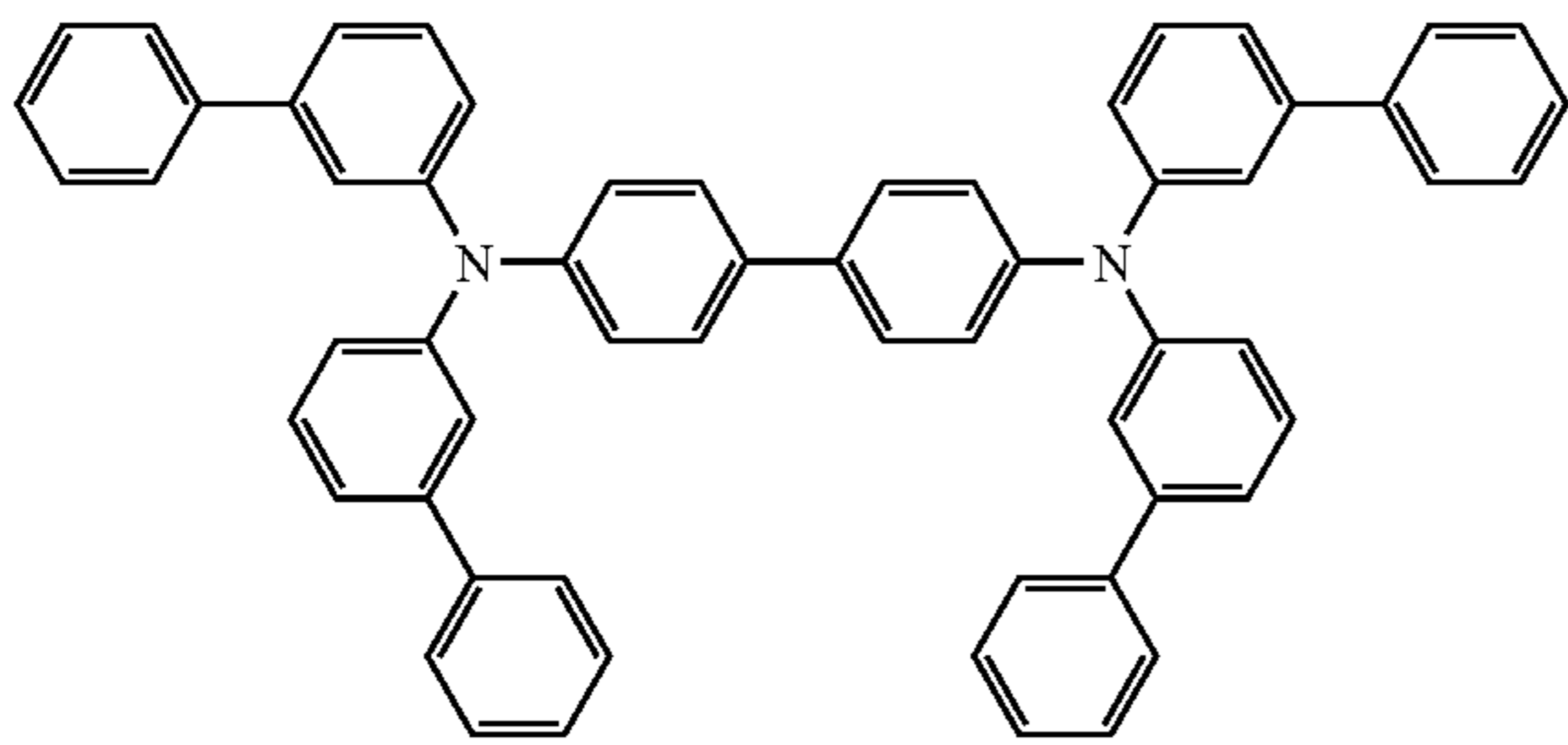
TPD
