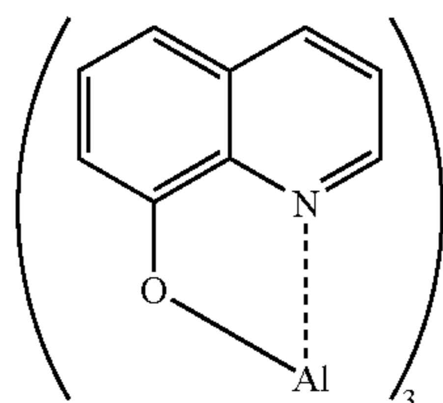
rubrene
