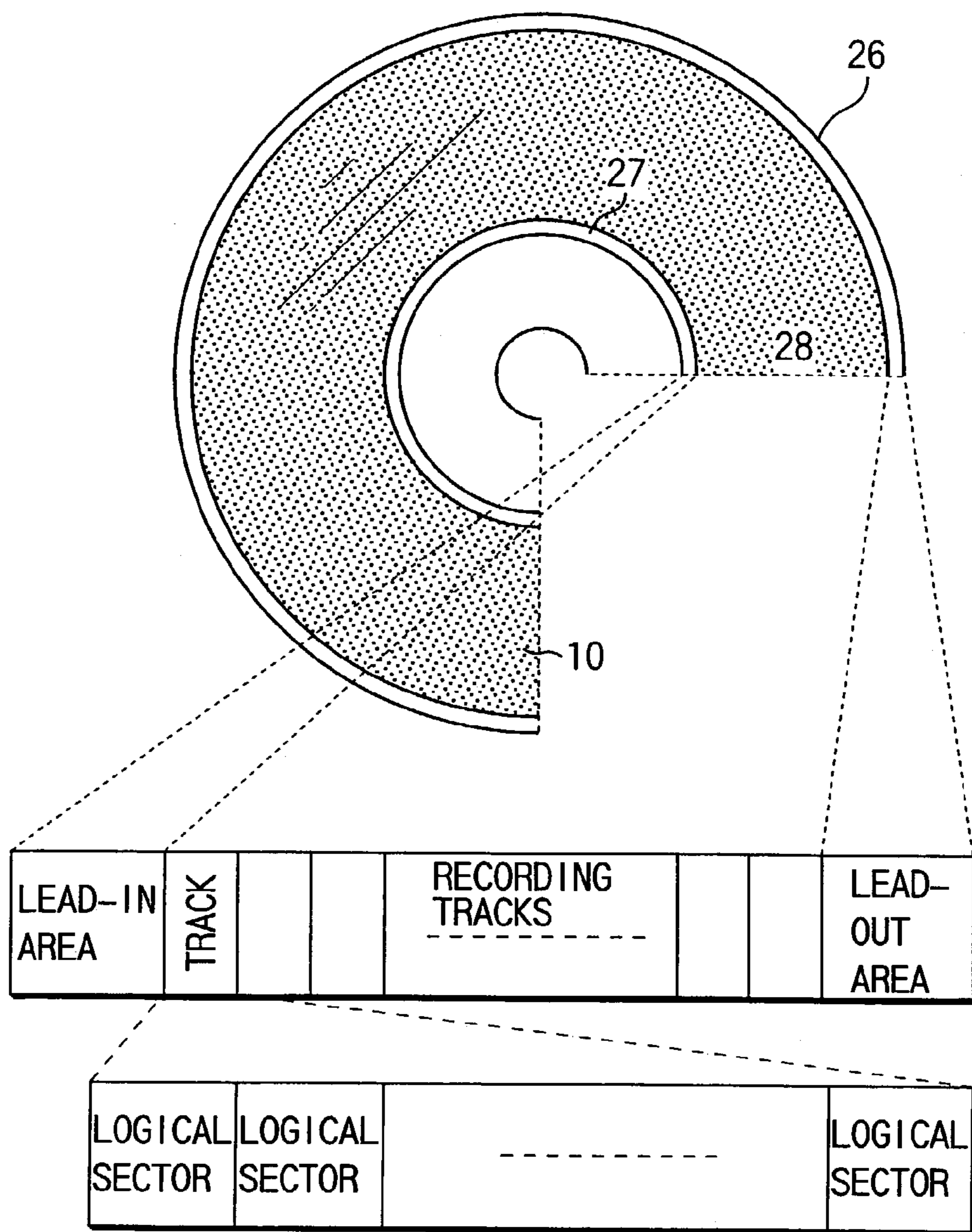
FIG. 2 ←→ 2048 BYTES (2k BYTES)
