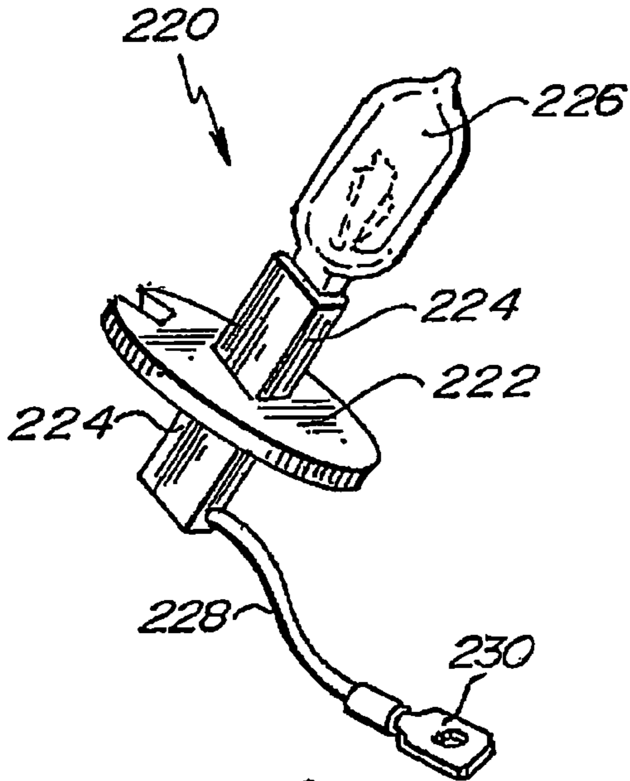
Fig. 18. PRIOR ART
