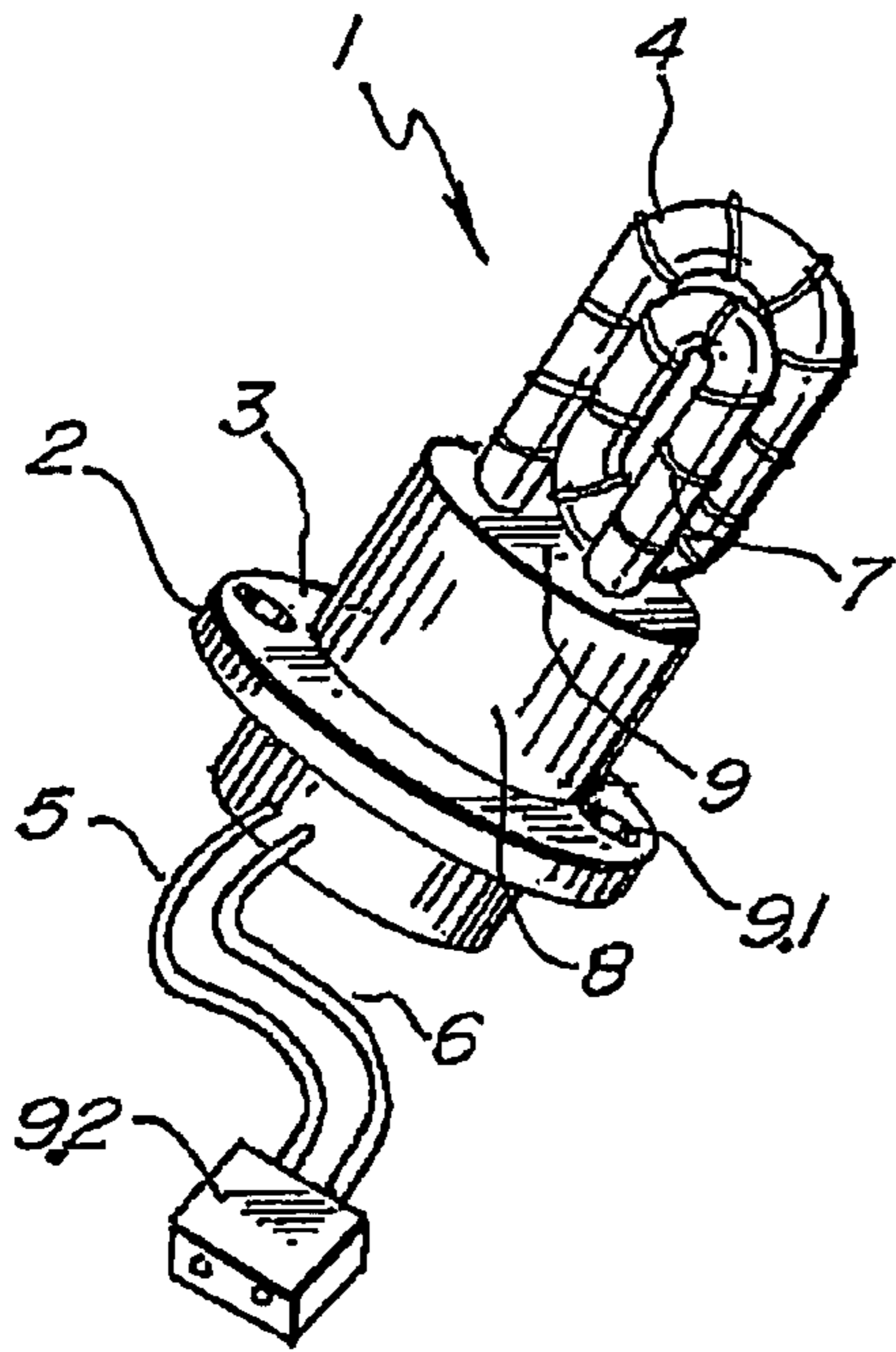
Fig. 16. PRIOR ART
