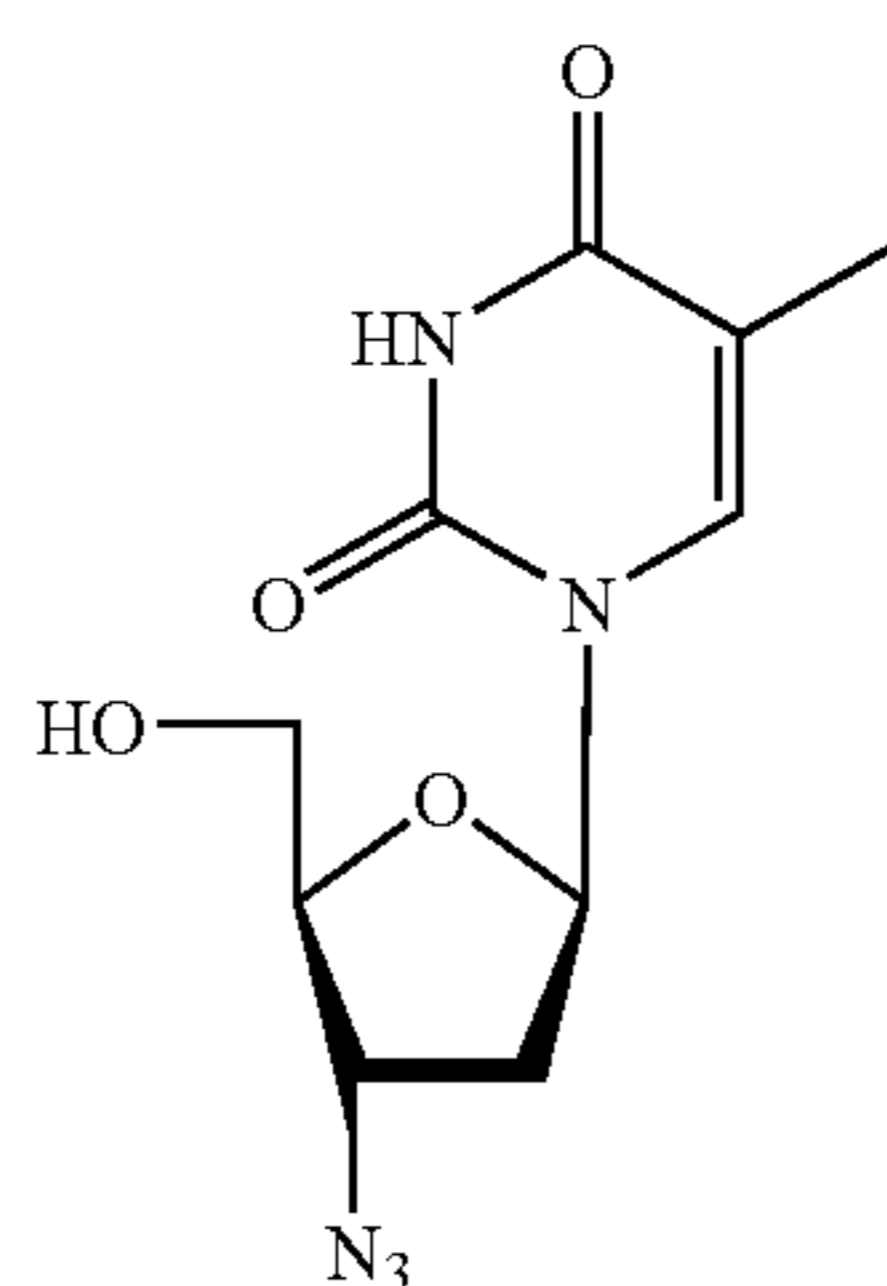
AZT
