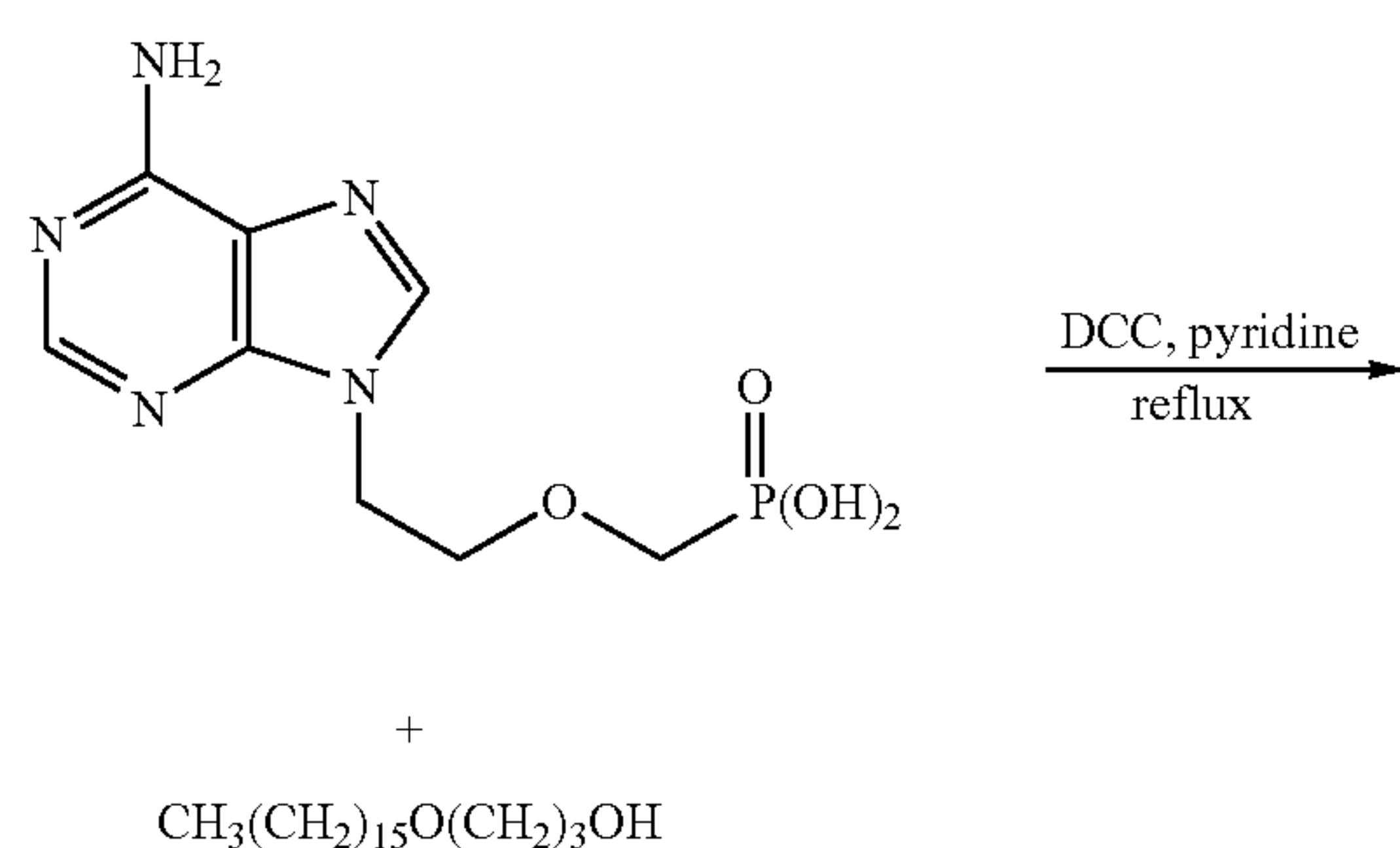
Scheme VI
