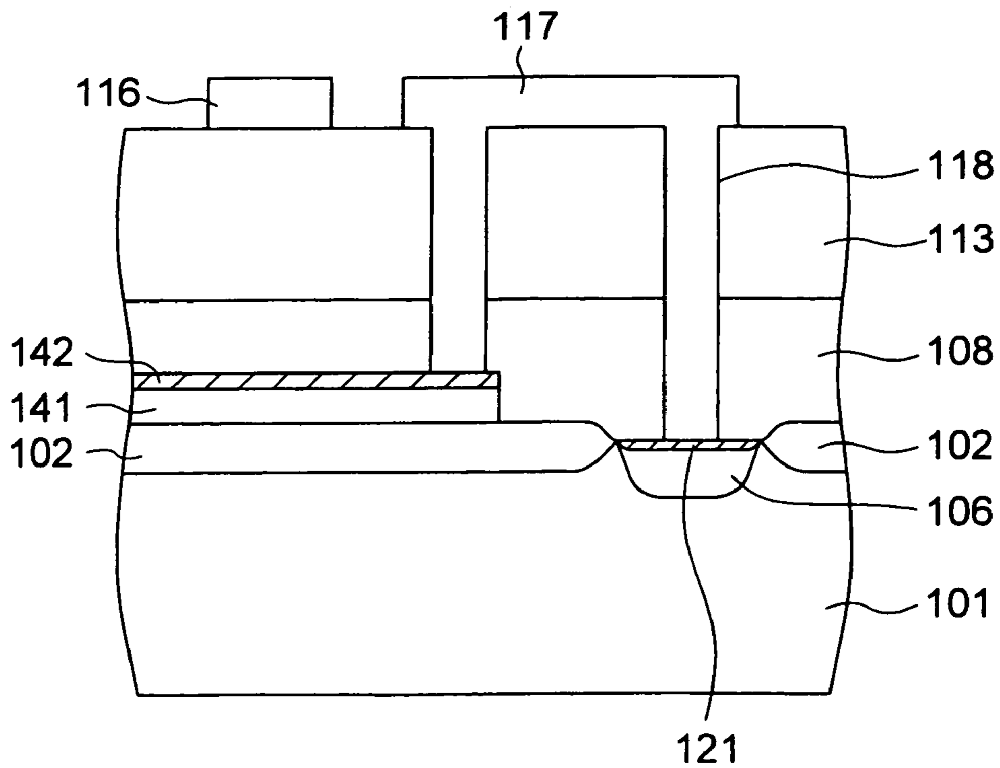
FIG. 6B d-d' SECTION
