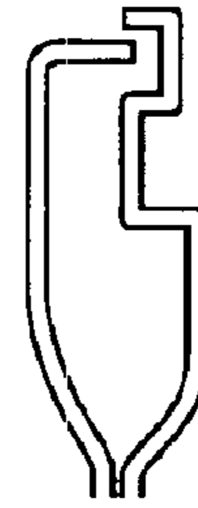
Tongue & Groove
