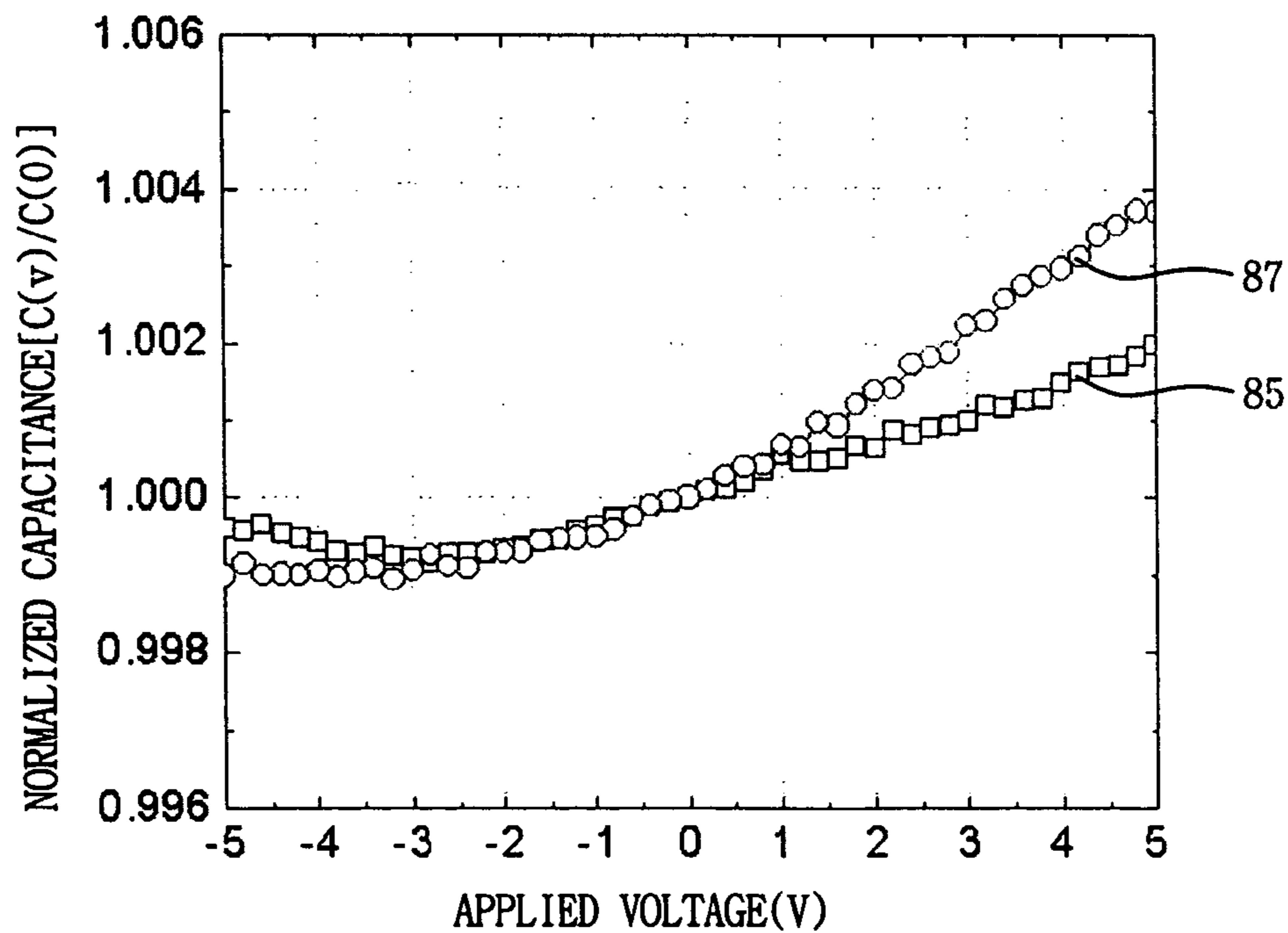
FIG. 7B
