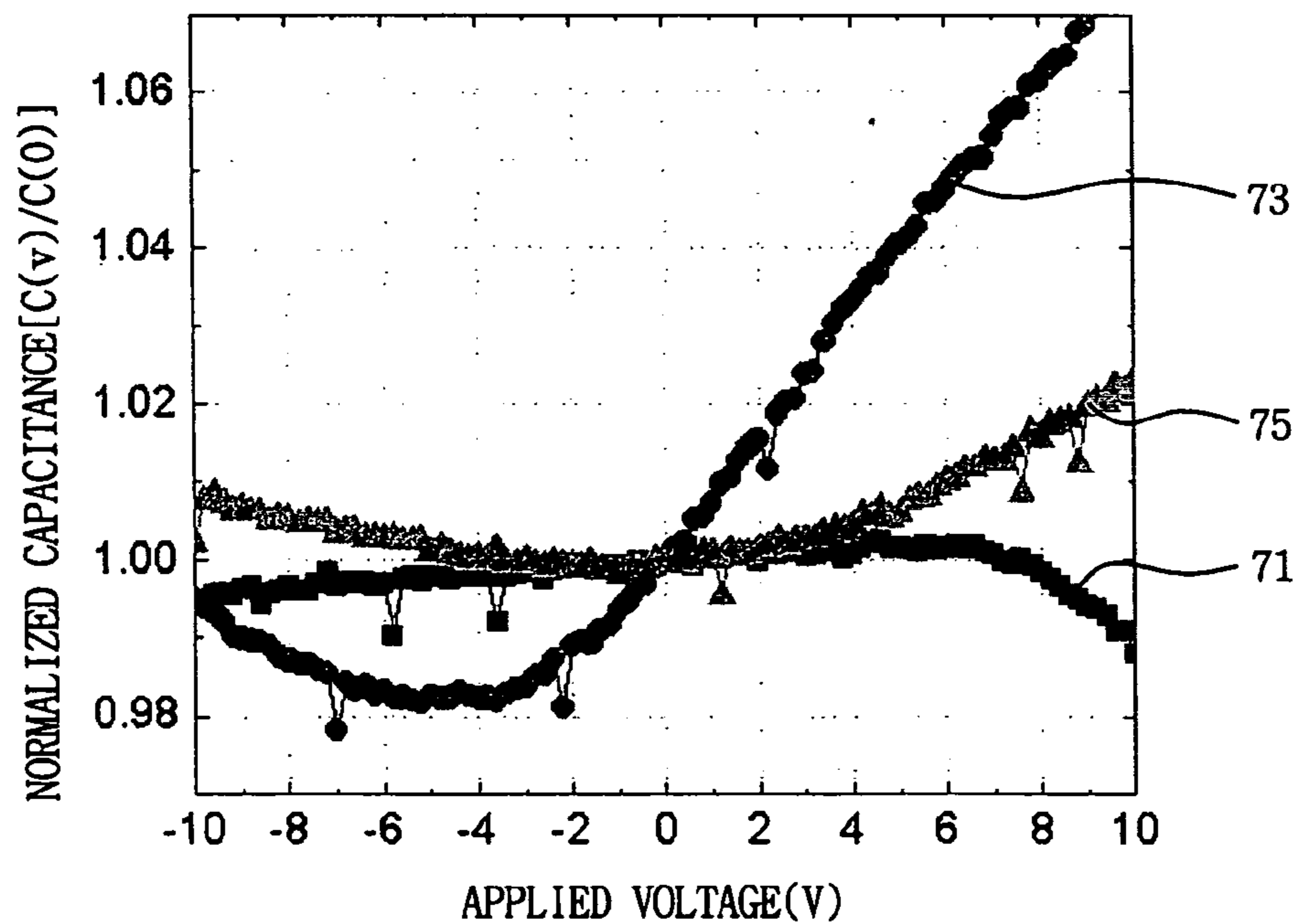
FIG. 4B
