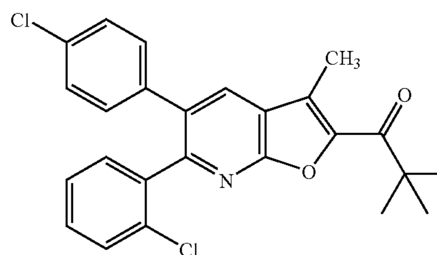
1-[6-(2-Chlorophenyl)-5-(4-chlorophenyl)-3-methylfuro[2,3-b]pyridin-2-yl]-2,2-dimethylpropan-1-one
