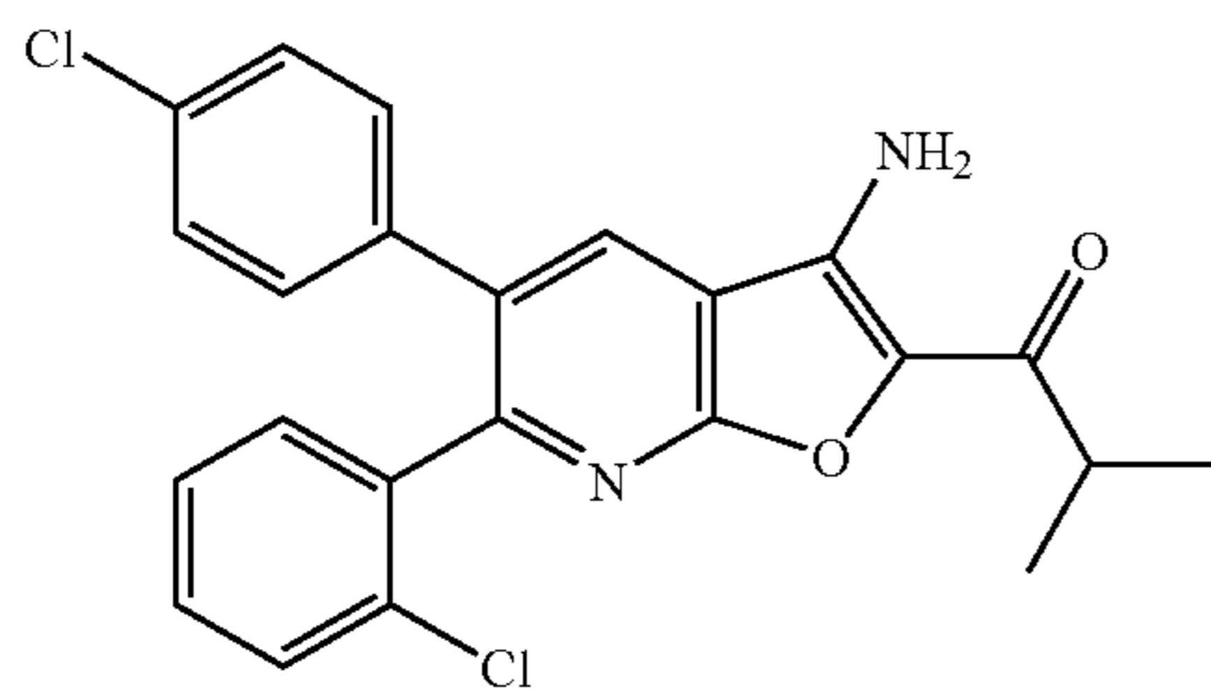
1-[3-Amino-6-(2-chlorophenyl)-5-(4-chlorophenyl) furo[2,3-b]pyridin-2-yl]-2-methylpropan-1-one
