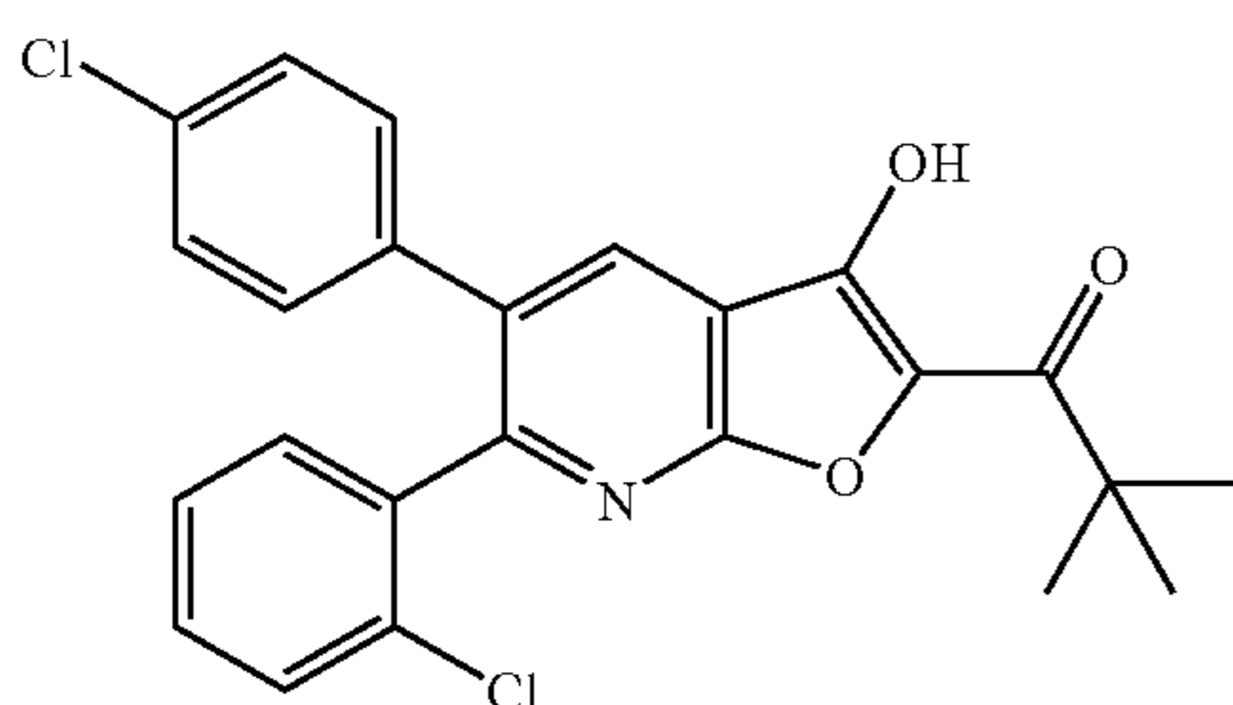
1-[6-(2-Chlorophenyl)-5-(4-chlorophenyl)-3-hydroxyfuro[2,3-b]pyridin-2-yl]-2,2-dimethylpropan-1-one
