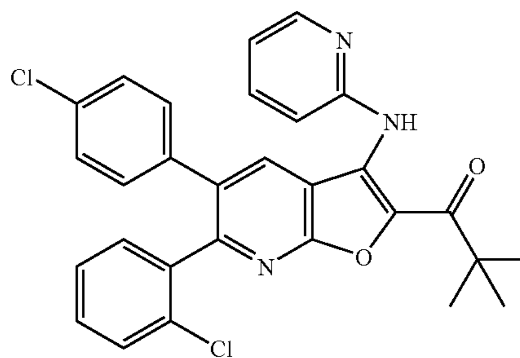
1-[6-(2-Chlorophenyl)-5-(4-chlorophenyl)-3-(pyridin-2-ylamino)furo[2,3-b]pyridin-2-yl]-2,2-dimethylpropan-1-one
