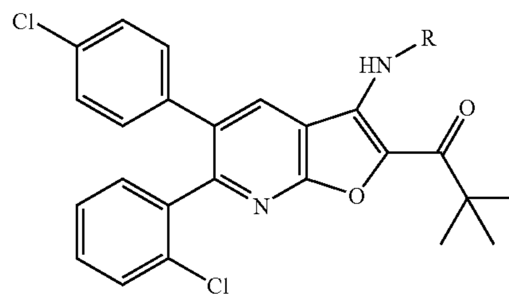
1-[3-(Allylamino)-6-(2-chlorophenyl)-5-(4-chlorophenyl)furo[2,3-b]pyridin-2-yl]-2,2-dimethylpropan-1-one (R=allyl)
