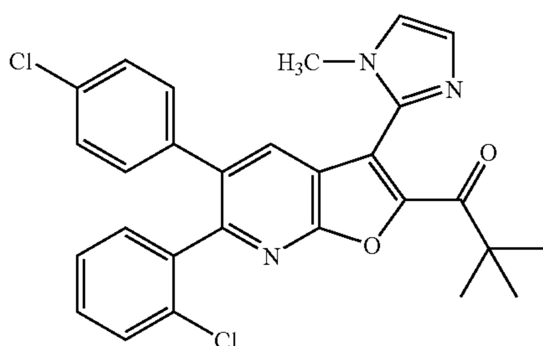
1-[6-(2-Chlorophenyl)-5-(4-chlorophenyl)-3-(1-methyl-1H-imidazol-2-yl)furo[2,3-b]pyridin-2-yl]-2,2-dimethylpropan-1-one
