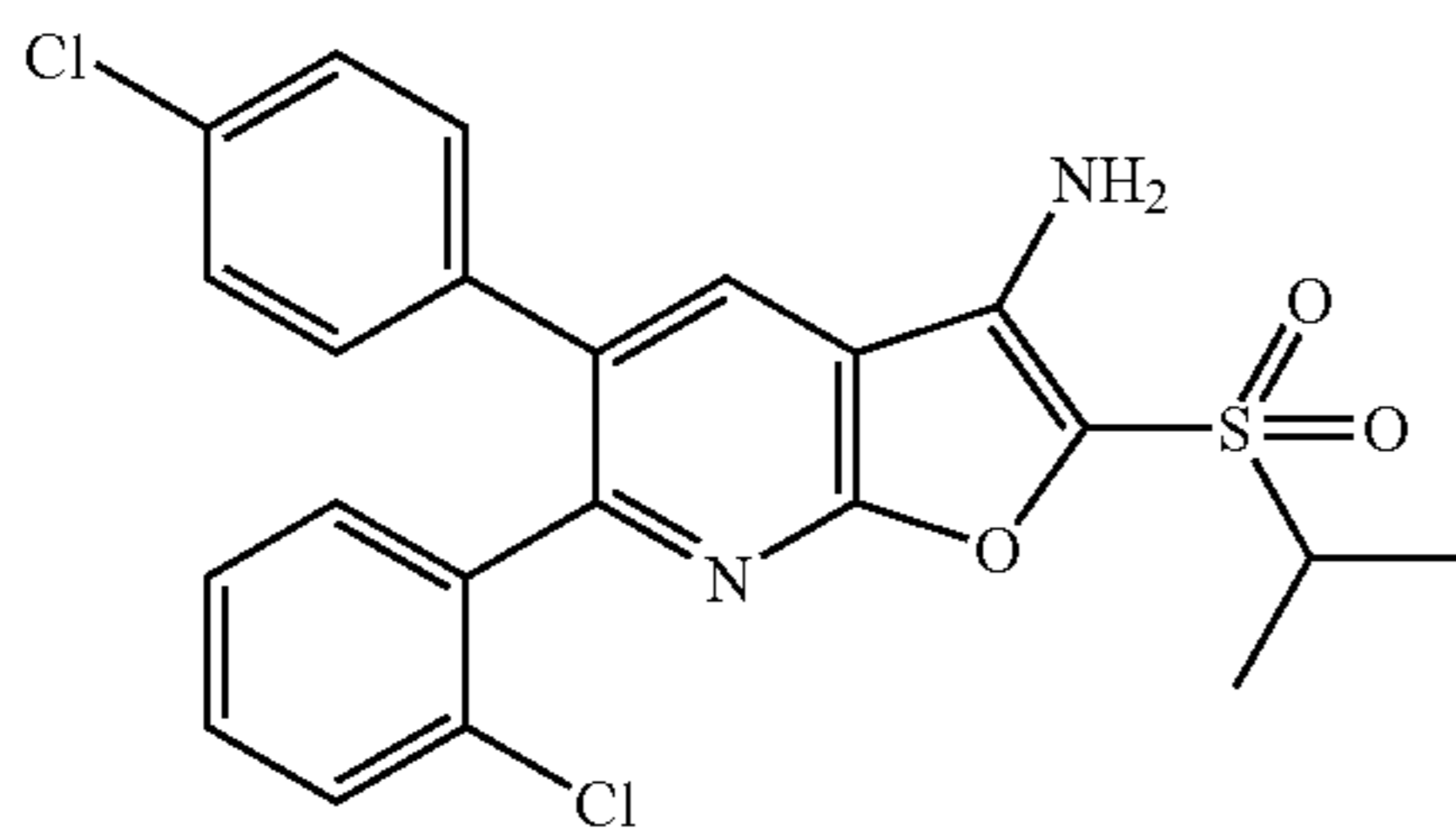
2-(Tert-butylsulfonyl)-6-(2-chlorophenyl)-5-(4-chlorophenyl)furo[2,3-b]pyridin-3-amine
