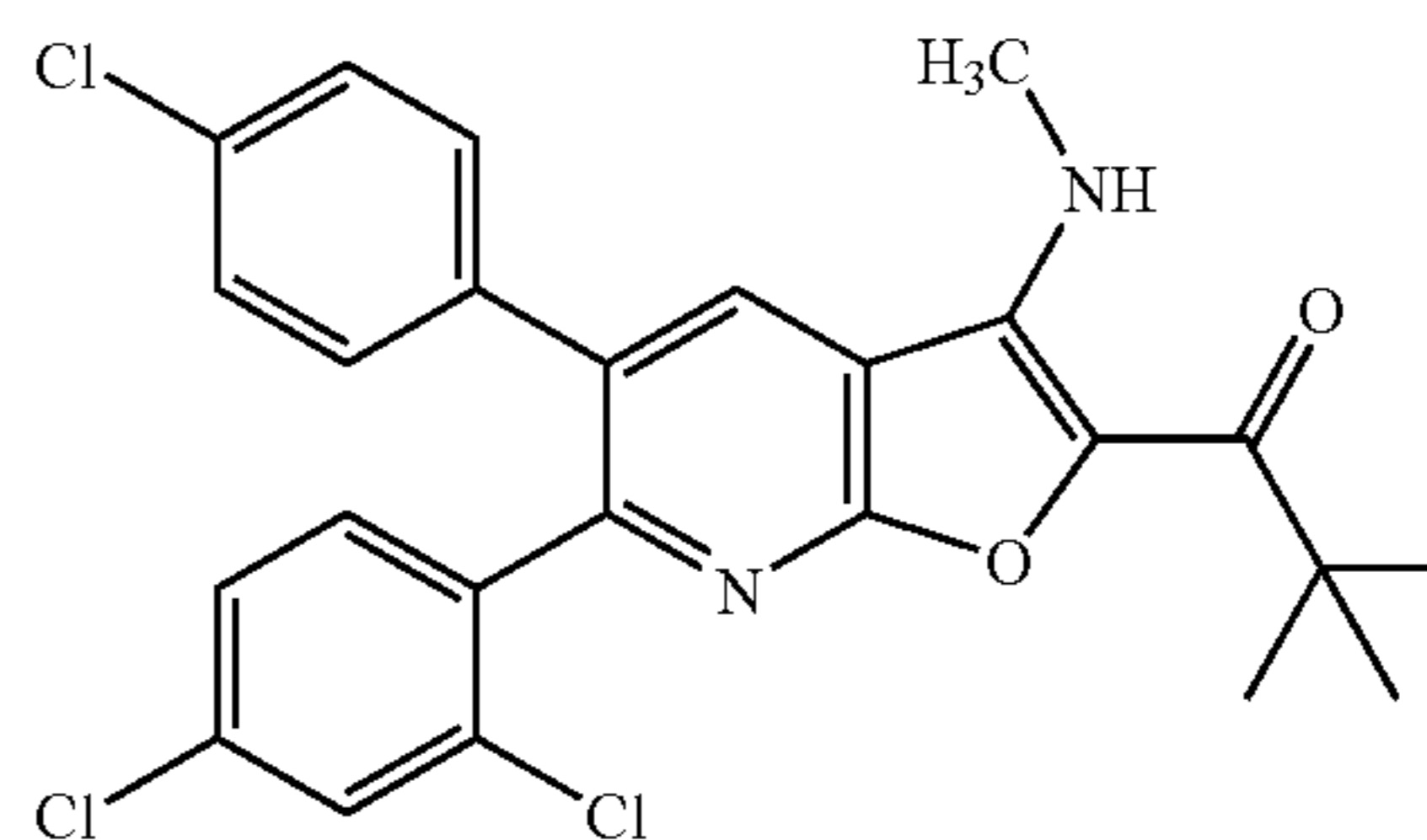
1-[5-(4-Chlorophenyl)-6-(2,4-dichlorophenyl)-3-(methylamino)furo[2,3-b]pyridin-2-yl]-2,2-dimethylpropan-1-one
