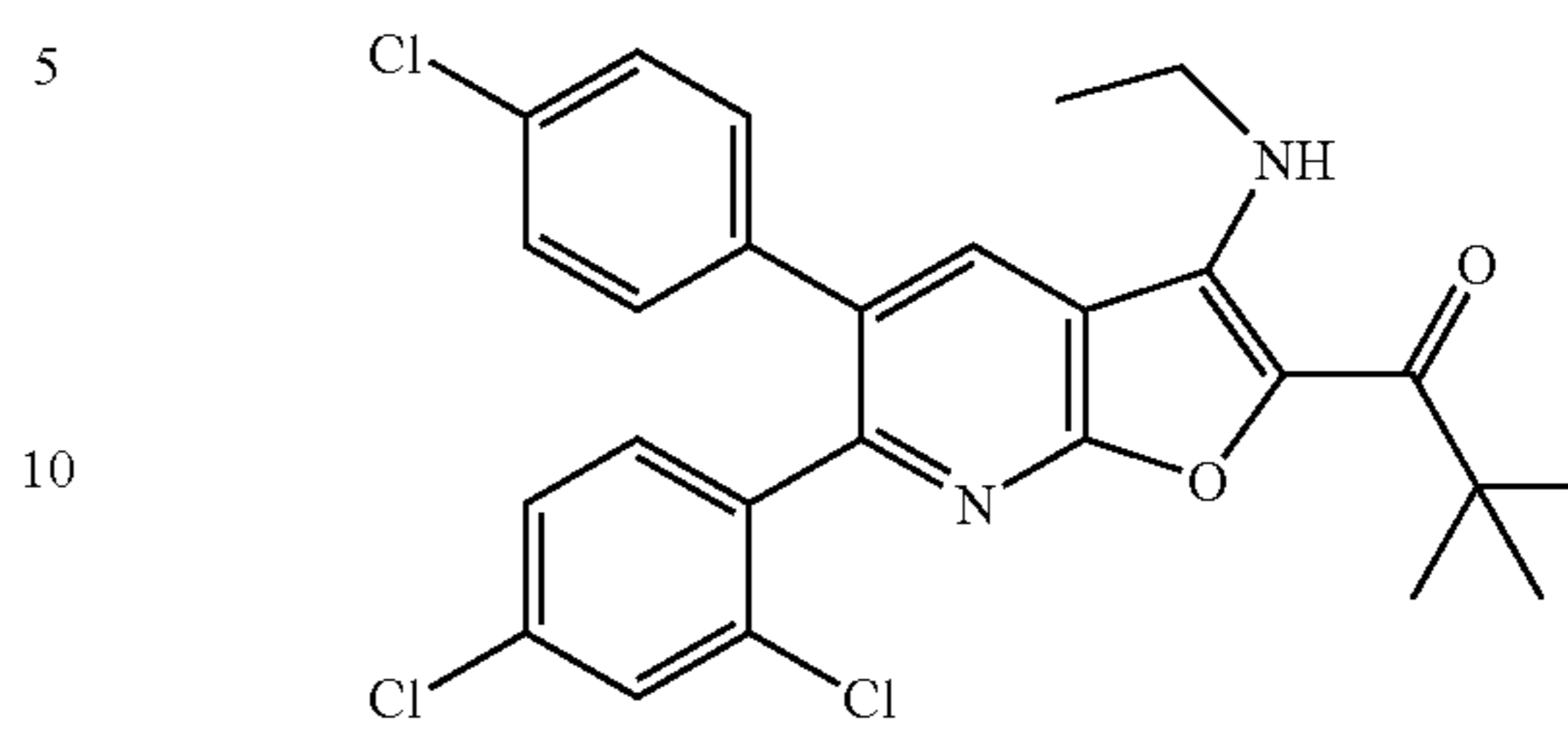
1-[5-(4-Chlorophenyl)-6-(2,4-dichlorophenyl)-3-(ethylamino)furo[2,3-b]pyridin-2-yl]-2,2-dimethylpropan-1-one
