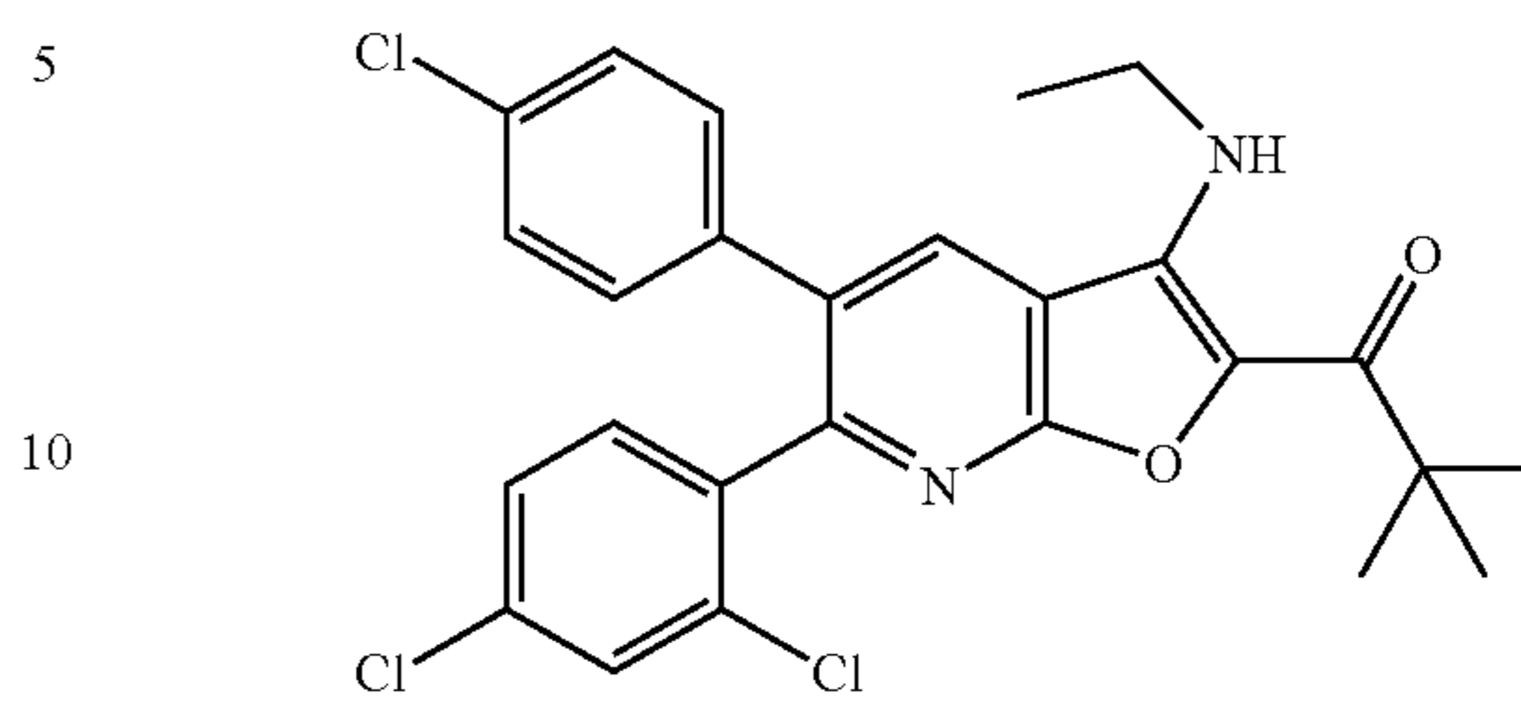
1-[5-(4-Chlorophenyl)-6-(2,4-dichlorophenyl)-3-(ethylamino)furo[2,3-b]pyridin-2-yl]-2,2-dimethylpropan-1-one
