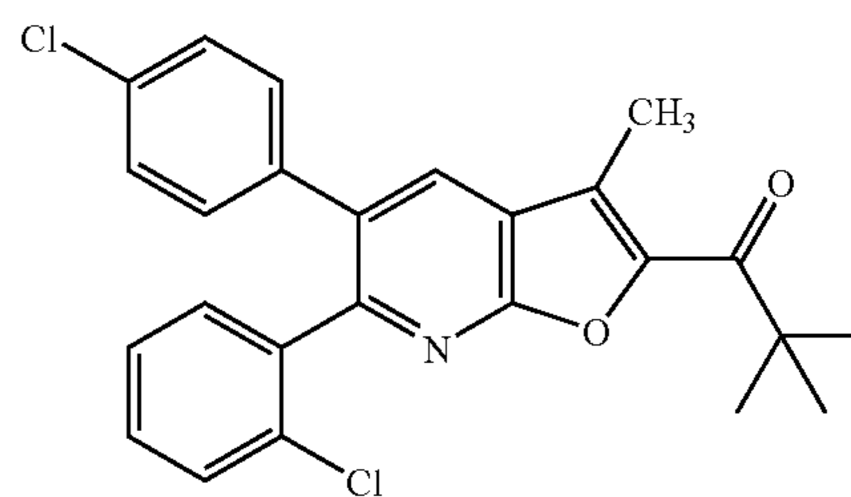
1-[6-(2-Chlorophenyl)-5-(4-chlorophenyl)-3-methylfuro[2,3-b]pyridin-2-yl]-2,2-dimethylpropan-1-one
