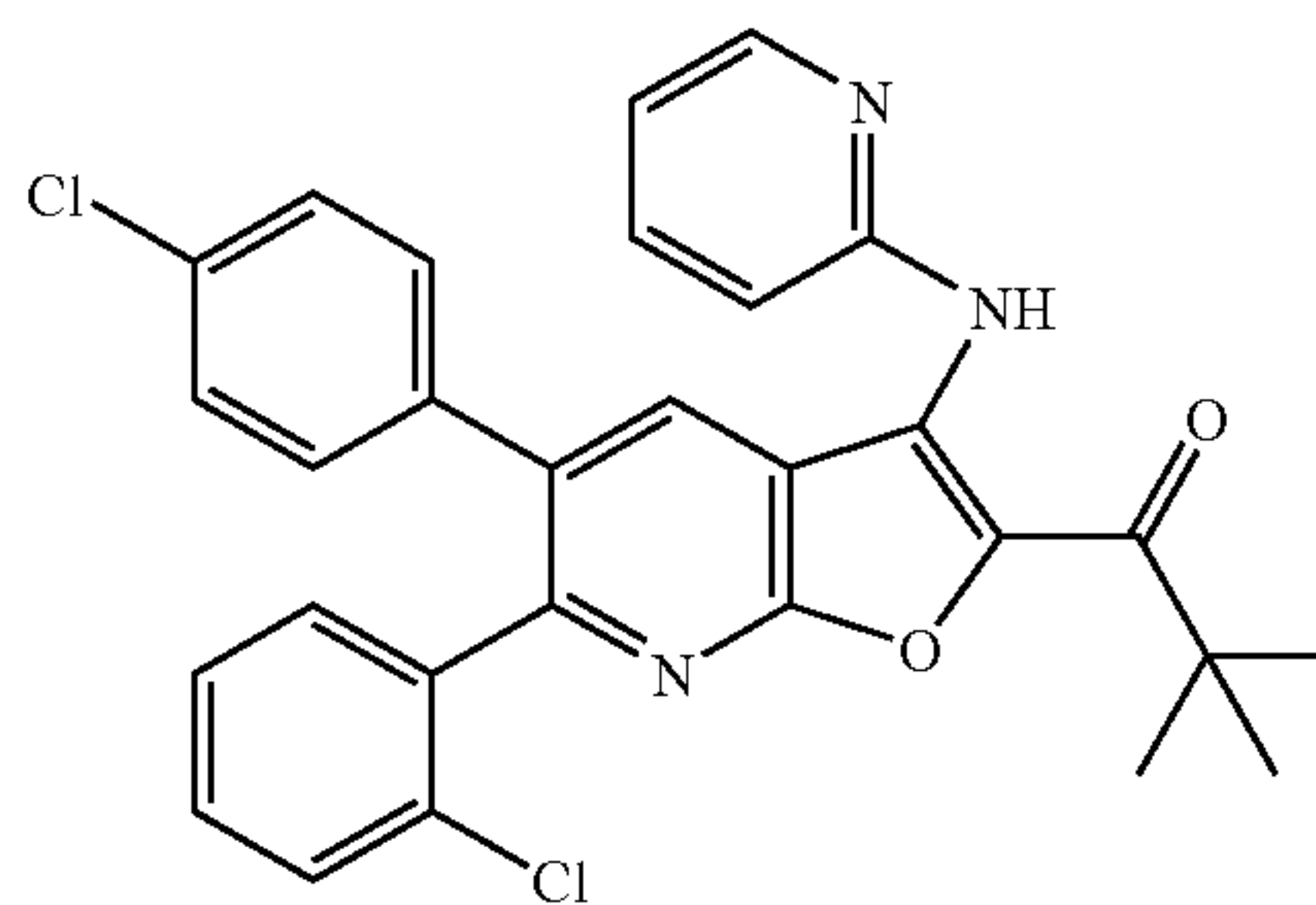
1-[6-(2-Chlorophenyl)-5-(4-chlorophenyl)-3-(pyridin-2-ylamino)furo[2,3-b]pyridin-2-yl]-2,2-dimethylpropan-1-one
