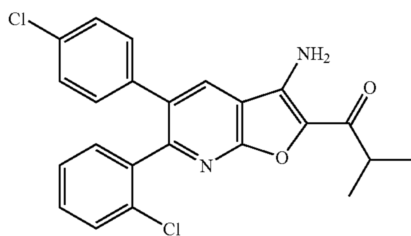
1-[3-Amino-6-(2-chlorophenyl)-5-(4-chlorophenyl)furo[2,3-b]pyridin-2-yl]-2-methylpropan-1-one
