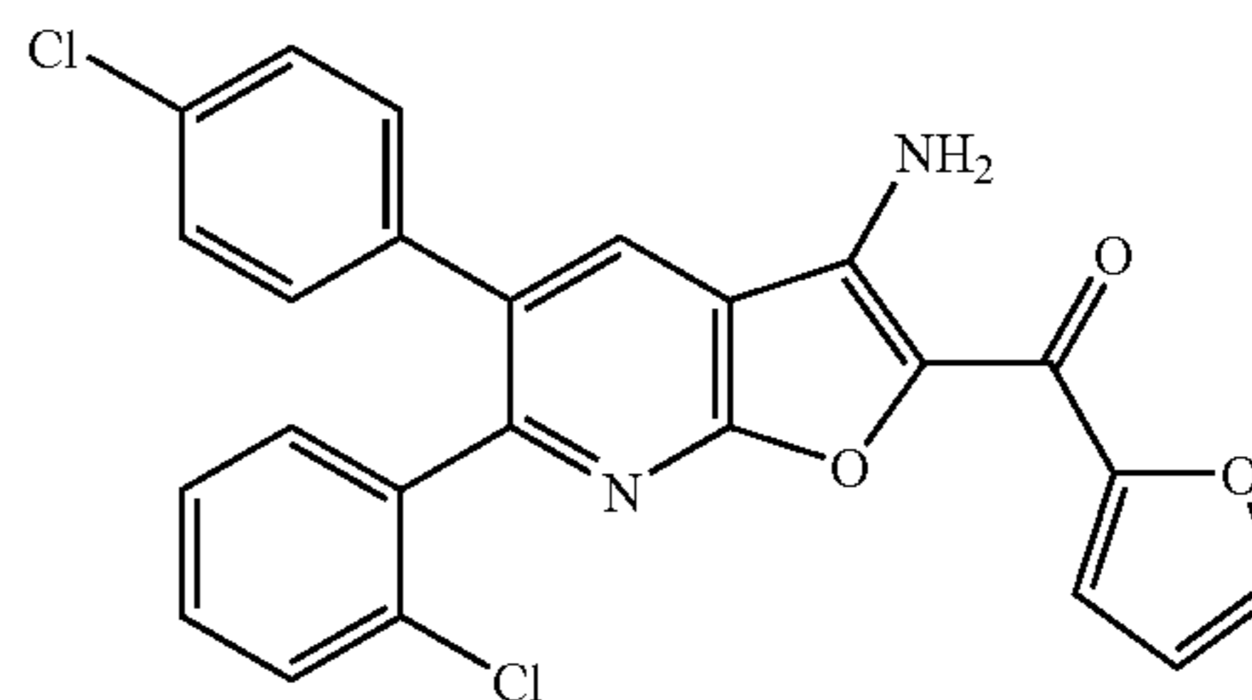
[3-amino-6-(2-chlorophenyl)-5-(4-chlorophenyl)furo[2,3-b]pyridin-2-yl](2-furyl)methanone
