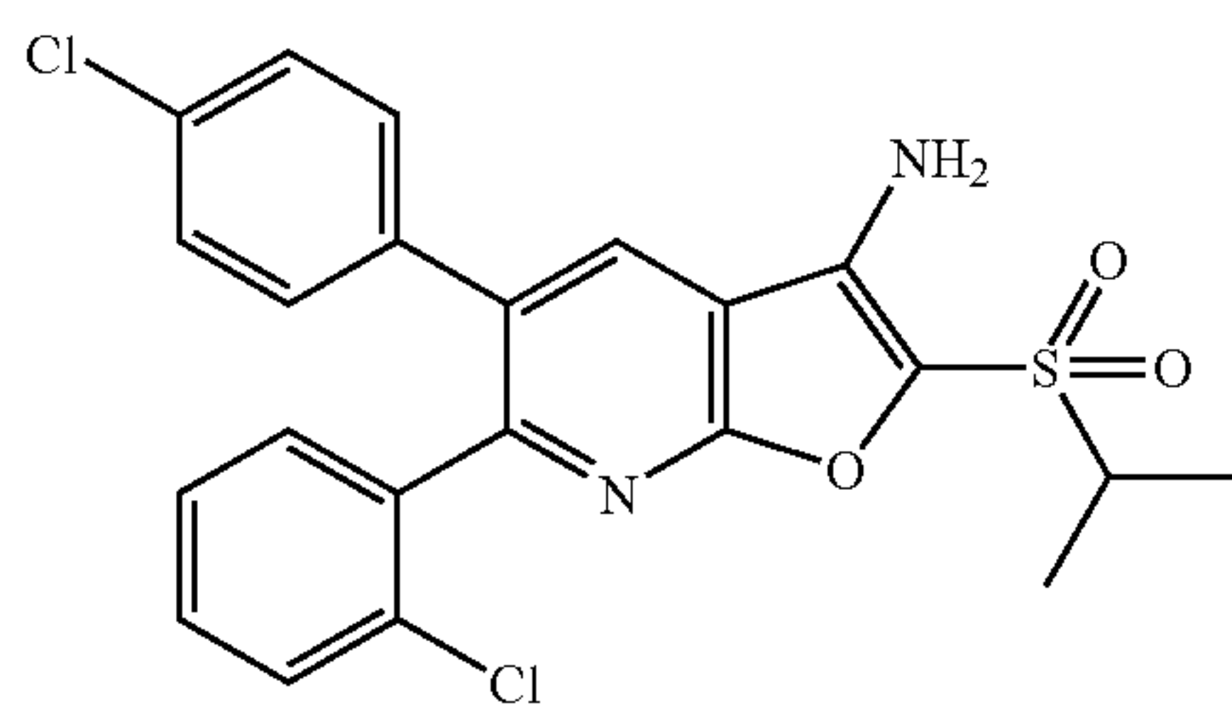
2-(Tert-butylsulfonyl)-6-(2-chlorophenyl)-5-(4-chlorophenyl)furo[2,3-b]pyridin-3-amine
