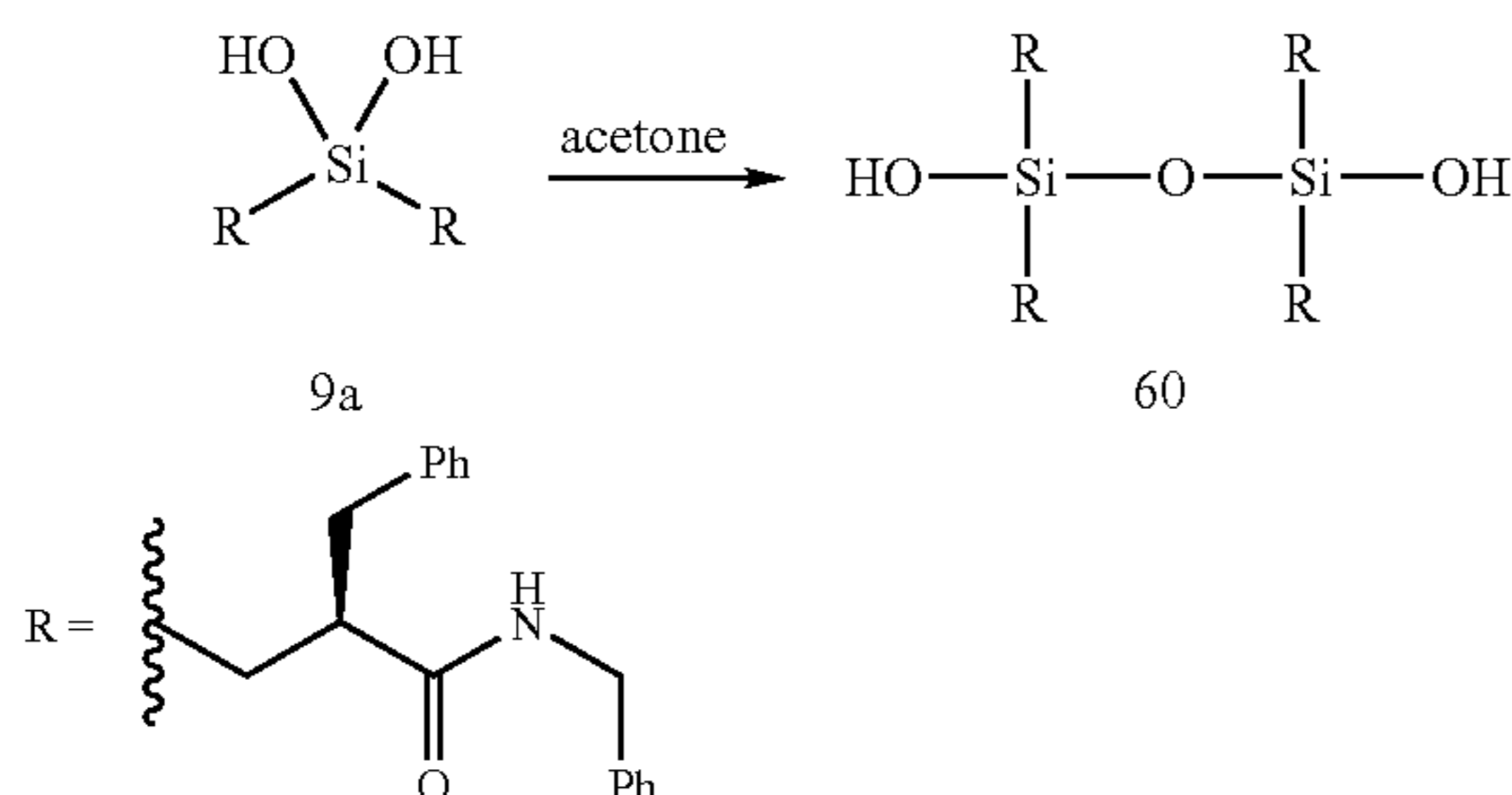
Silanediol Dimer (60)
