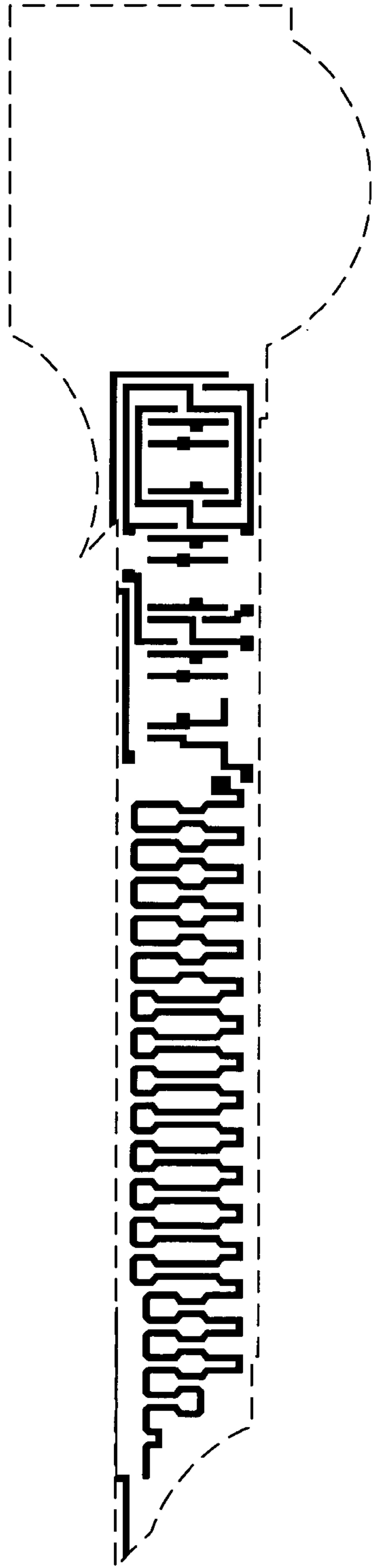
Poly mask
