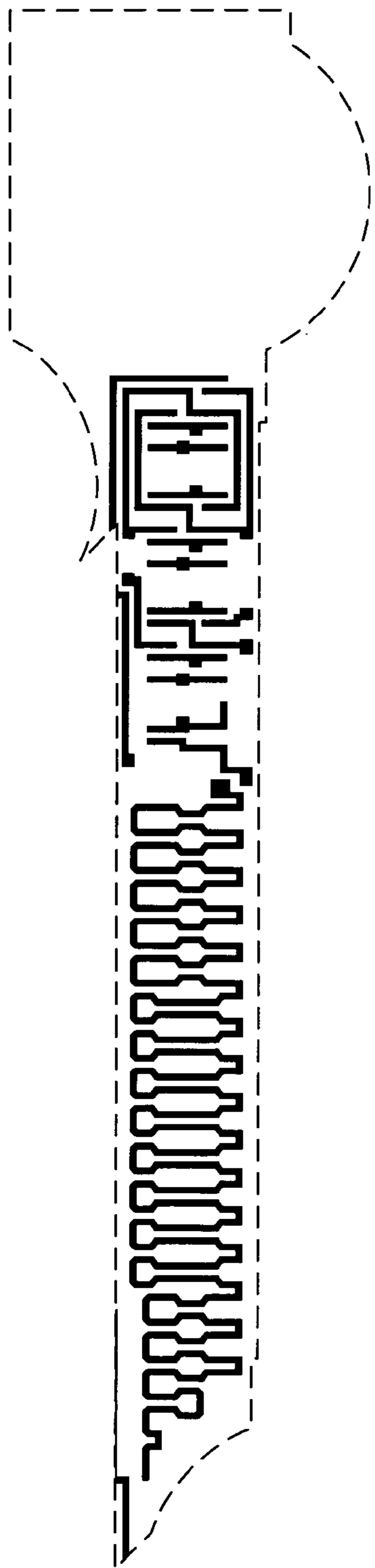
Poly mask
