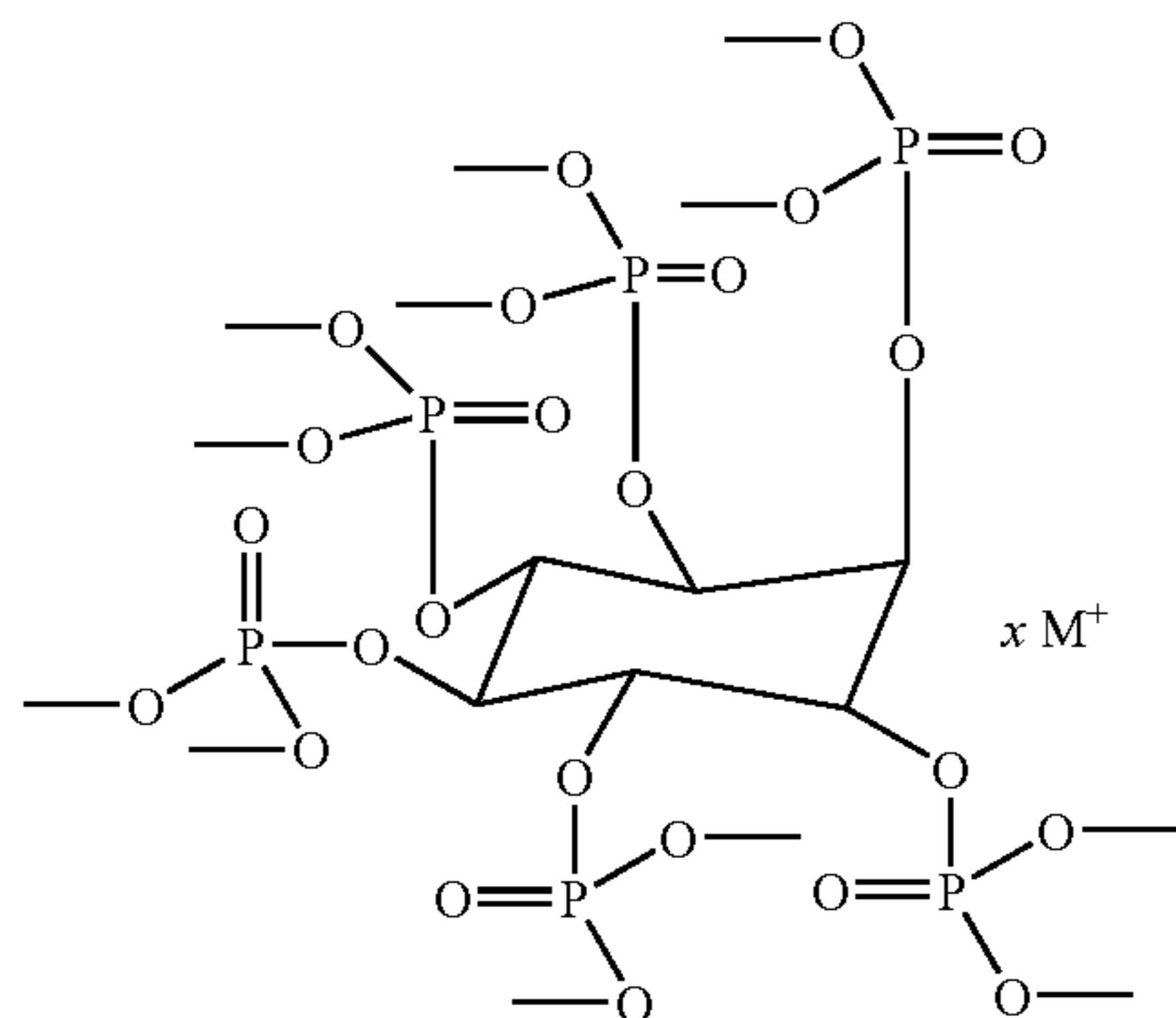
IV: IHP ammonium salt
