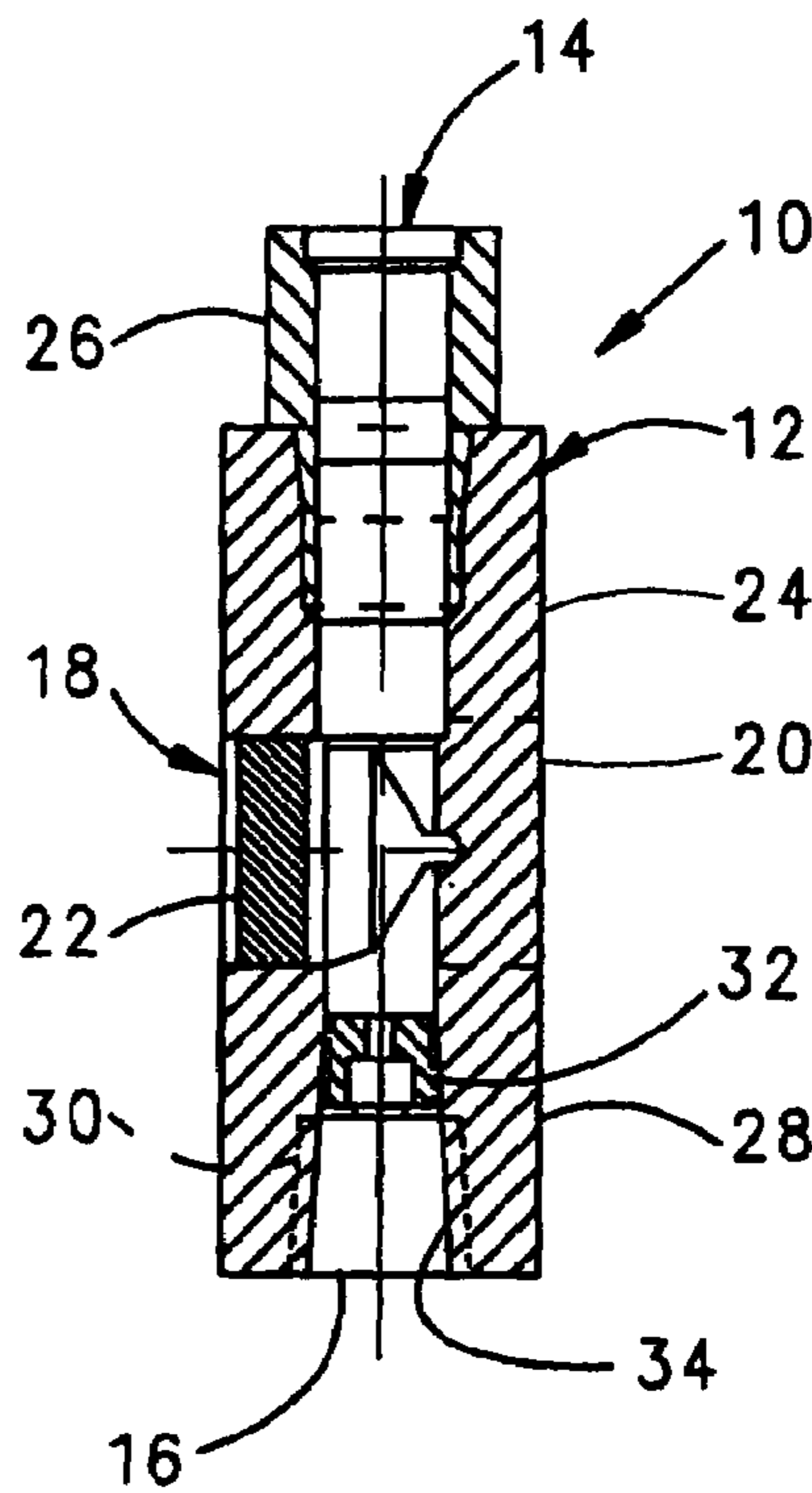
SECTION A-A
