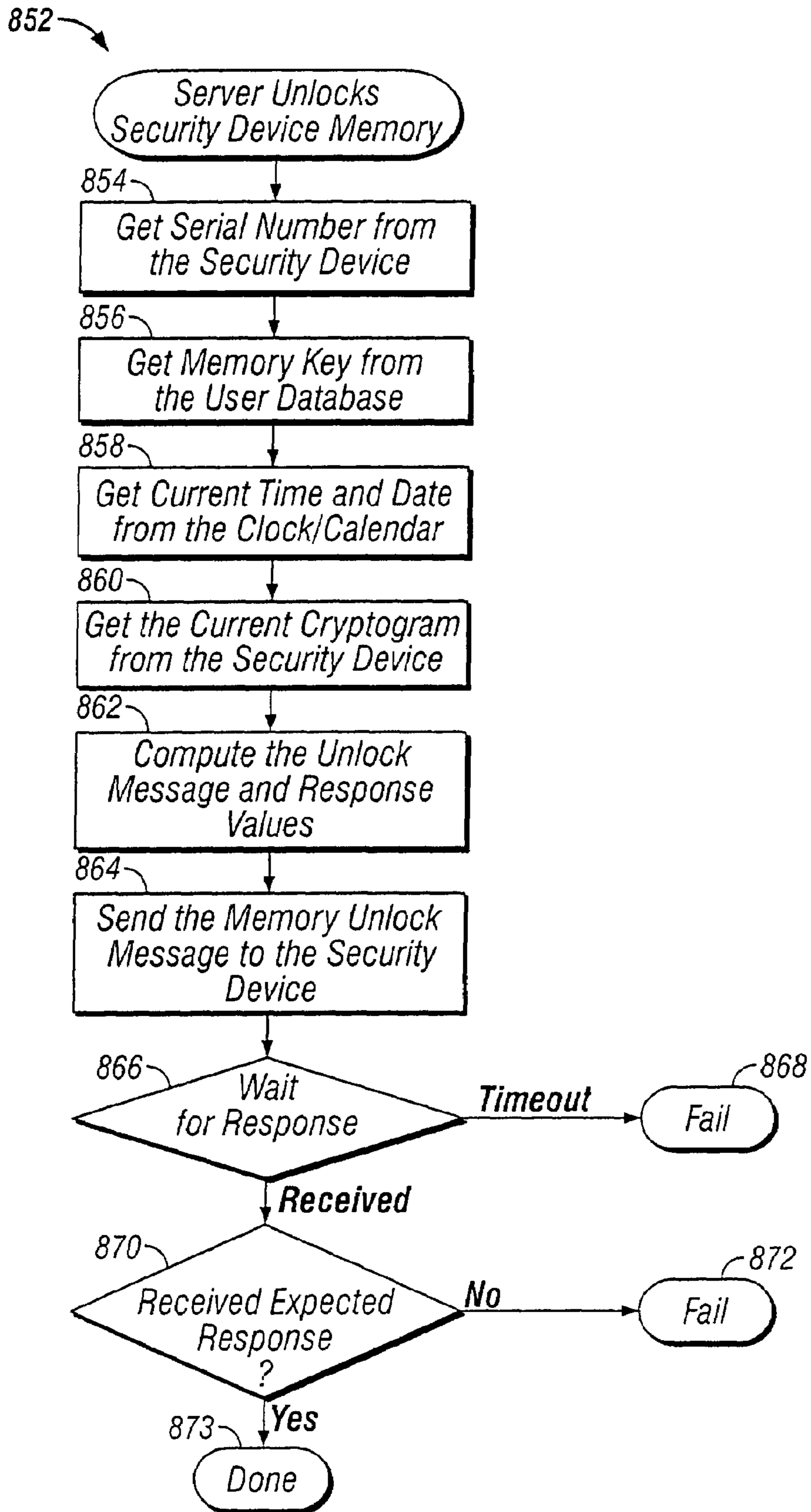
FIG. 8d
