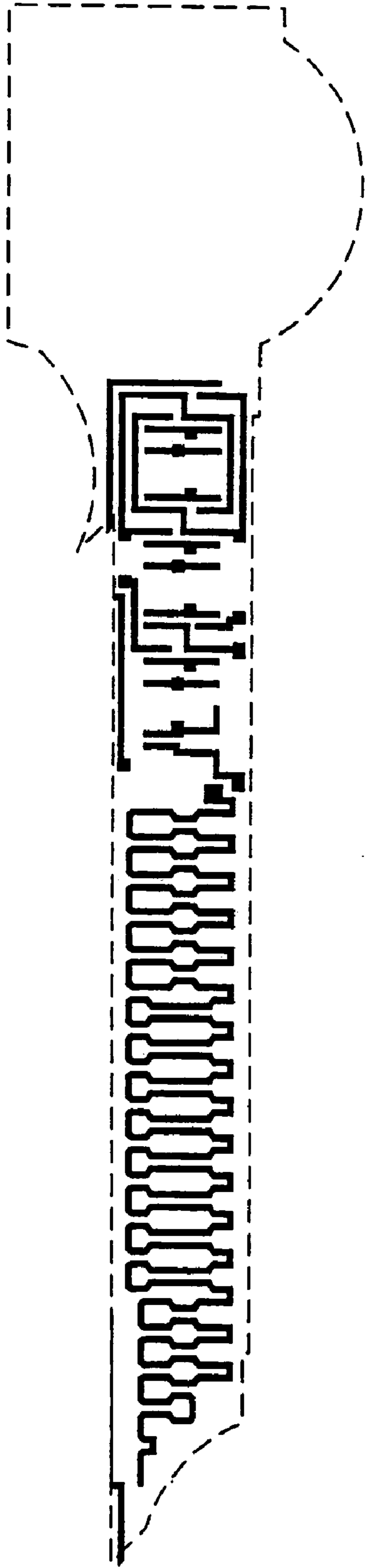
Poly mask
