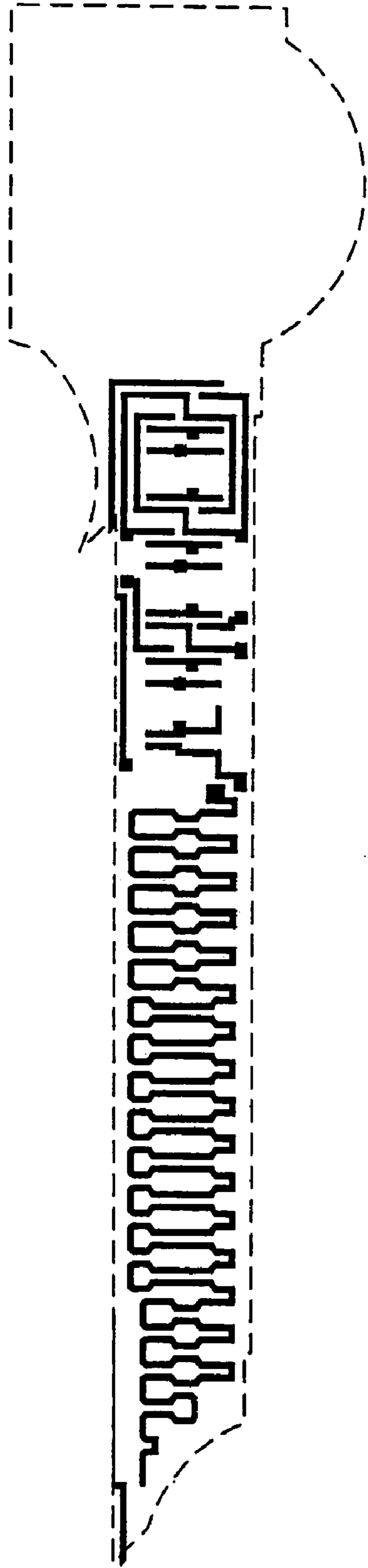
Poly mask
