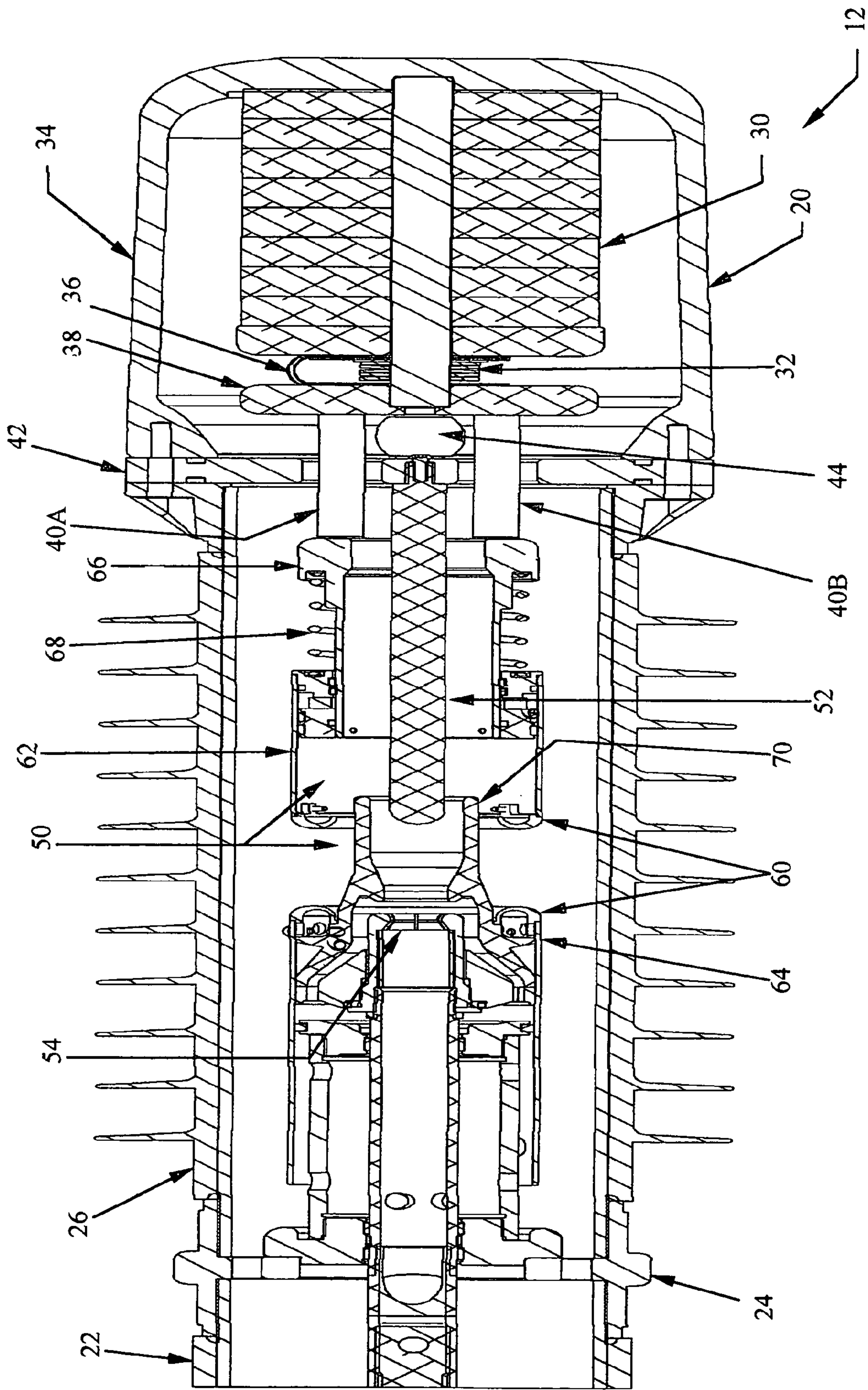
FIG. 5
