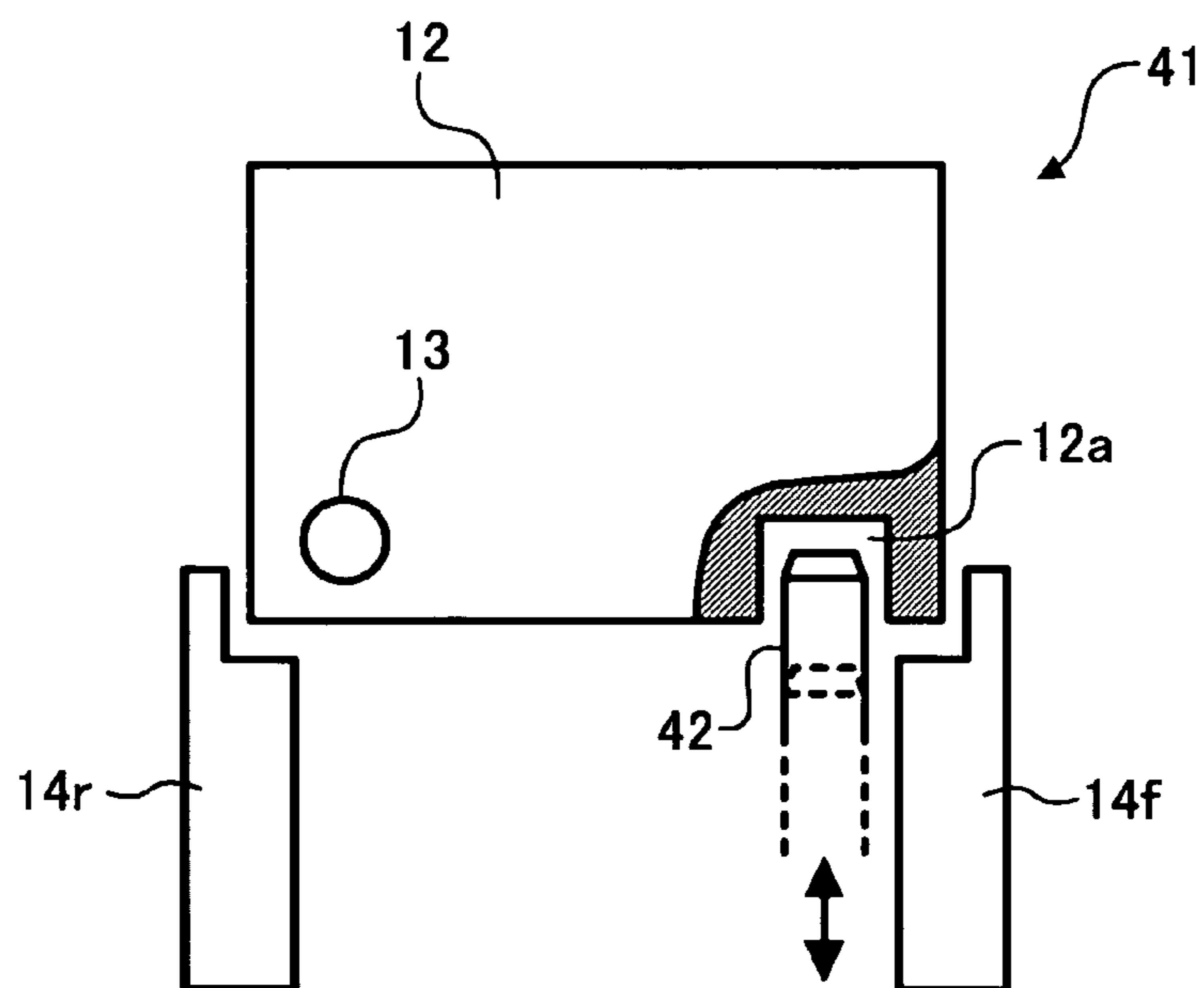
FIG. 6B
