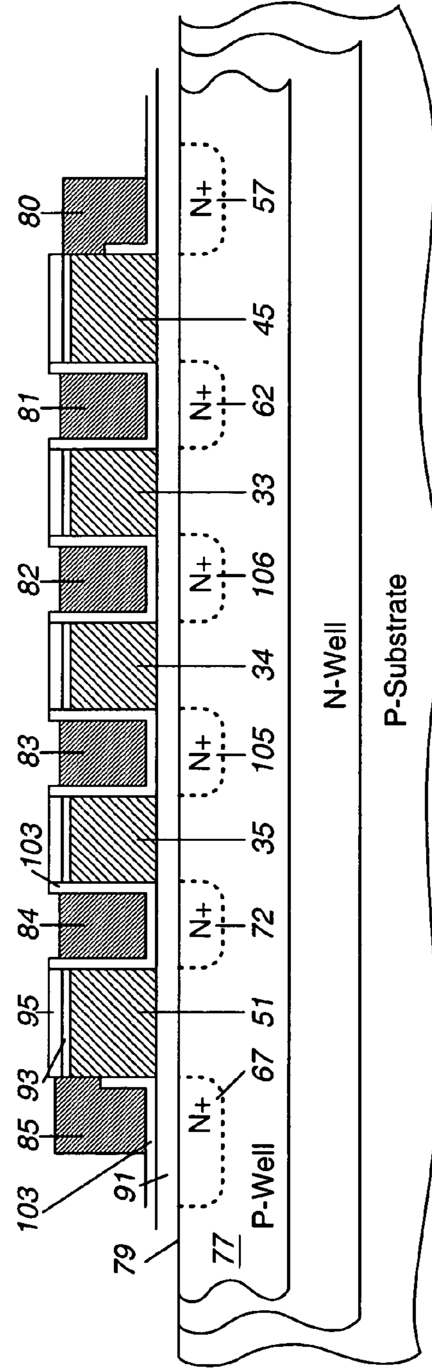
FIG. 4 (Section A-A)
