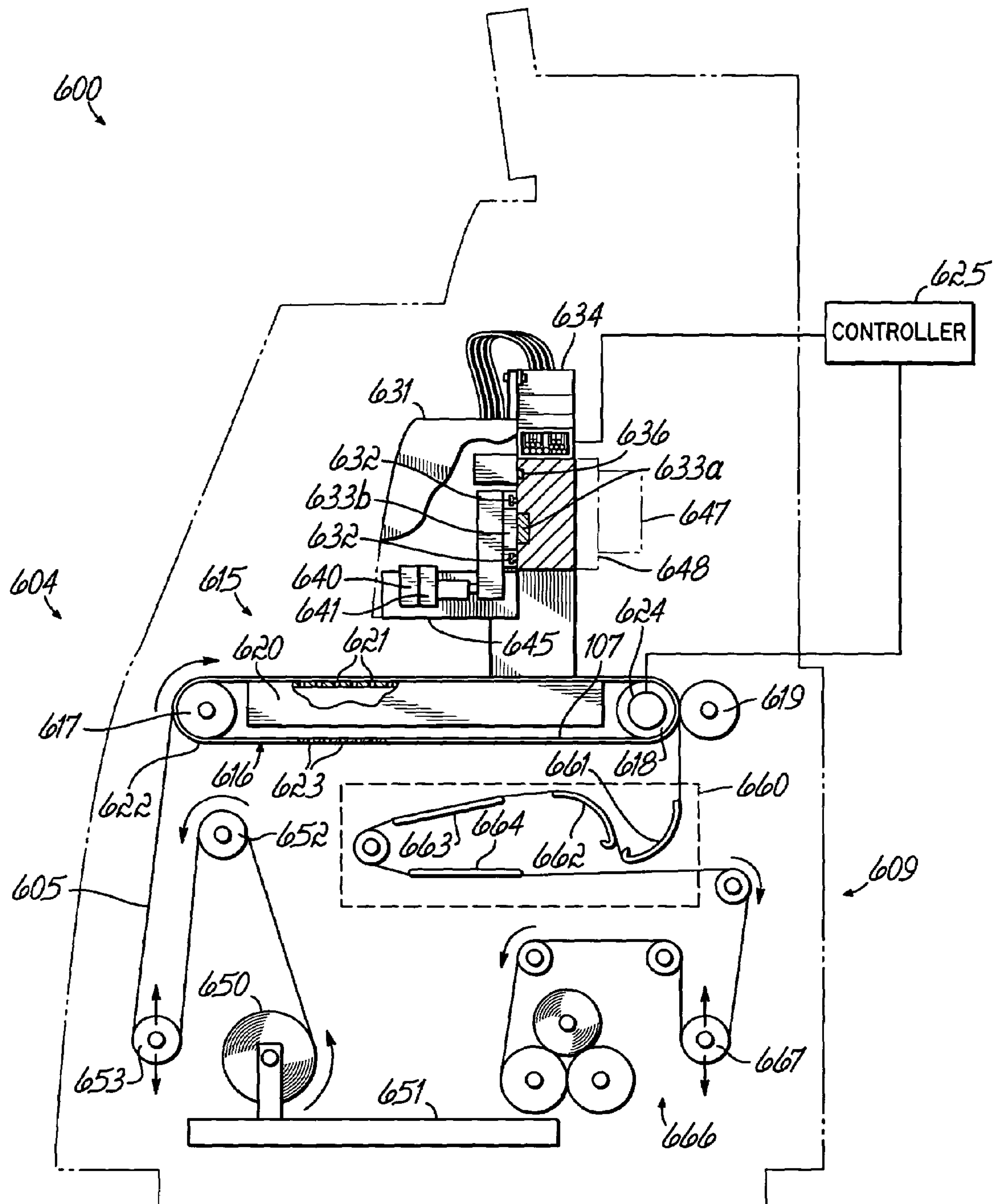
FIG. 3
