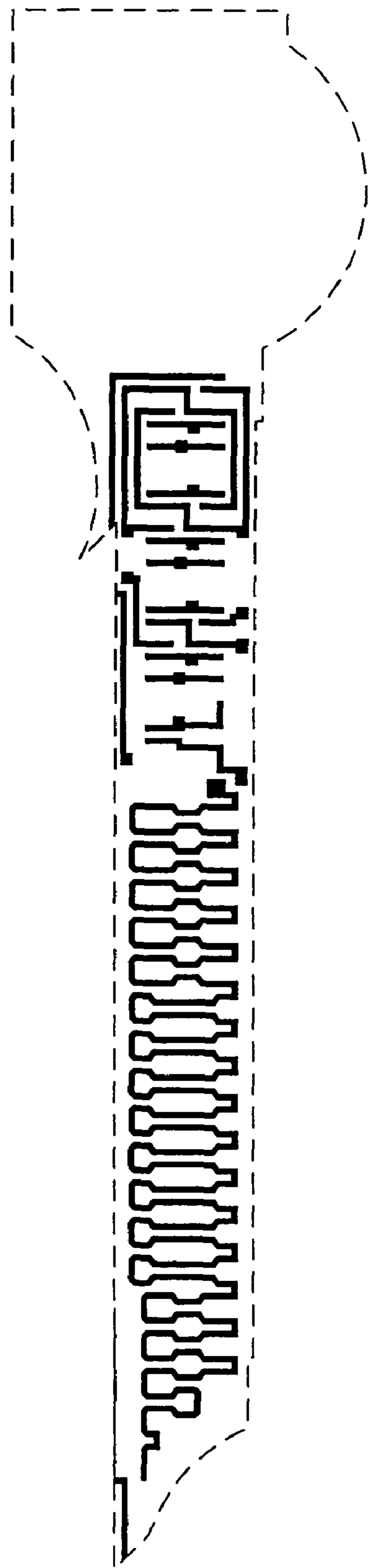
Poly mask
