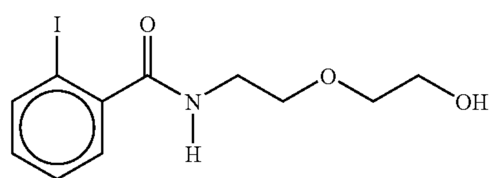
2-[N-(2-iodobenzoyl)aminoethoxy]ethanol
