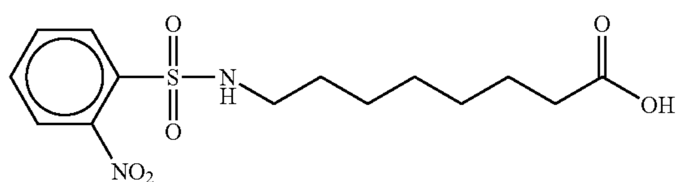
8-(2-nitrobenzenesulfonyl)aminocaprylic acid
