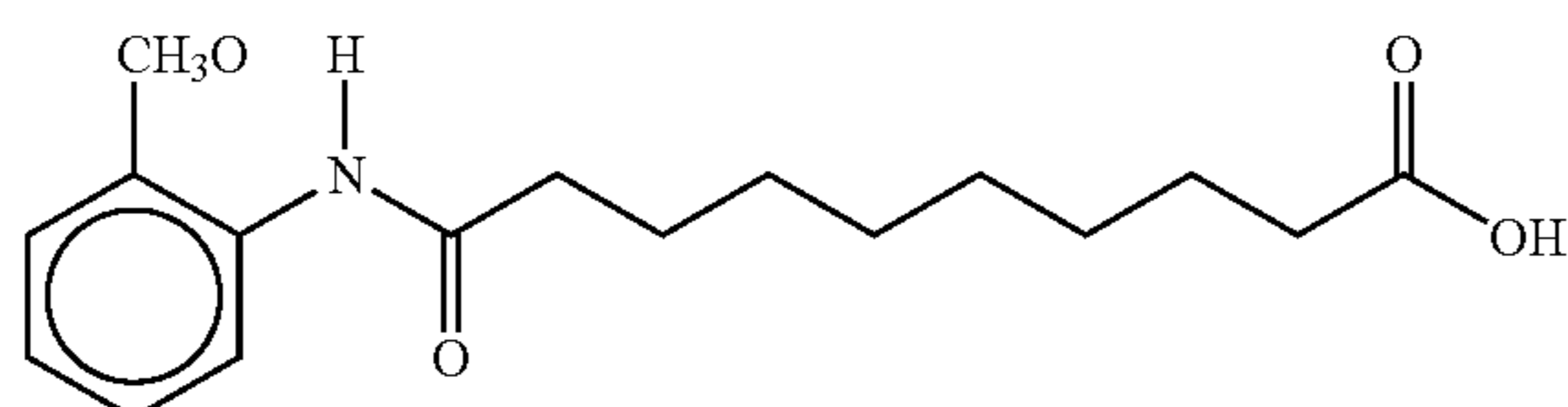
10-(N-2-Methoxyanilino)sebacic acid
