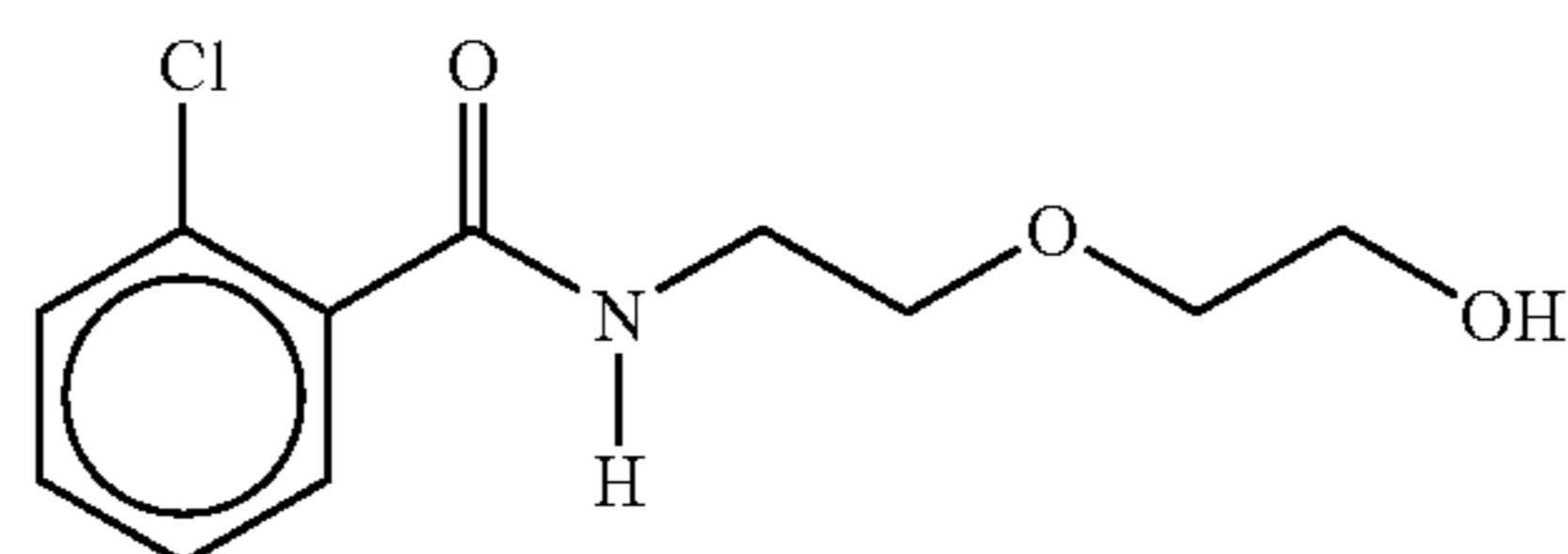
2-[2-N-(2-chlorobenzoyl)aminoethoxy]ethanol
