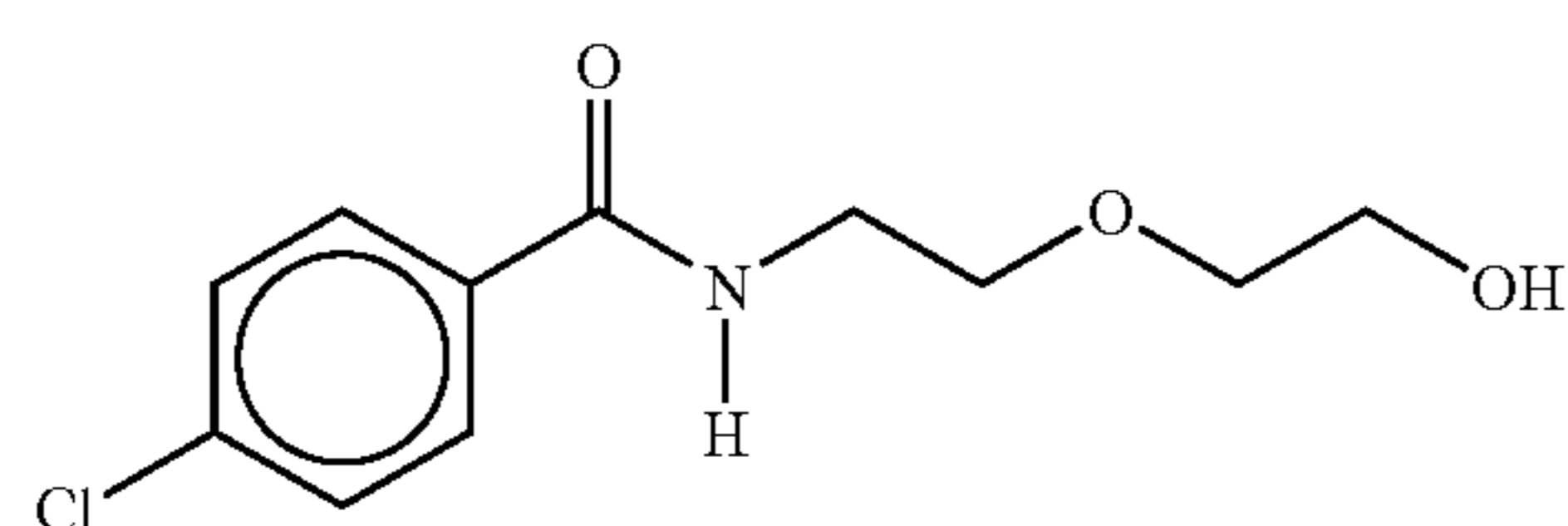
2-[2-N-(4-chlorobenzoyl)aminoethoxy]ethanol
