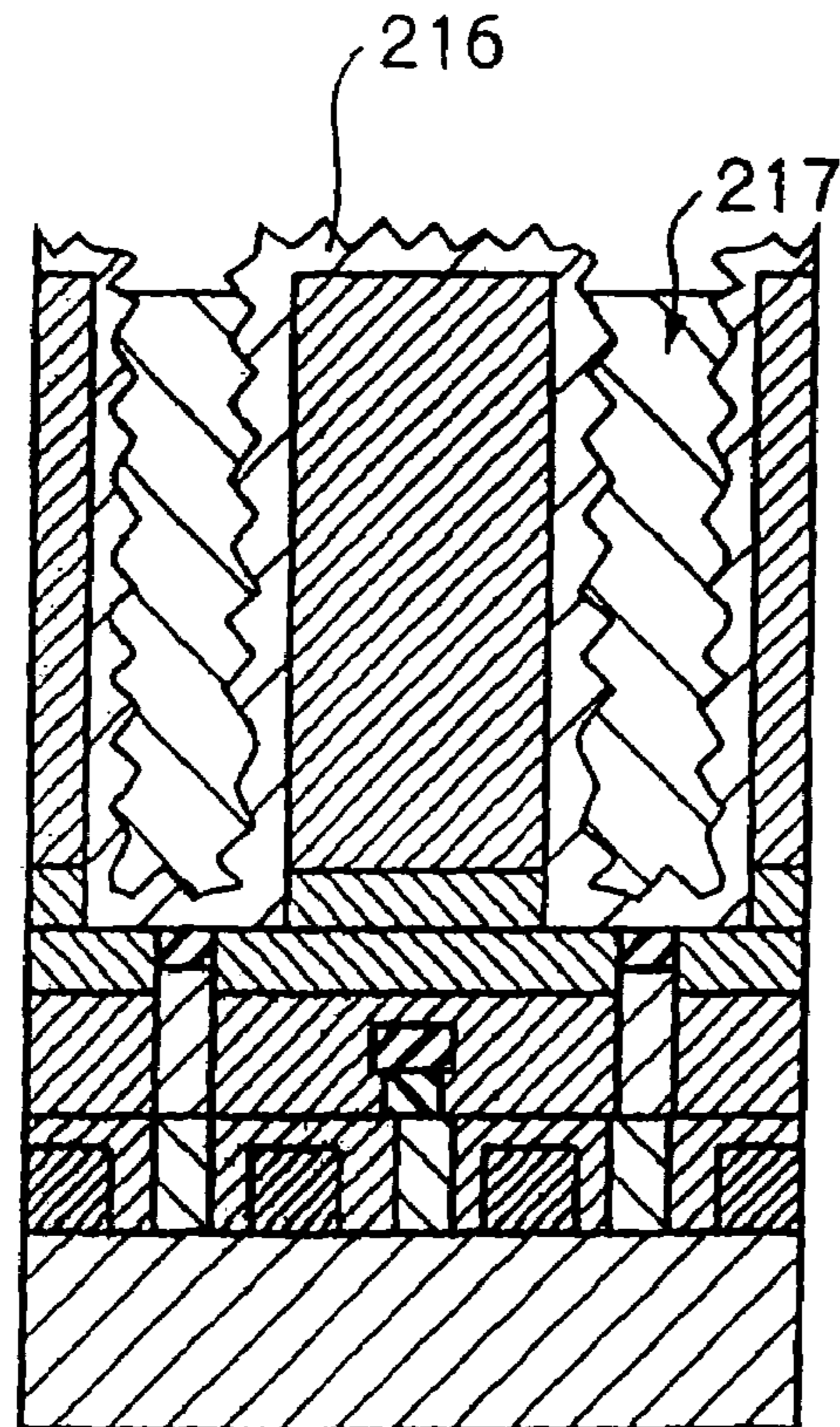
FIG. 2E (PRIOR ART)
