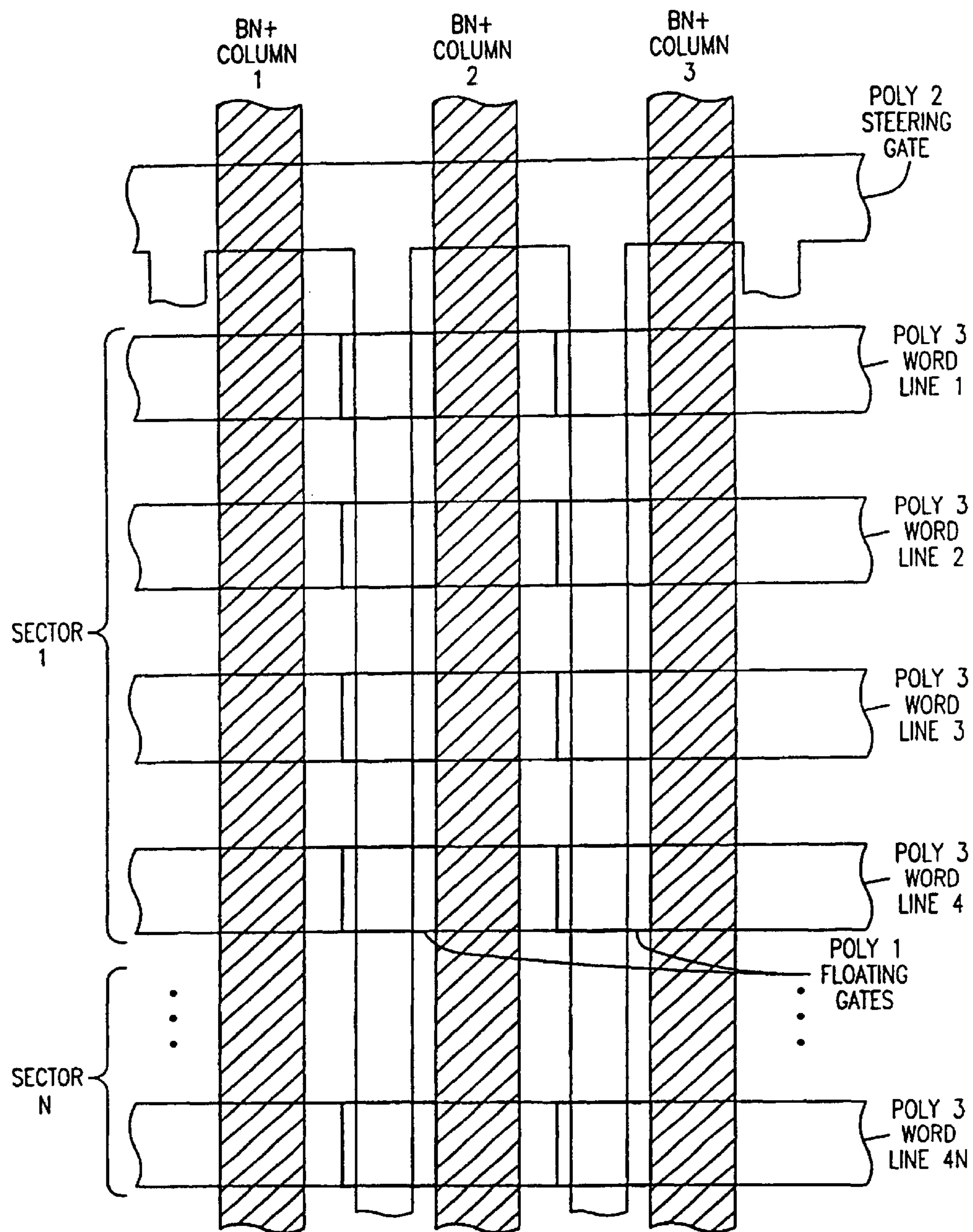
FIG. 1G
