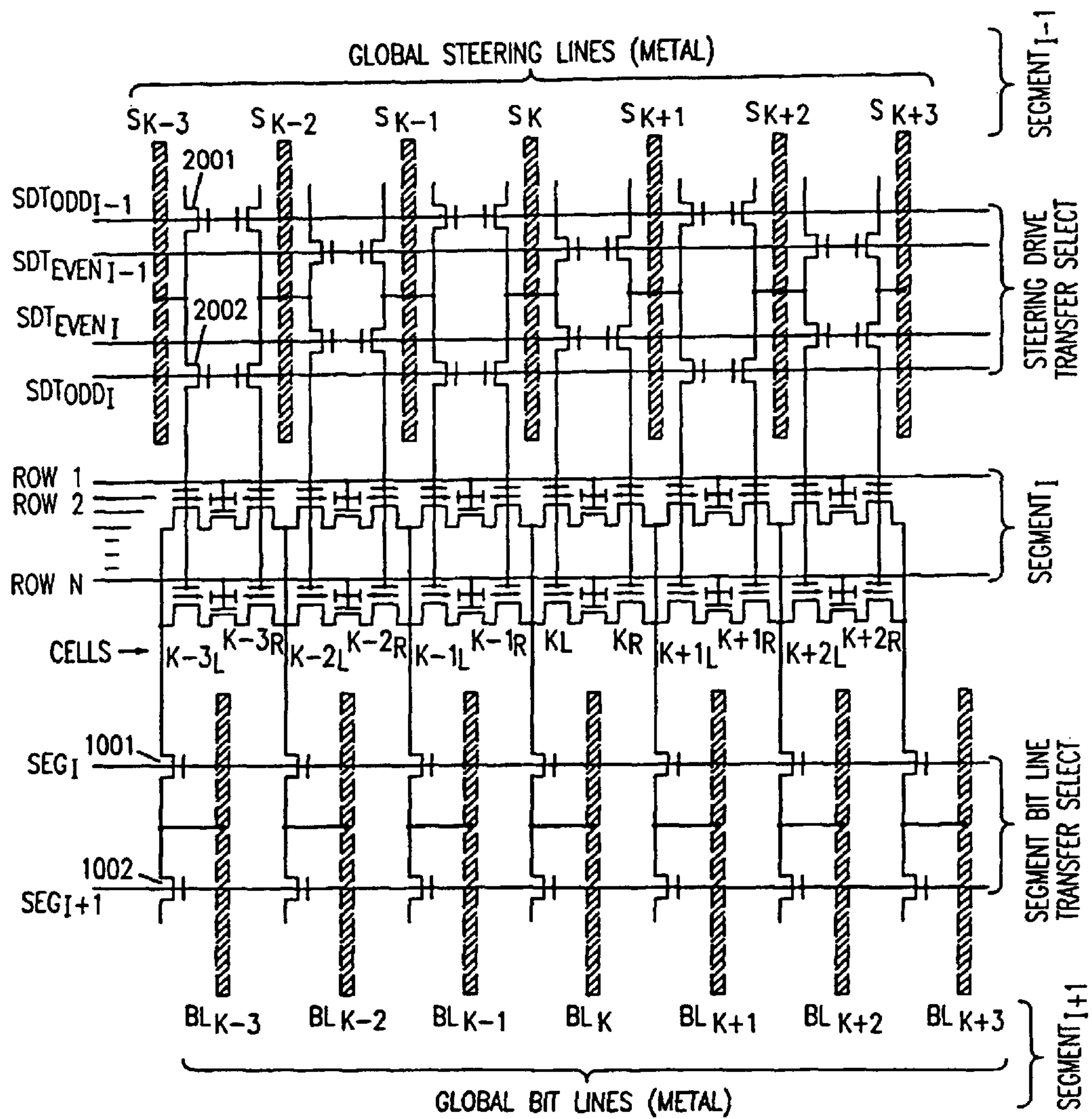
FIG. 10C
