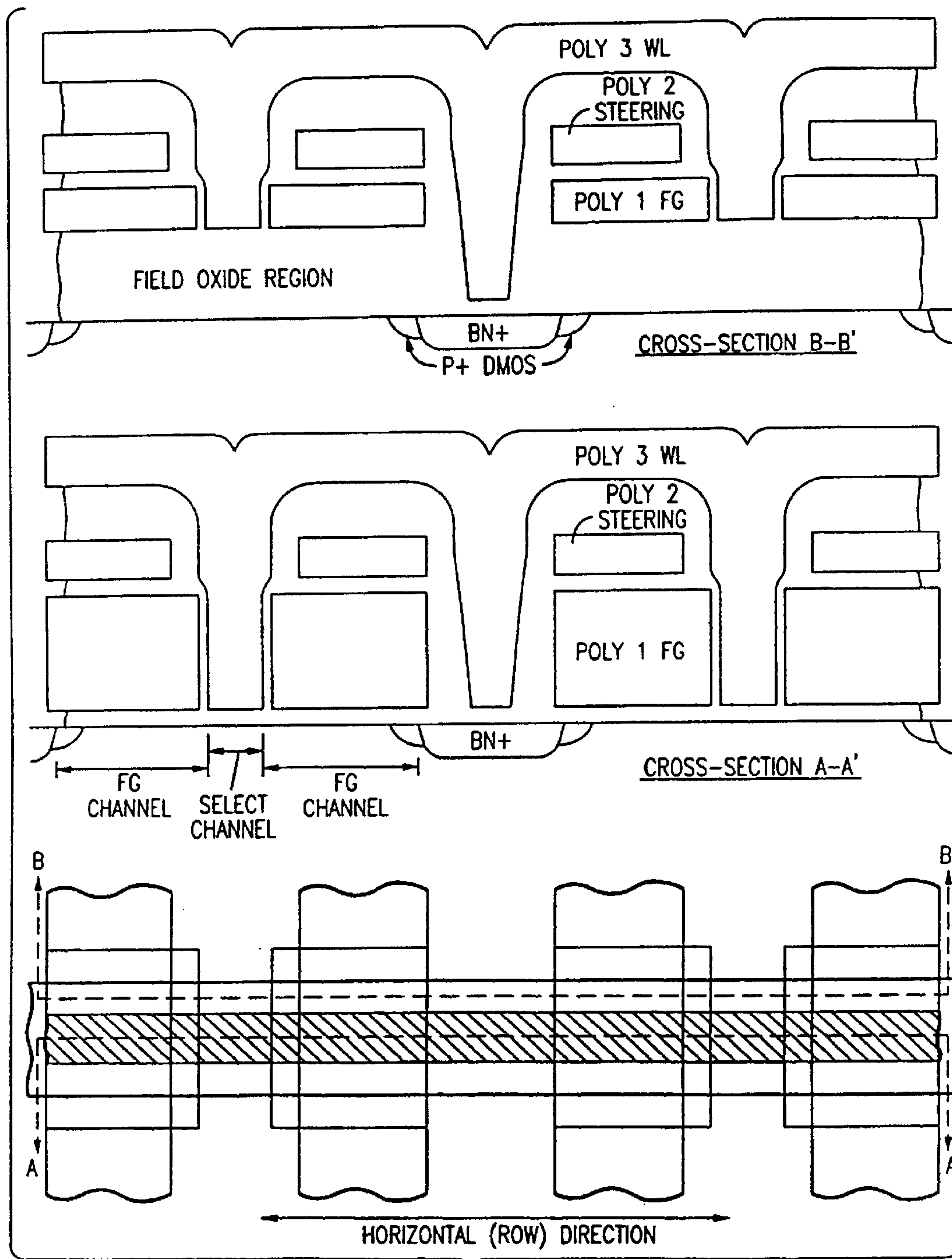
FIG. 11E
