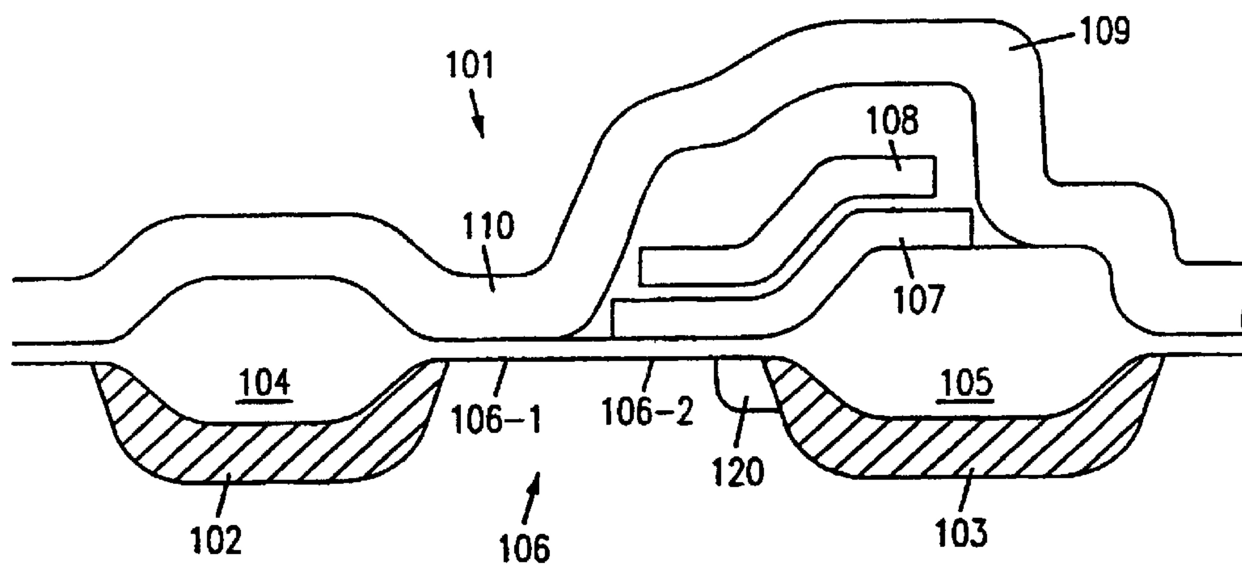
FIG. 1B
