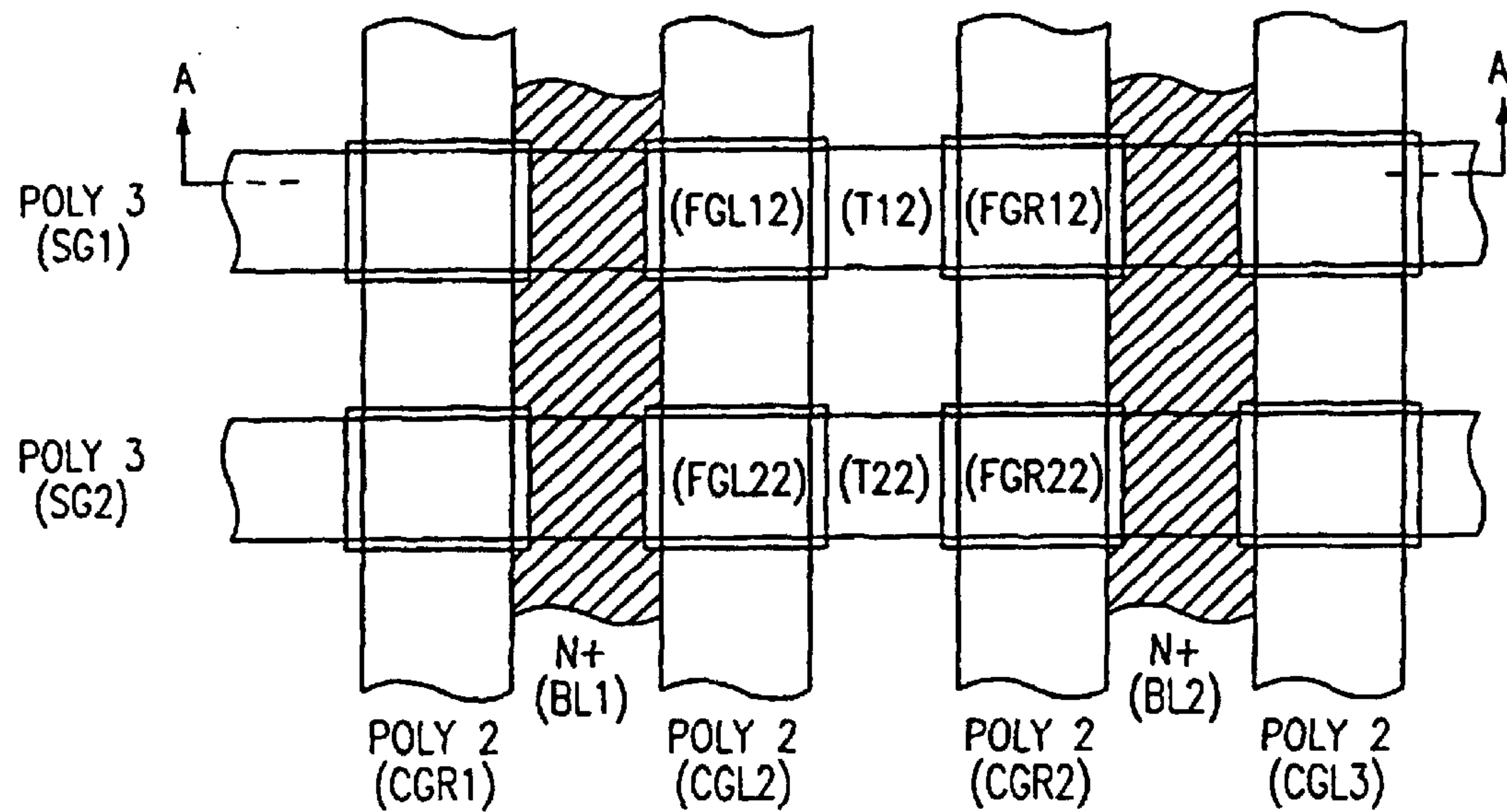
FIG. 9A
