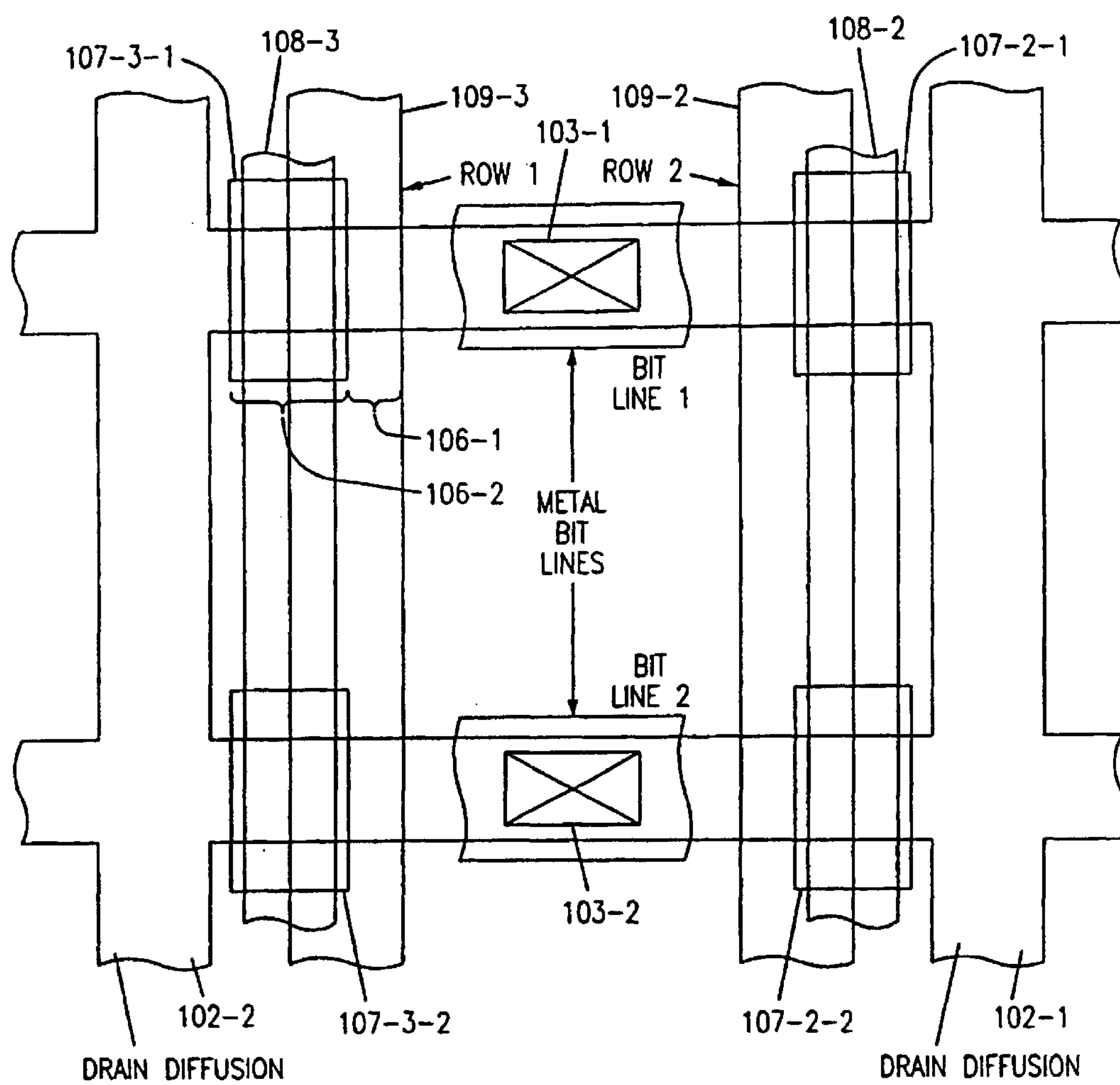
FIG. 2B
